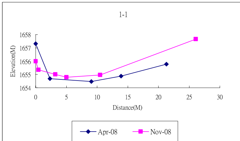
圖 2-7 南湖溪中游斷面 1-1 剖面高程圖
