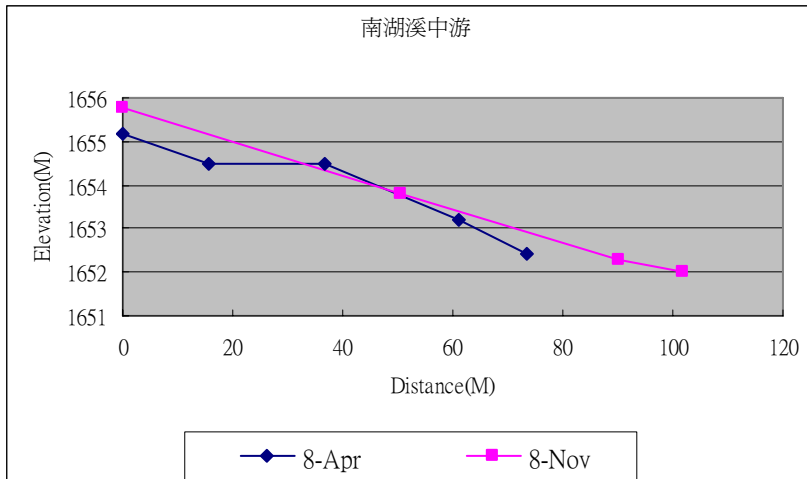
圖 2-6 南湖溪中游斷面高程剖面圖
