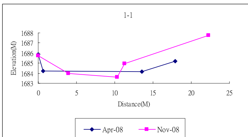
圖 2-5 南湖溪上游斷面 1-1 剖面高程圖
