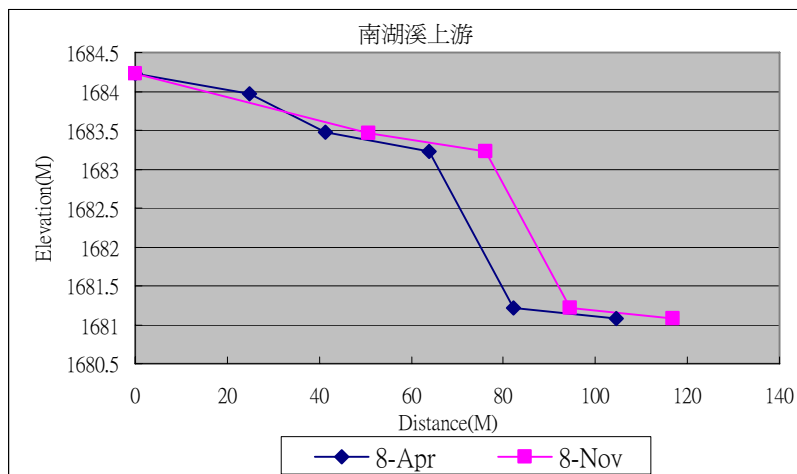
圖 2-4 南湖溪上游斷面高程剖面圖
