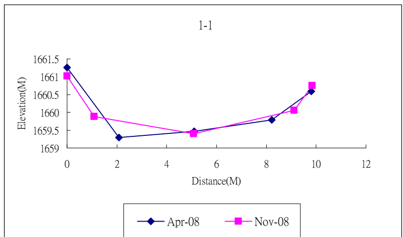
圖 2-11 耳無溪断面 1-1 剖面高程圖
