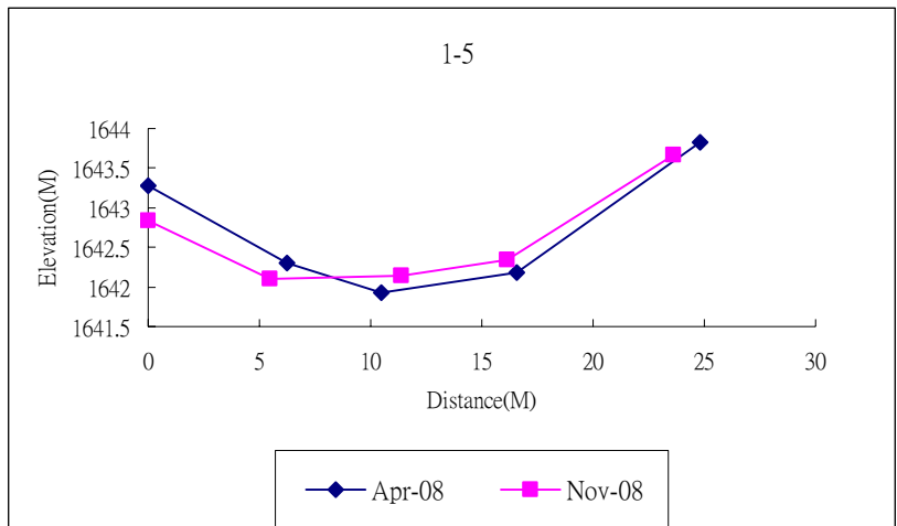
圖 2-9 南湖溪下游断面 1-5 剖面高程圖
