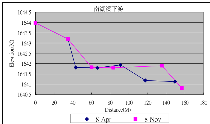
圖 2-8 南湖溪下游斷面高程剖面圖
