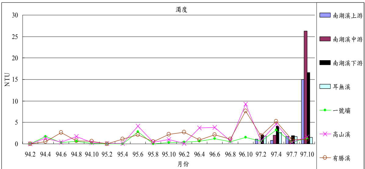
圖 1-8 歷年七家灣溪與南湖溪 2、4、6、7、8、10 月濁度之變化
