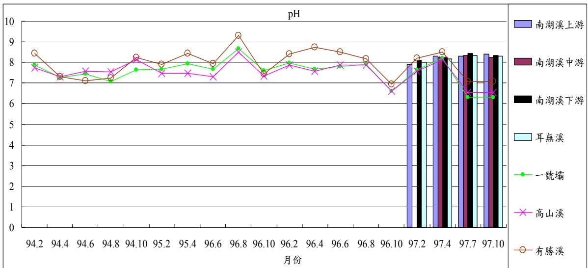
圖 1-4 歷年七家灣溪與南湖溪 2、4、6、7、8、10 月 pH 值之變化
