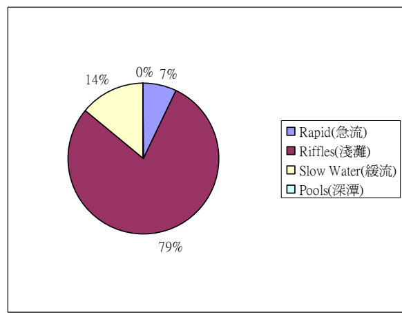
圖 2-15 南湖溪中游棲地環境類型分布 (2008/04)
