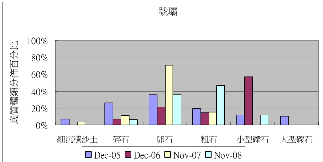
圖 2-29 一號壩 11 月份底質分佈類型百分比圖
