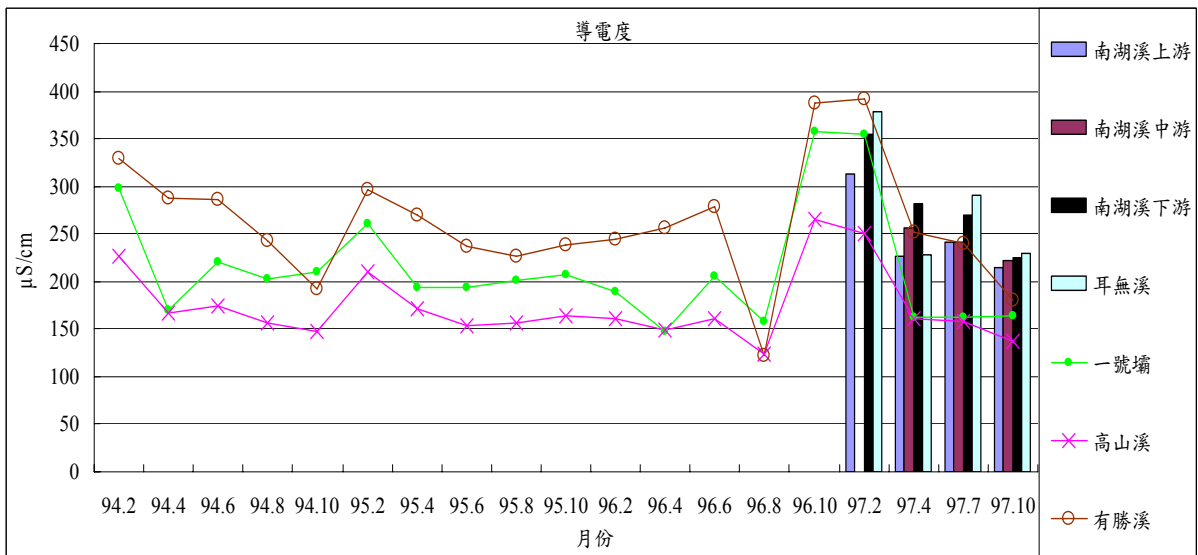
圖 1-6 歷年七家灣溪與南湖溪 2、4、6、7、8、10 月導電度之變化
