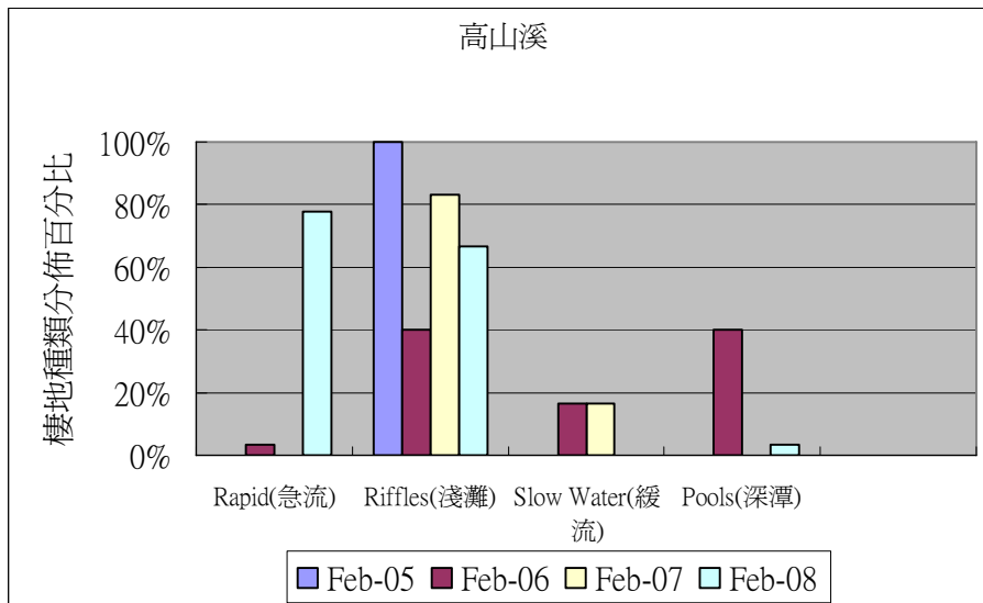
圖 2-30 高山溪 2 月份棲地分佈類型百分比圖
