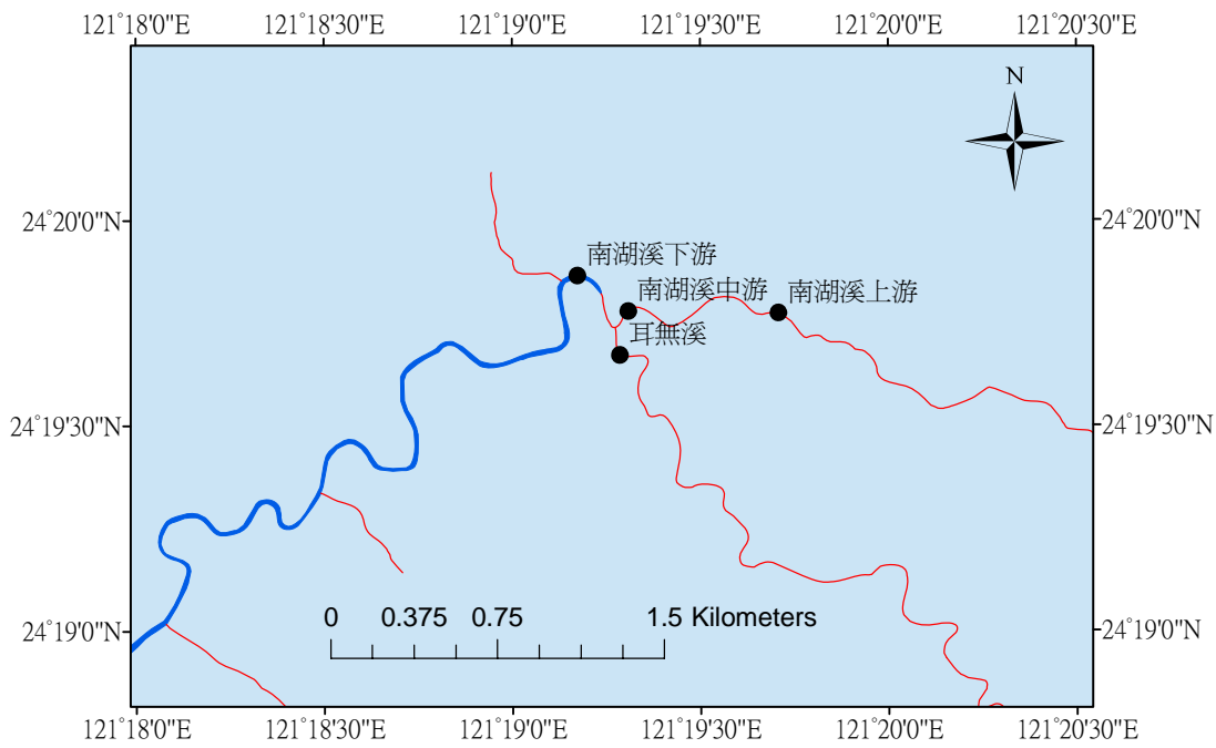
圖 3-1、南湖溪之水棲昆蟲監測調查採樣站之相關位置圖
