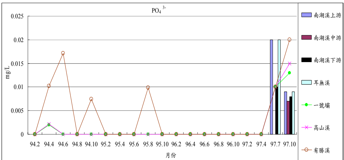
圖 1-16 歷年七家灣溪與南湖溪 2、4、6、7、8、10 月 PO 4 3- 值變化
