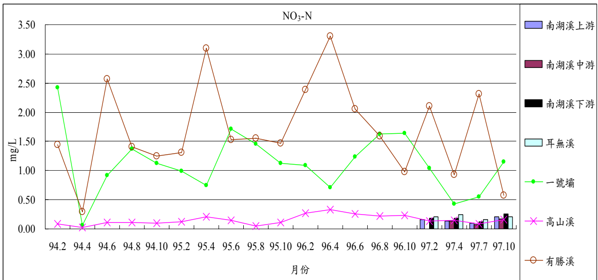
圖 1-11 歷年七家灣溪與南湖溪 2、4、6、7、8、10 月 NO 3 -N 之變化
