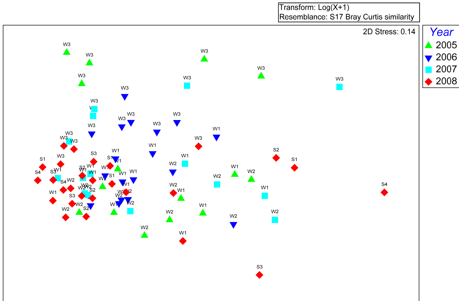
圖 3-5、南湖溪採樣站與武陵地區溪流 3 測站水生昆蟲之 MDS 分析。(圖標數字前二碼表示樣站編號，W1 為一號壩、W2 為高山溪、W3 為有勝溪、S1 為南湖溪下游、S2 為耳無溪、S3 為南湖溪上游及 S4 為南湖溪中游)
