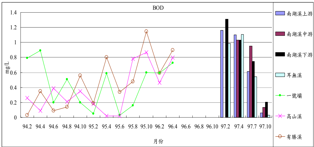
圖 1-9 歷年七家灣溪與南湖溪 2、4、6、7、8、10 月 BOD 值之變化
