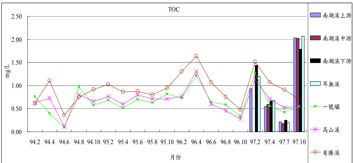
圖1-18 歷年七家灣溪與南湖溪2、4、6、7、8、10月TOC之變化
