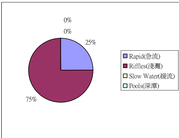
圖 2-14 南湖溪中游棲地環境類型分布 (2008/11)
