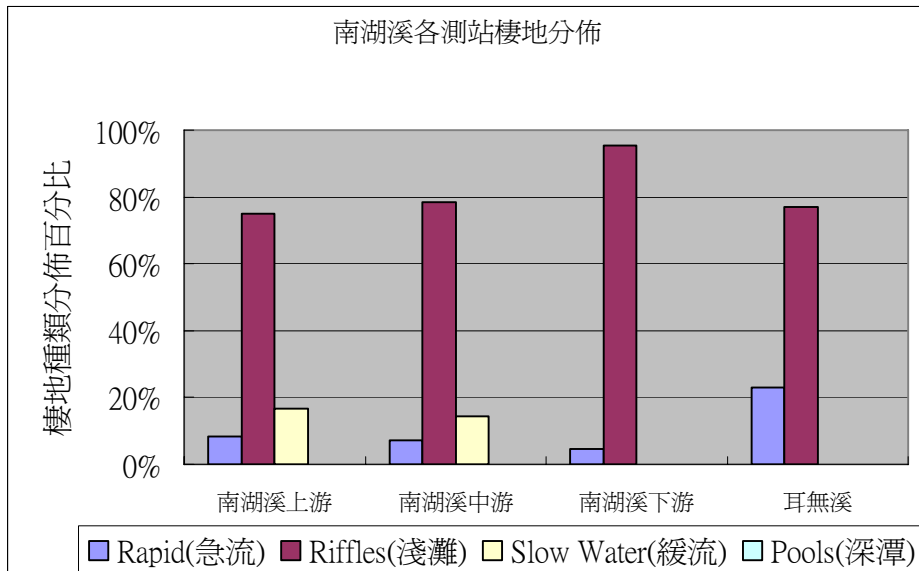
圖 2-20 南湖溪 4 月份各測站棲地分佈類型百分比圖
