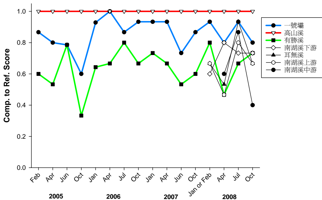
圖 3-4、南湖溪採樣站與武陵地區溪流 3 測站水生昆蟲之 RBPII 相對分數。
