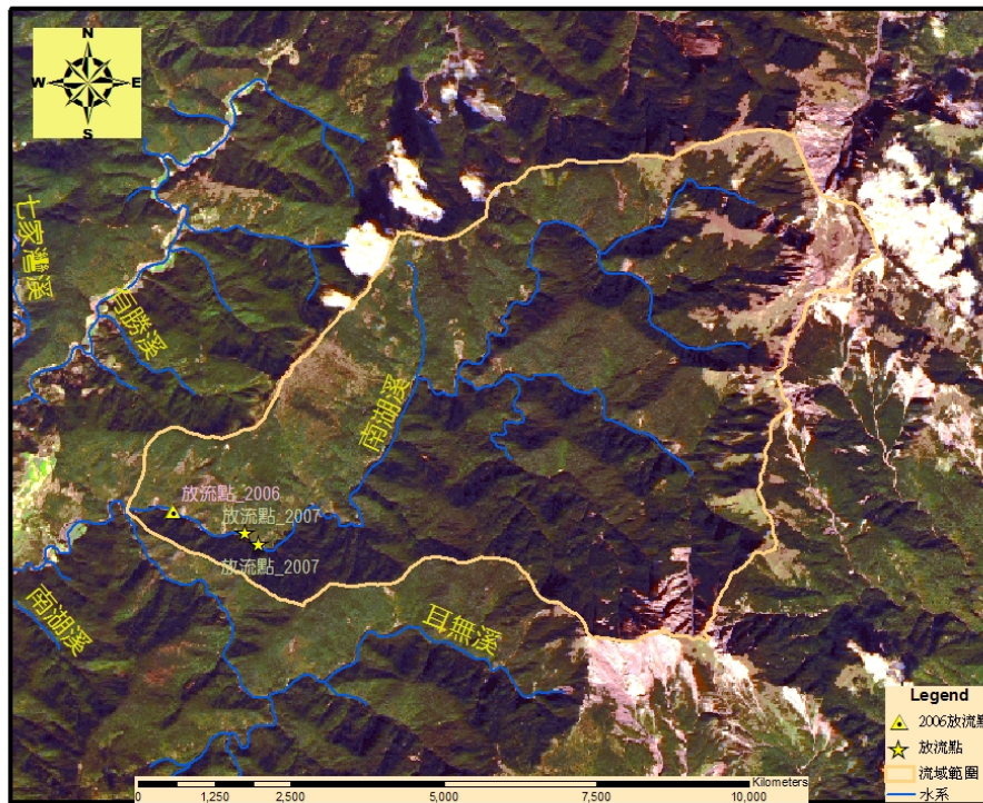
圖 2-1 南湖溪之櫻花鉤吻鮭放流點
