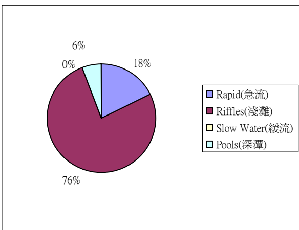
圖 2-16 南湖溪下游棲地環境類型分布 (2008/11)
