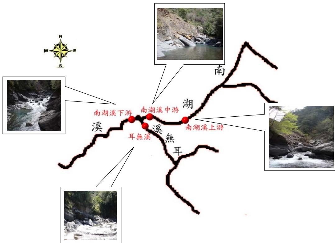
圖 1-2 南湖溪各測站位置圖
