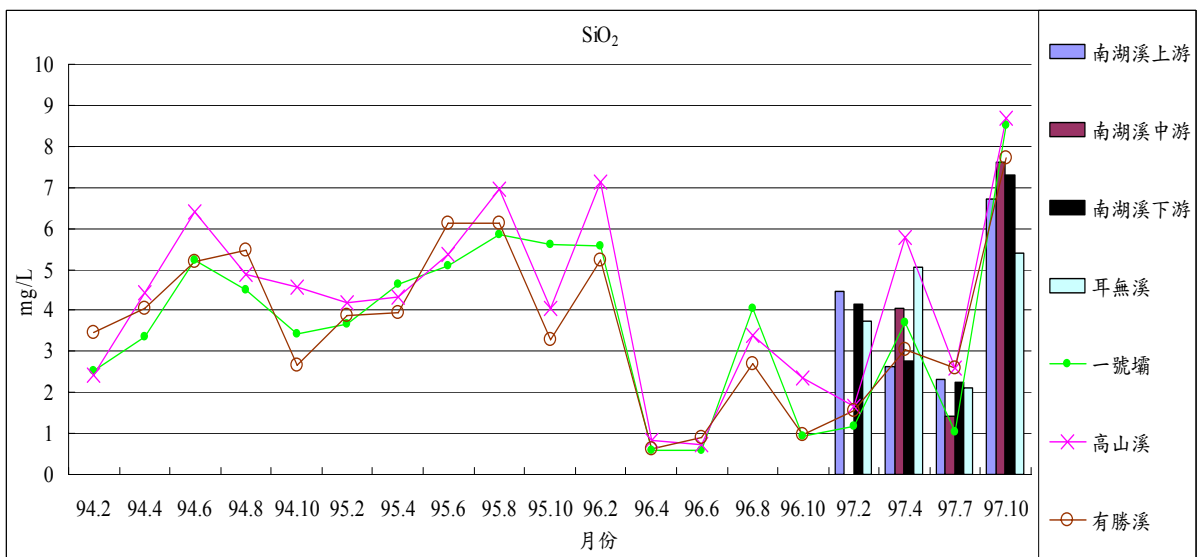
圖 1-10 歷年七家灣溪與南湖溪 2、4、6、7、8、10 月 SiO 2 之變化
