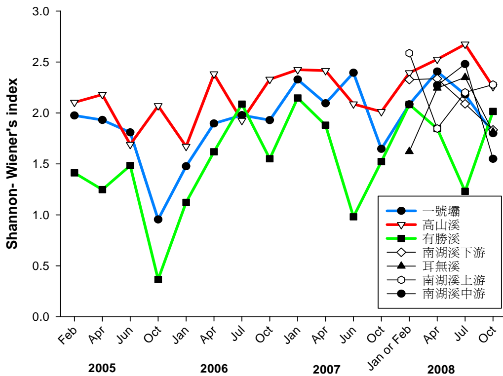
圖 3-3、南湖溪採樣站與武陵地區溪流 3 測站水生昆蟲之 Shannon- Wiener's index。
