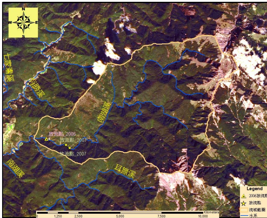
圖 1-1 南湖溪流域及歷年櫻花鉤吻鮭放流點空照圖
