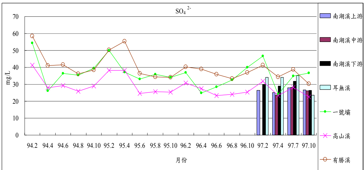
圖 1-14 歷年七家灣溪與南湖溪 2、4、6、7、8、10 月 SO 4 2- 之變化
