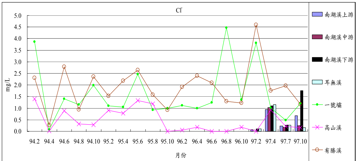
圖 1-15 歷年七家灣溪與南湖溪 2、4、6、7、8、10 月 CI 值變化
