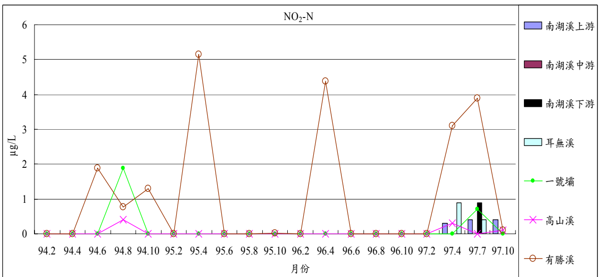
圖 1-12 歷年七家灣溪與南湖溪 2、4、6、7、8、10 月 NO 2 -N 之變化
