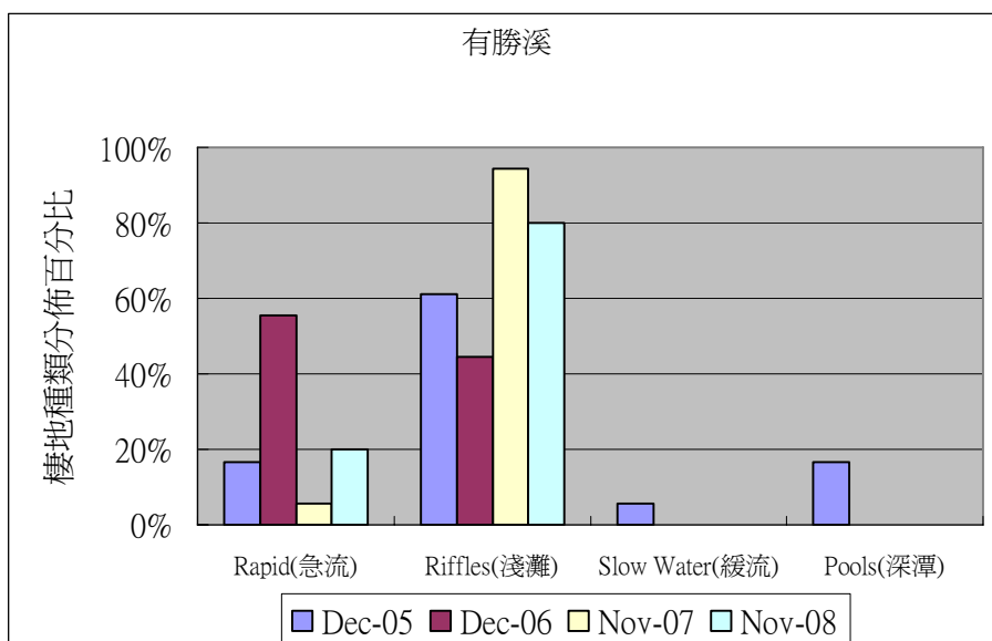
圖 2-23 有勝溪棲地歷年 11 月份分佈類型百分比圖
