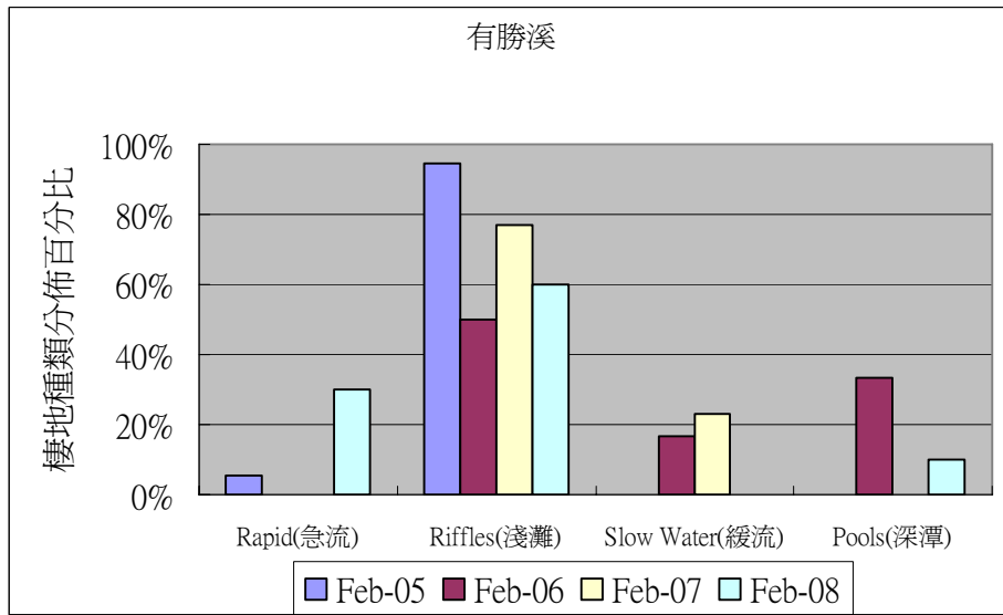
圖 2-22 有勝溪棲地歷年 2 月份分佈類型百分比圖
