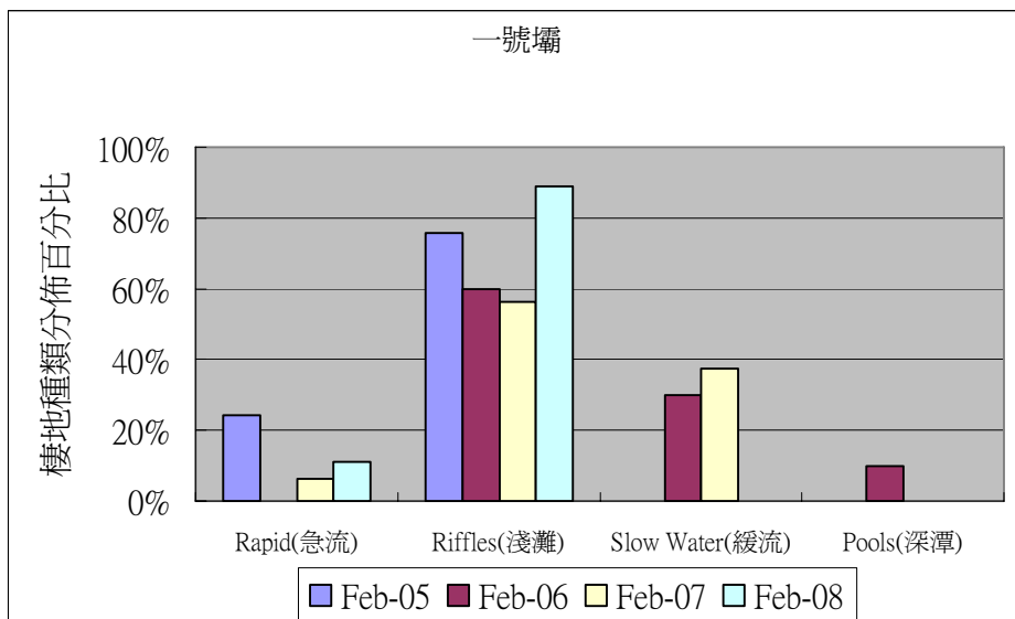
圖 2-26 一號壩歷年 2 月份棲地分佈類型百分比圖
