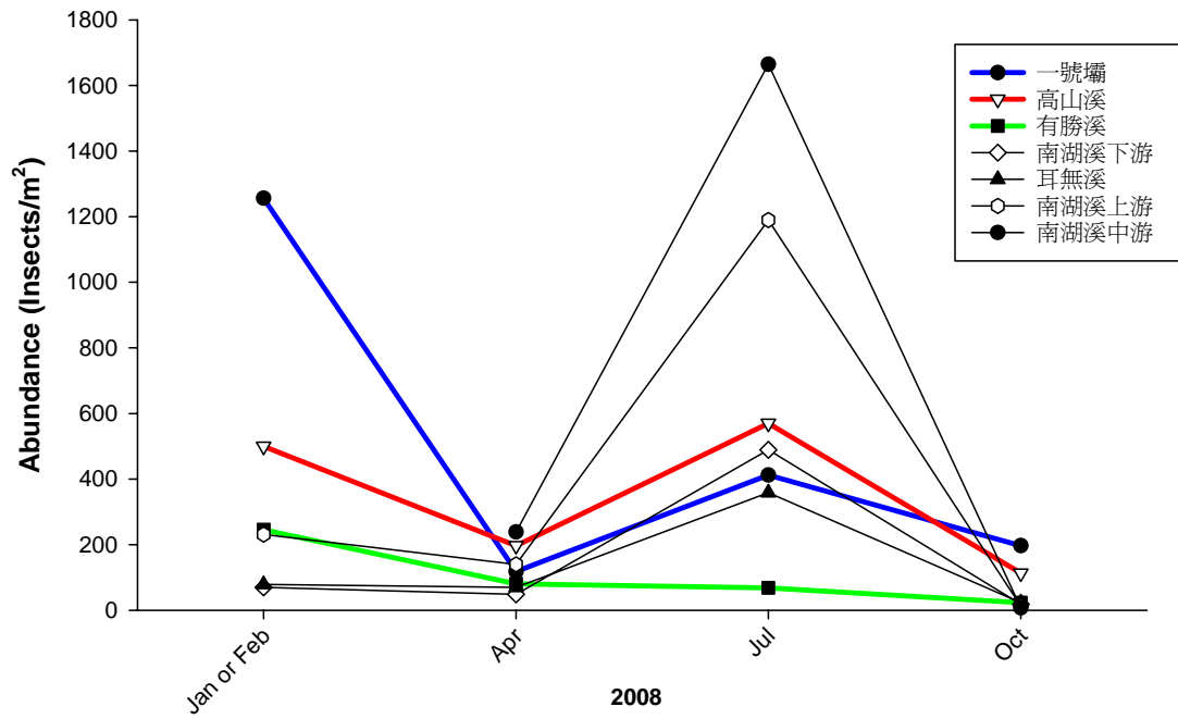
圖 3-6、南湖溪採樣站與武陵地區溪流 3 測站之櫻花鉤吻鮭中大體型昆蟲食 餌(郭及丘，2008)之數量變化圖
