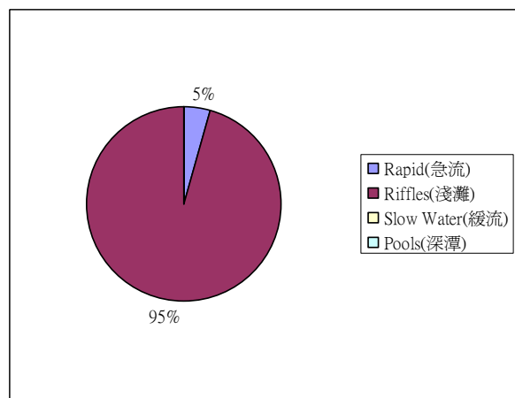
圖 2-17 南湖溪下游棲地環境類型分布 (2008/04)
