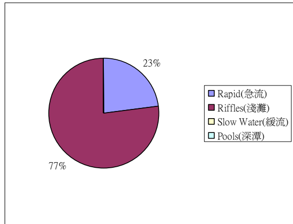
圖 2-19 耳無溪棲地環境類型分布 (2008/04)
