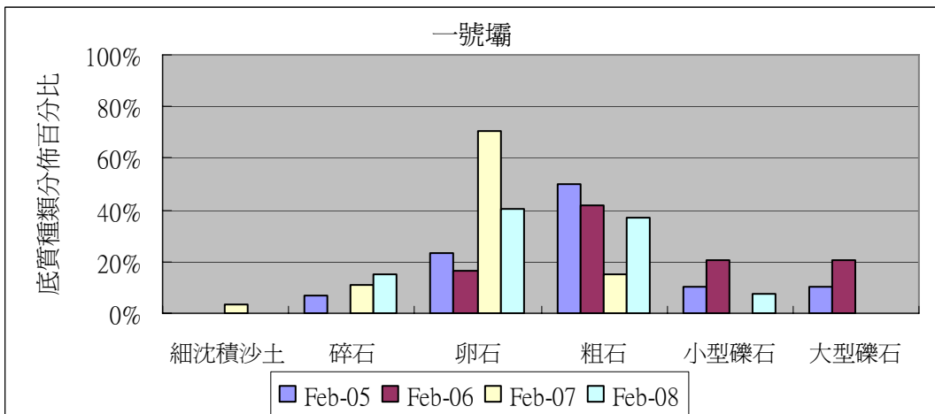
圖 2-28 一號壩 2 月份底質分佈類型百分比圖
