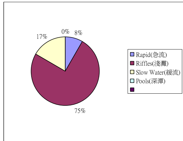
圖 2-13 南湖溪上游棲地環境類型分布 (2008/04)
