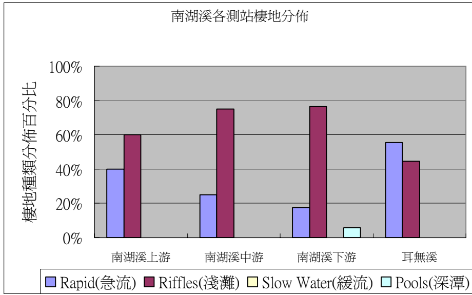
圖 2-21 南湖溪 11 月份各測站棲地分佈類型百分比圖
