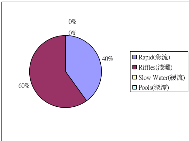
圖 2-12 南湖溪上游棲地環境類型分布 (2008/11)
