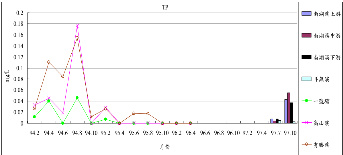
圖 1-17 歷年七家灣溪與南湖溪 2、4、6、7、8、10 月 TP 之變化
