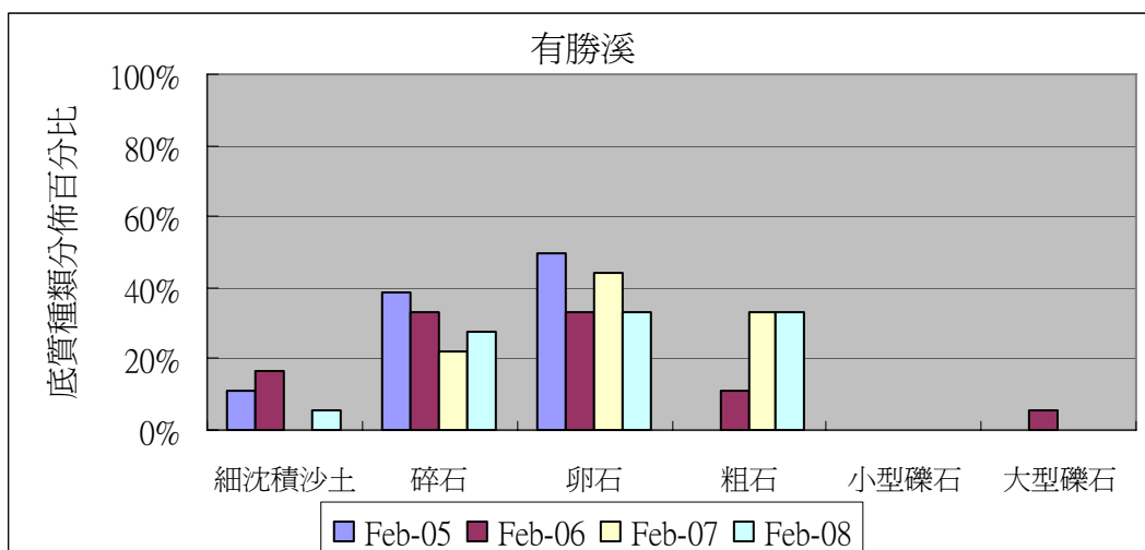
圖 2-24 有勝溪歷年 2 月份底質分佈類型百分比圖
