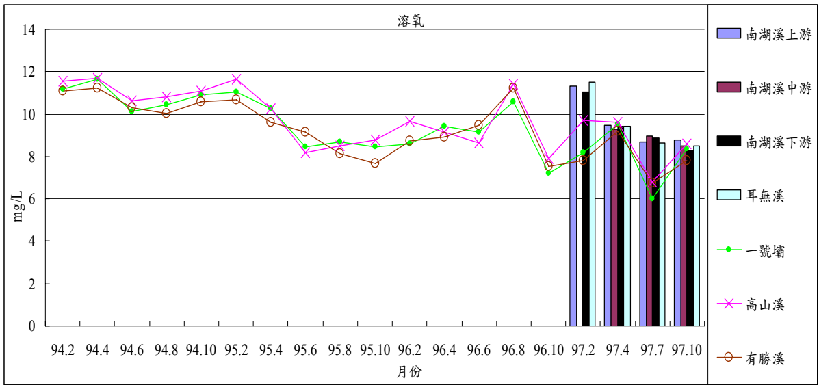
圖 1-7 歷年七家灣溪與南湖溪 2、4、6、7、8、10 月溶氧值之變化
