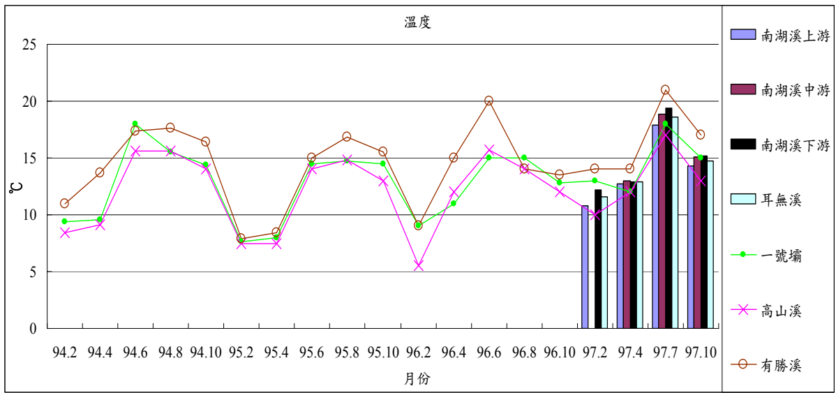
圖 1-5 歷年七家灣溪與南湖溪 2、4、6、7、8、10 月溫度之變化
