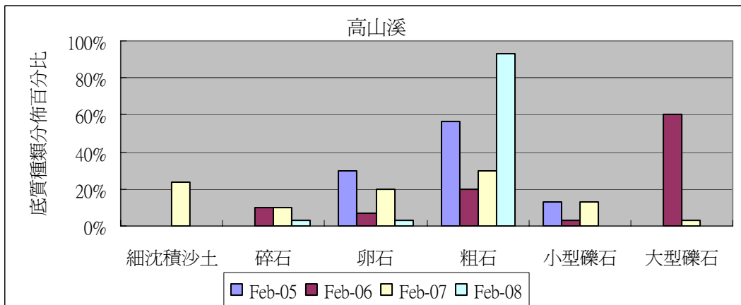
圖 2-32 高山溪 2 月份底質分佈類型百分比圖
