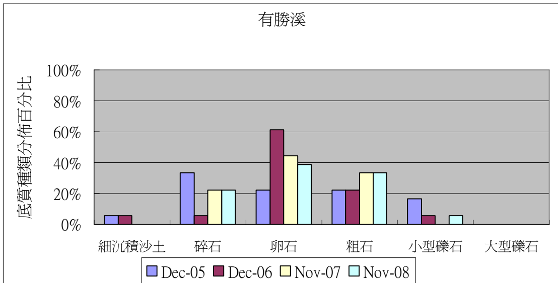
圖 2-25 有勝溪歷年 11 月份底質分佈類型百分比圖
