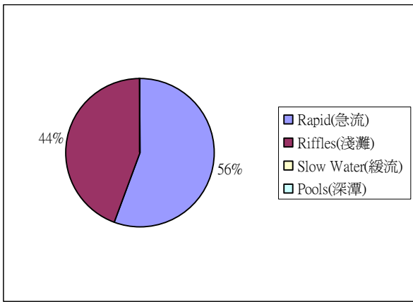
圖 2-18 耳無溪棲地環境類型分布 (2008/11)
