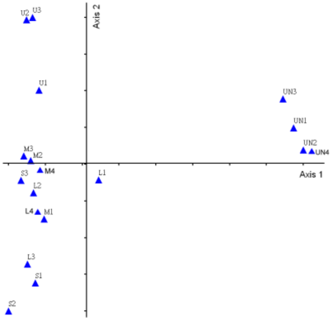
圖 6. 各樣區於 DCA 第一軸與第二軸平面上之分佈位置
