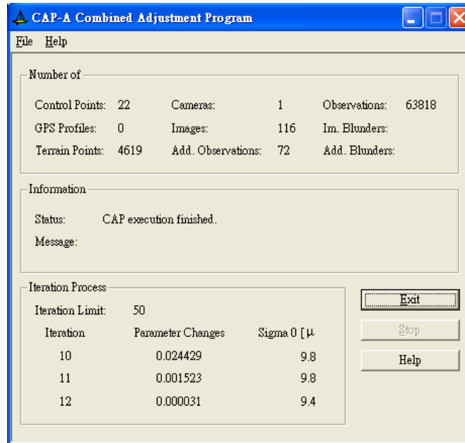
圖 6-103 自率光束法的空三平差結果
