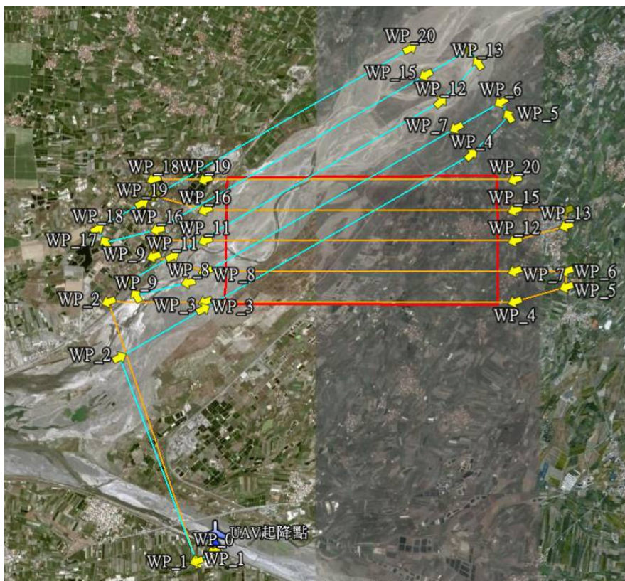
圖 5-15 航帶旋轉前後之飛行計畫比較
