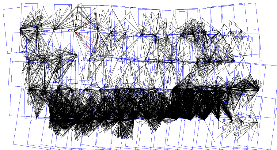
圖 6-36 快速自率光束法空三平差網形
