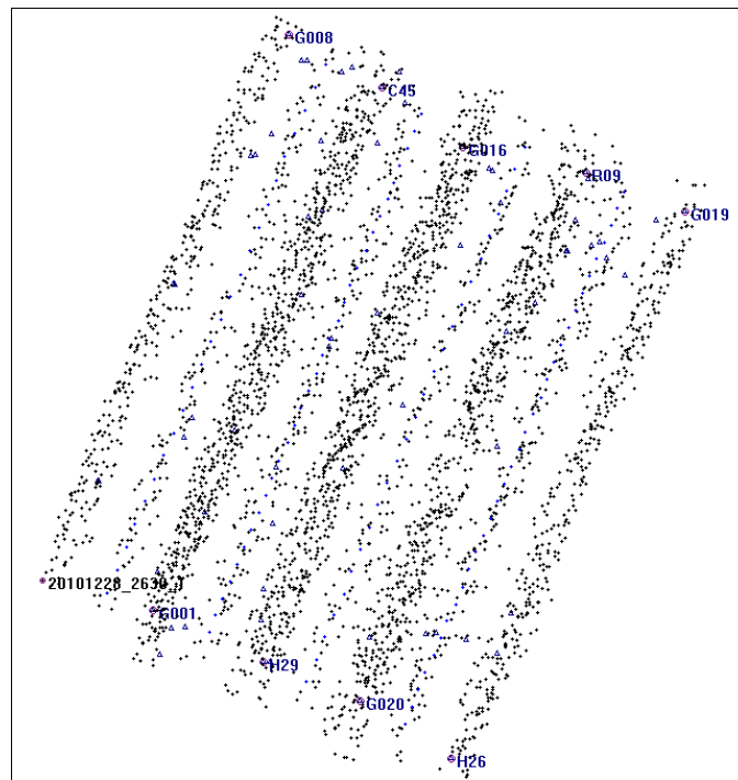
圖 6-68 模擬資料控制點(共 10 點)分布圖
