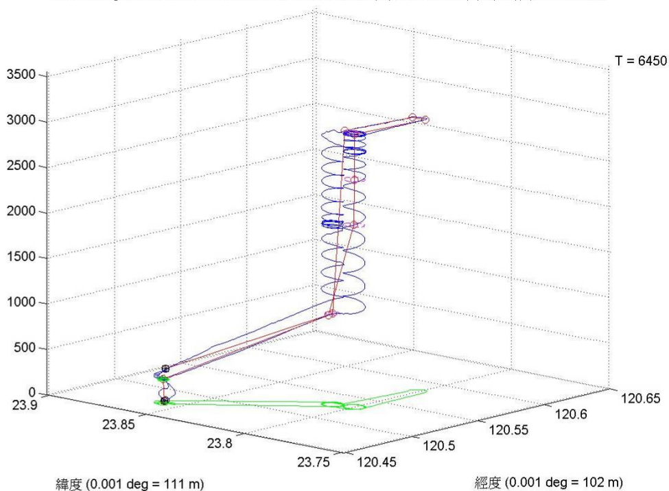
圖 4-14 UAV 3000 公尺高度飛行測試軌跡紀錄圖
