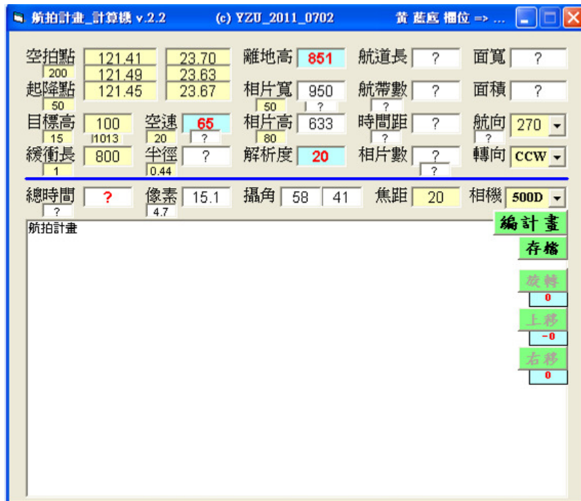
圖 5-4 航拍計畫計算機畫面
