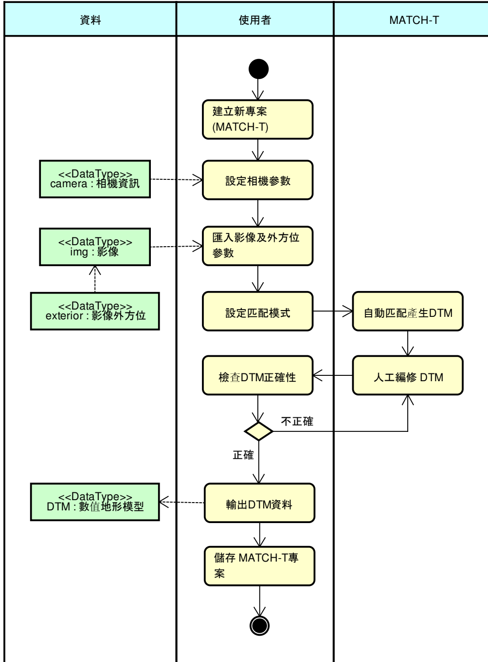
圖 8-14 「自動匹配產生DTM」之使用案例圖
