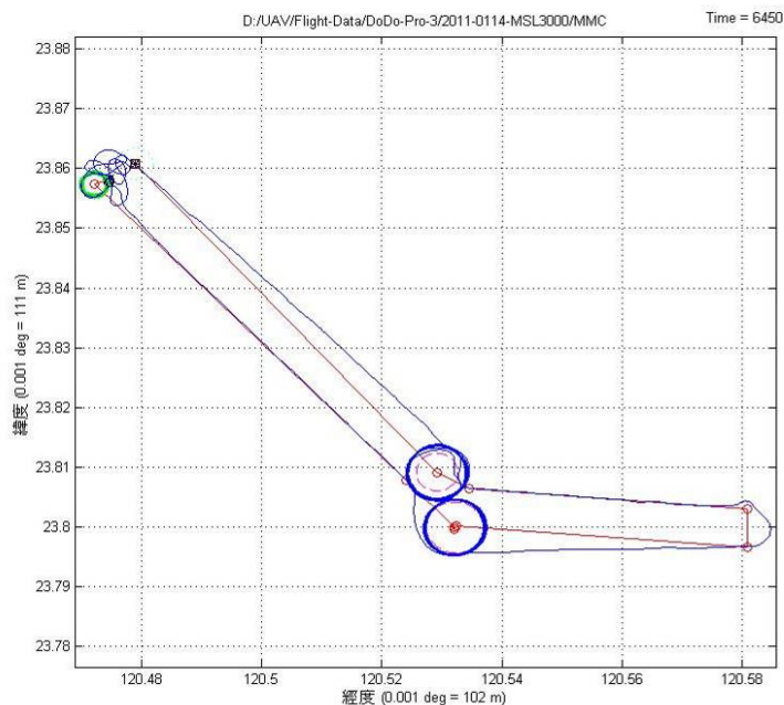
圖 4-16 UAV 飛行路徑(2D)
