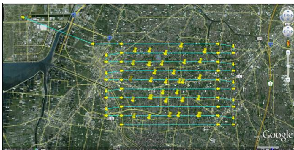
圖 5-25 航高 500m 東西向航拍計畫
