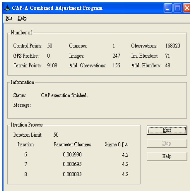
圖 6-92 自率光束法的空三平差結果
