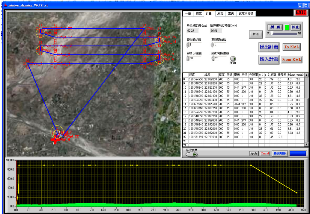
圖 5-10 編修完成之飛行計畫
