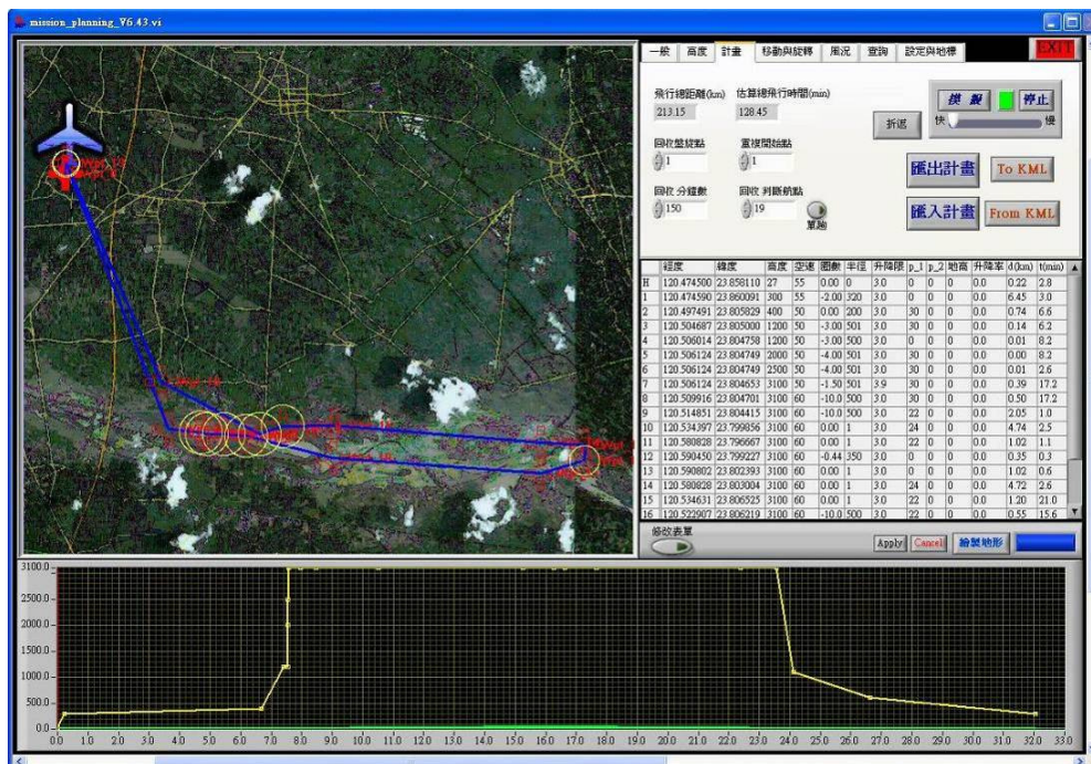
圖 7-10 修改後測試飛行計畫飛行路線
