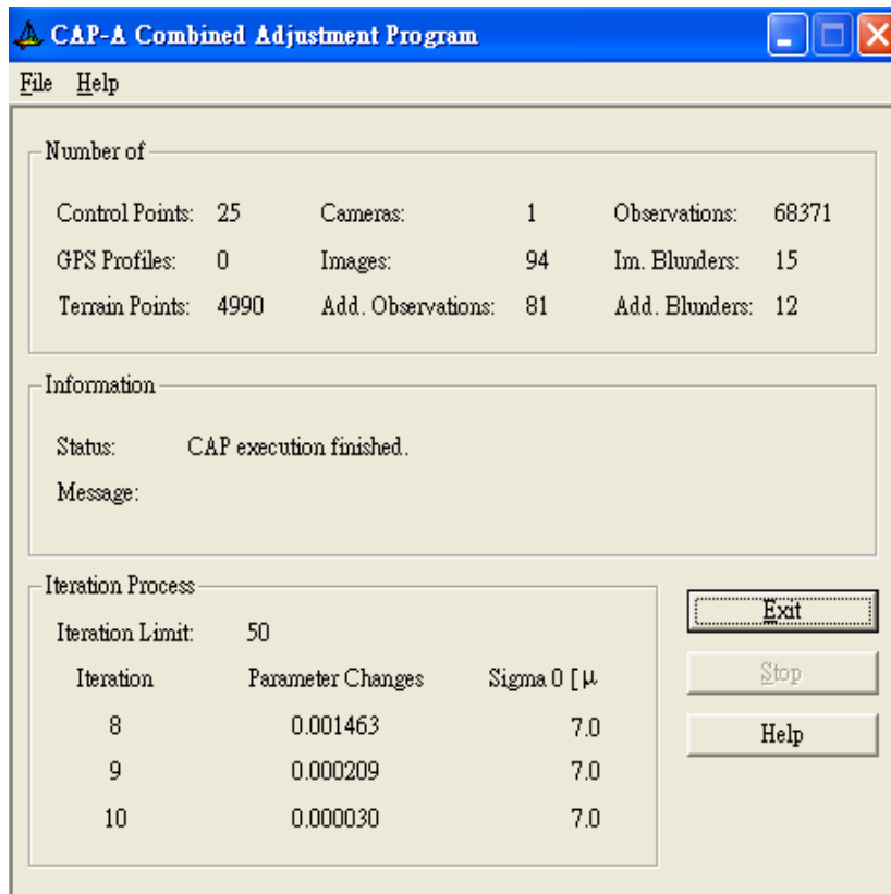
圖 6-111 自率光束法的空三平差結果
