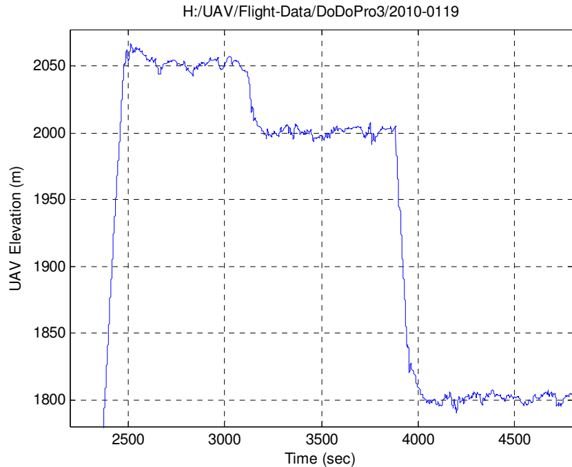
圖 4-3 航高控制 \pm 15 公尺
