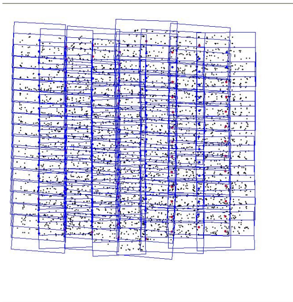
圖 6-27 自率光束法空三平差連結點與控制點分布情形
