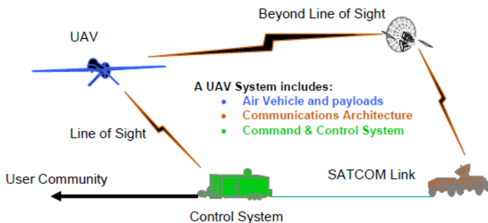
圖 3-7 無人航空系統示意圖(Cox et al., 2006)
