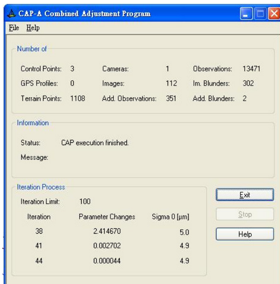
圖 6-11 快速自率光束法空三平差結果
