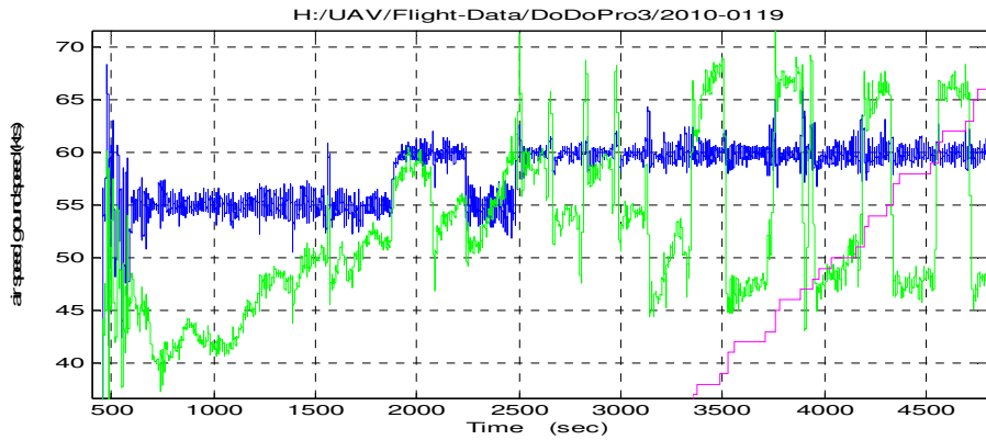
圖 4-2 速度控制精度 \pm 8 km/hr
