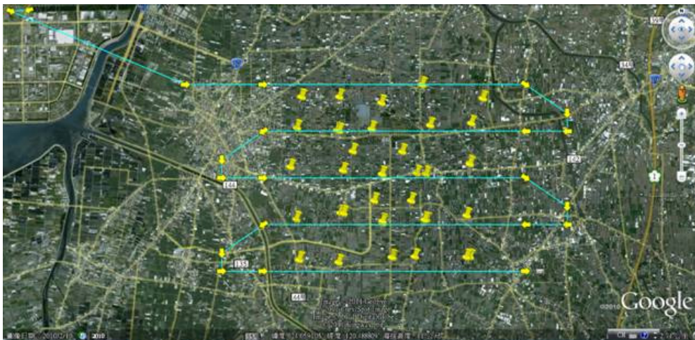
圖 5-26 航高 1000 公尺 東西向航拍計畫
