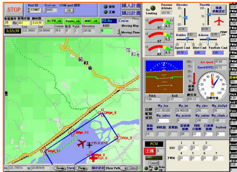
圖 5-1 UAVS 之軌跡規劃與監控畫面
