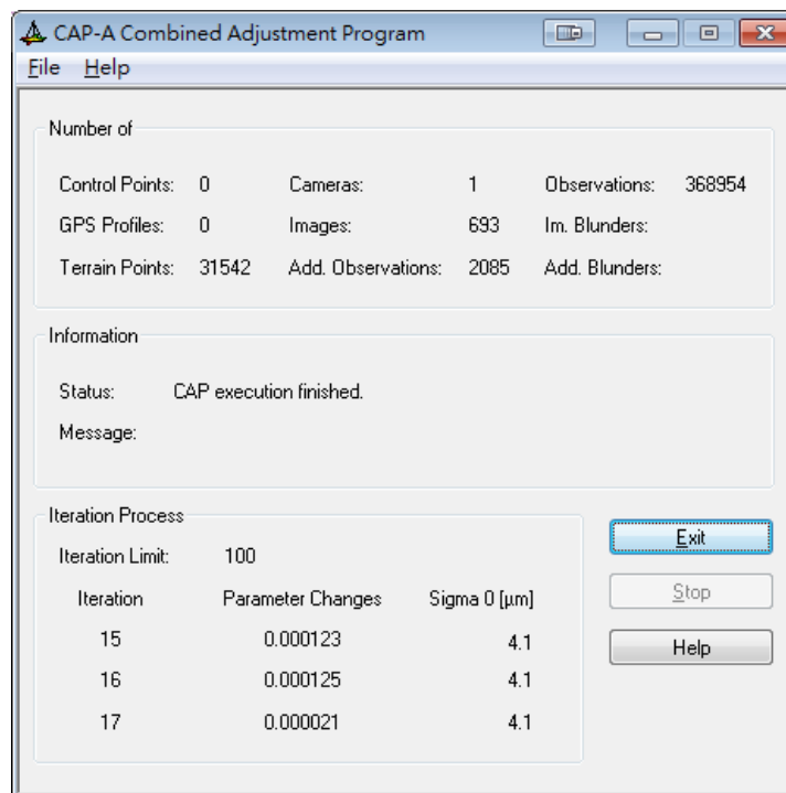
圖 6-82 自由網的自率光束法空三平差結果
