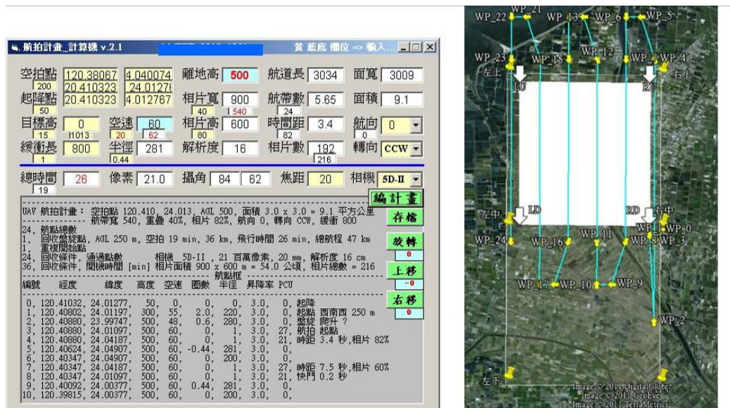
圖 5-3 航拍航線自動規劃軟體
