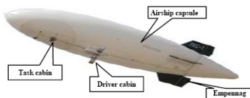
圖 3-13 遙控飛機相關規格
