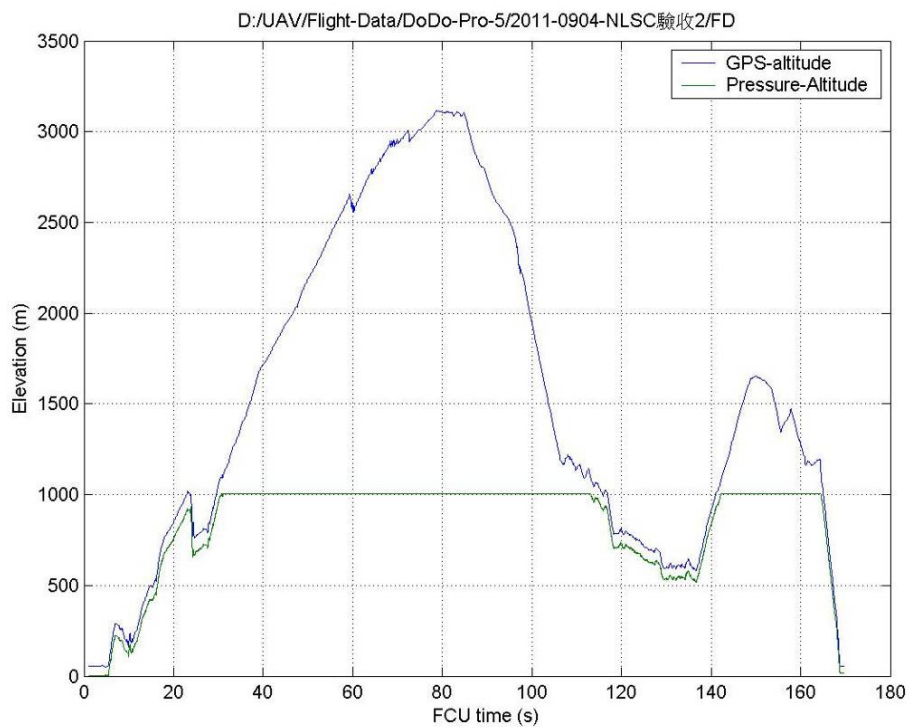
圖 4-26 UAV 3000 公尺高度飛行測試軌跡紀錄圖
