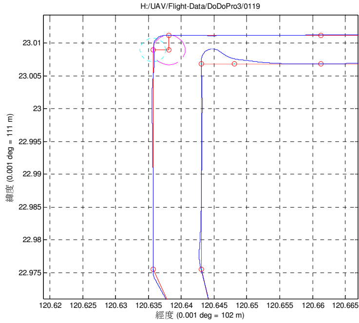
圖 4-4 航線精度 \pm 15 公尺 (進入直線航道 1000 公尺 以後)
