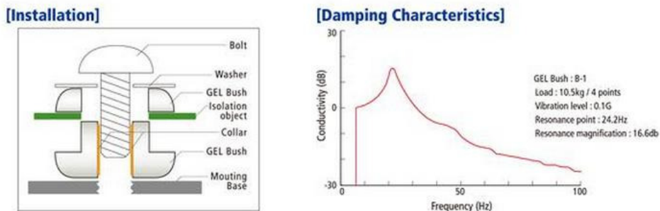
圖 4-11 矽膠避震墊與響應圖
