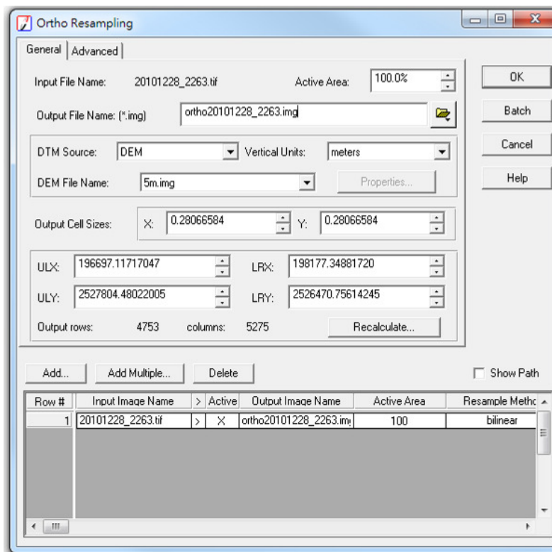
圖 6-20 Ortho Resampling 產生正射影像
