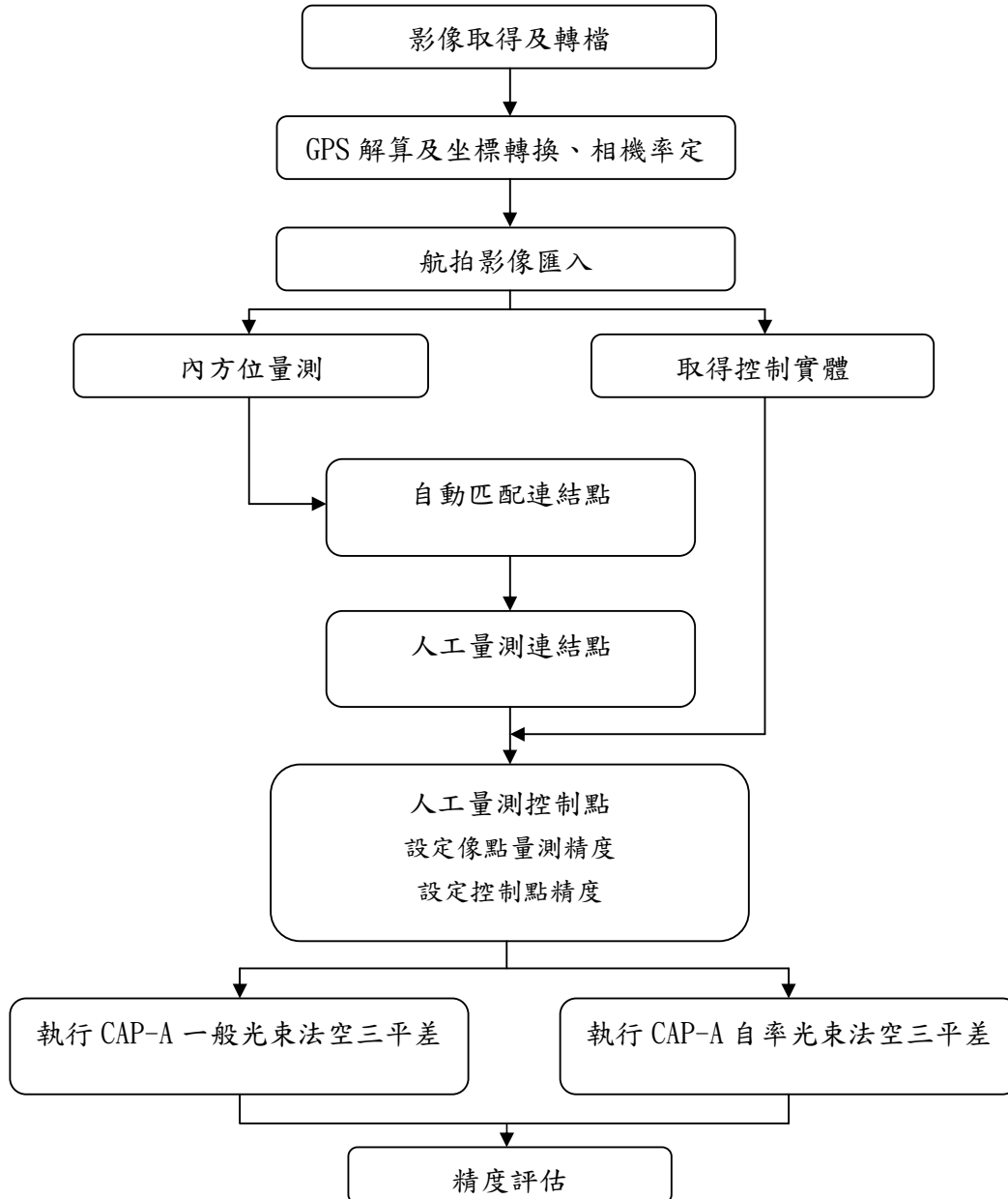
圖 6-60 不同率定方式 LPS ORIMA 空三平差作業流程
