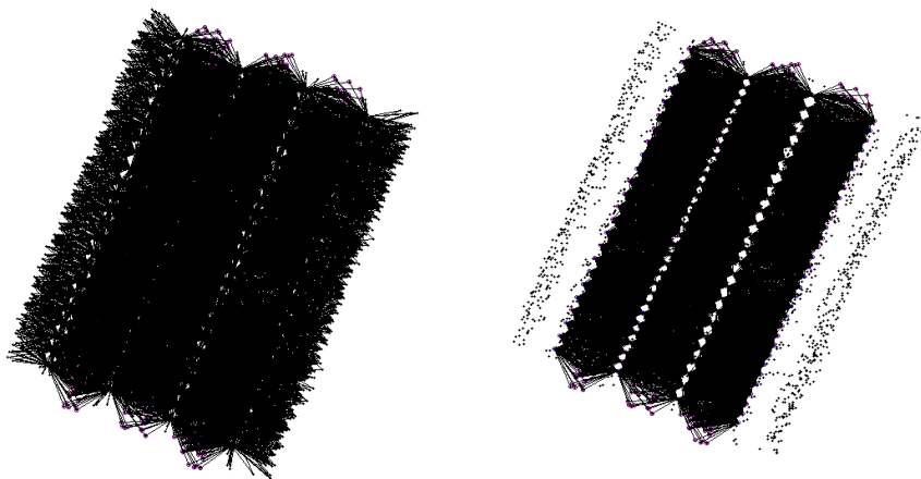
圖 6-66 全測區之網形(左)及航帶間之網形(右)
