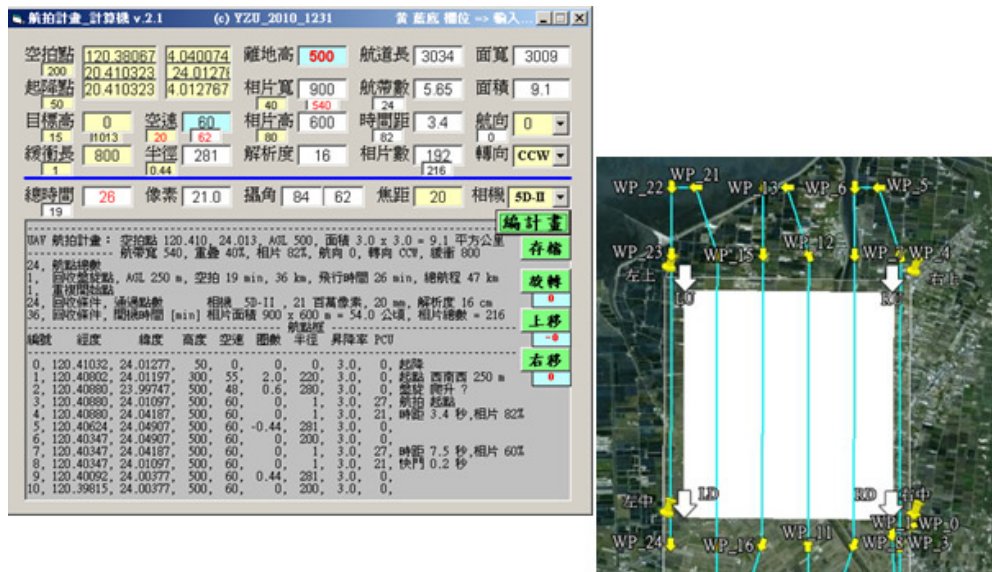
圖 5-36 垂直航拍航線規劃範例
