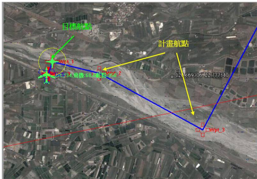
圖 4-21 禁限航區航點設定示意圖
