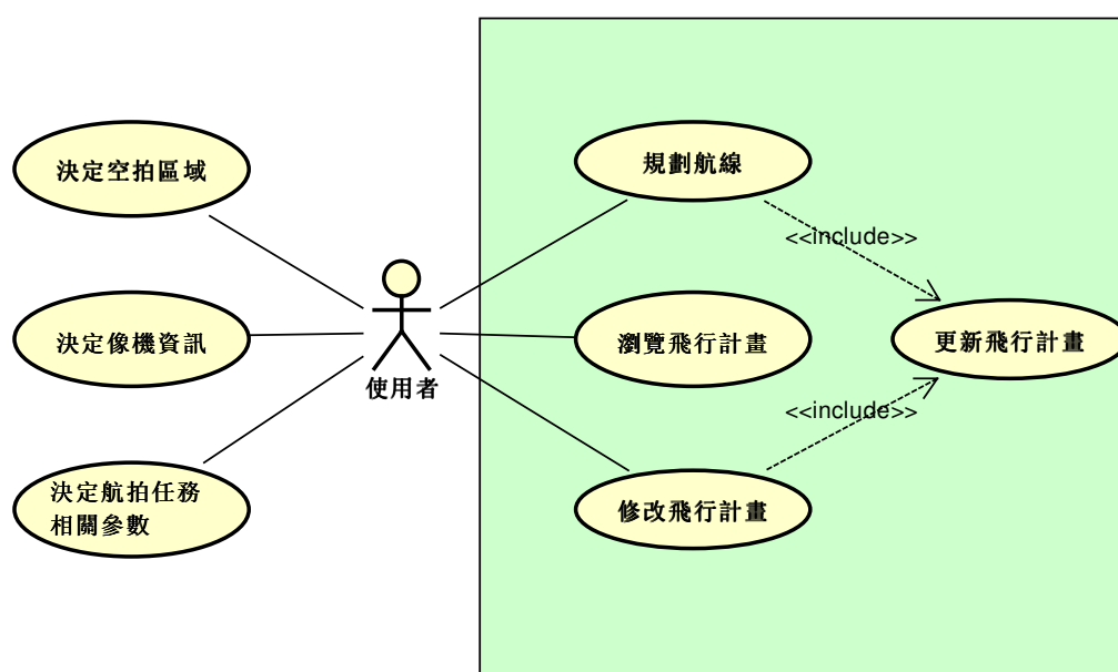
圖 8-4 「航拍任務規劃子系統」之使用案例圖
