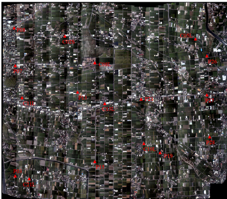
圖 6-88 正射鑲嵌檢核點分布圖
