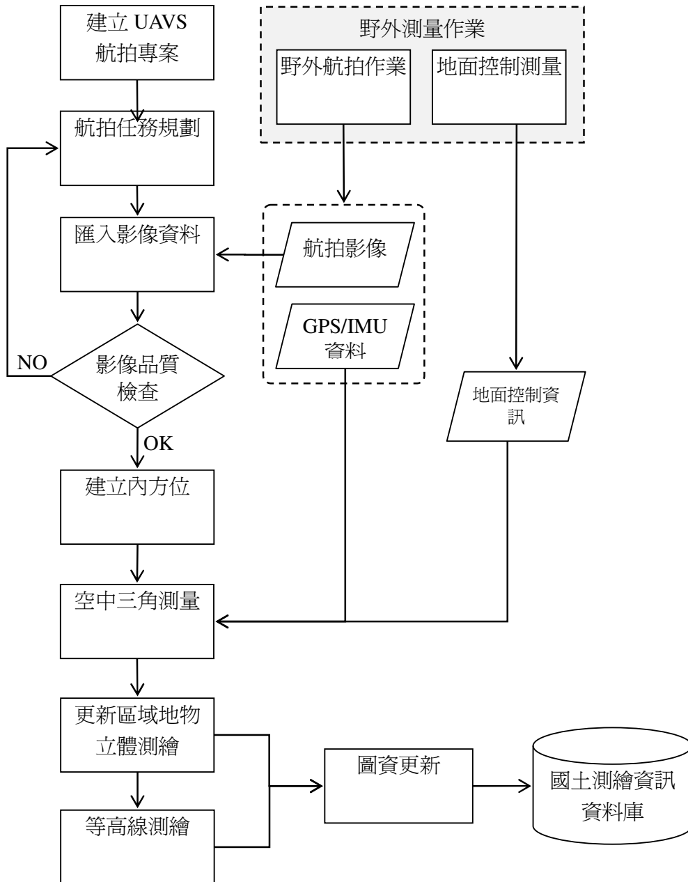
圖 8-9 圖資更新標準作業流程
