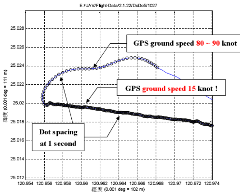
圖 4-6 UAV 於 8 級風下作業紀錄
