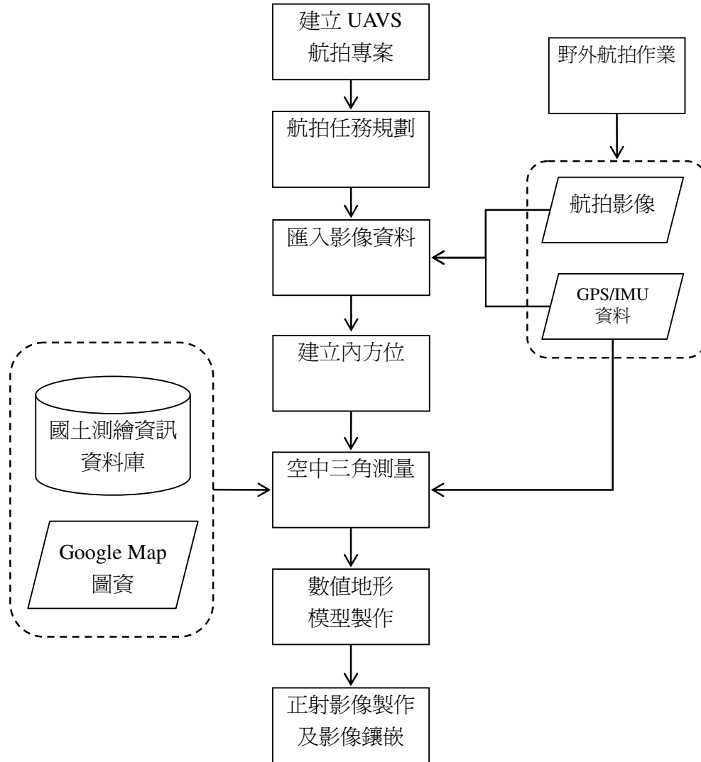
圖 8-5 快速影像正射及鑲嵌之作業流程圖
