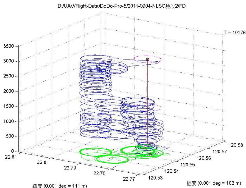
圖 4-28 UAV 飛行路徑(3D)
