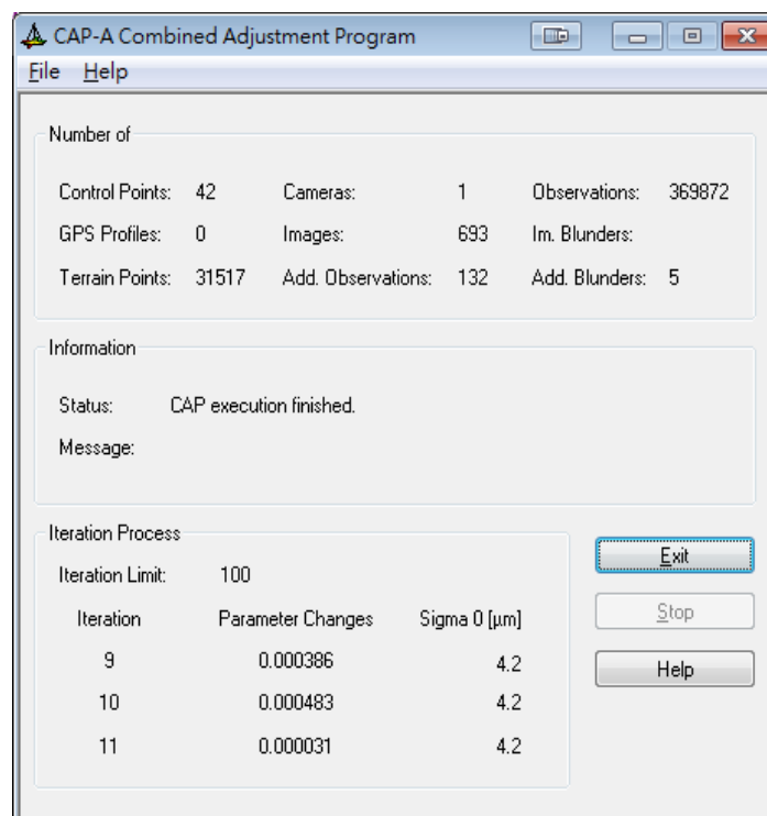
圖 6-83 自率光束法的空三平差結果
