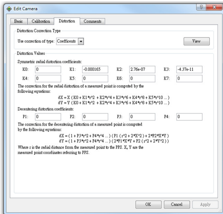
圖 6-14 相機參數設定(Distortion)
