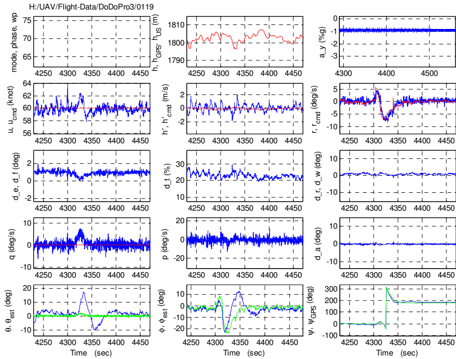
圖 4-5 俯仰 (pitch) 與 滾轉 (roll) 角 \pm 2 度以內
