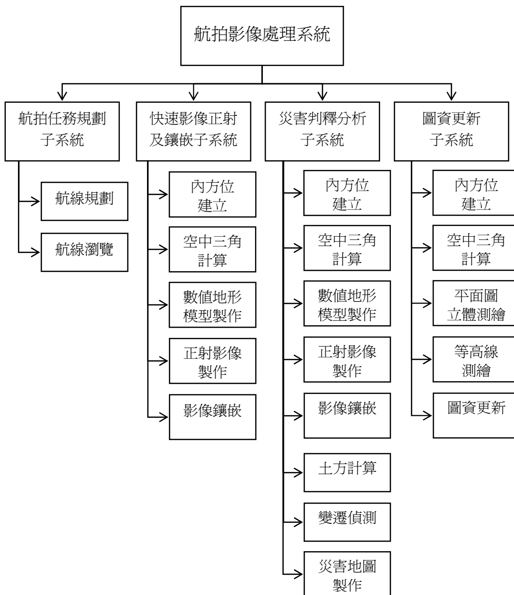
圖 8-2 航拍影像處理系統架構圖
