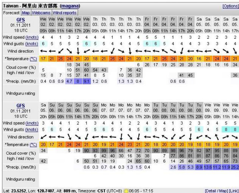
圖 5-32 WindGuru 溫度與雲況預估網頁
