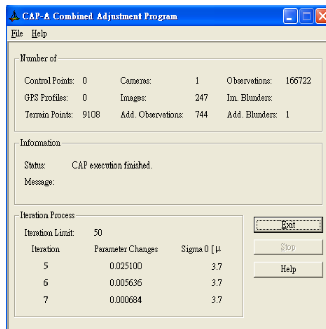
圖 6-91 自由網的自率光束法空三平差結果
