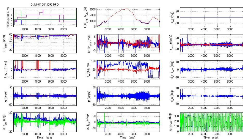
圖 4-29 UAV 高空飛行數據紀錄
