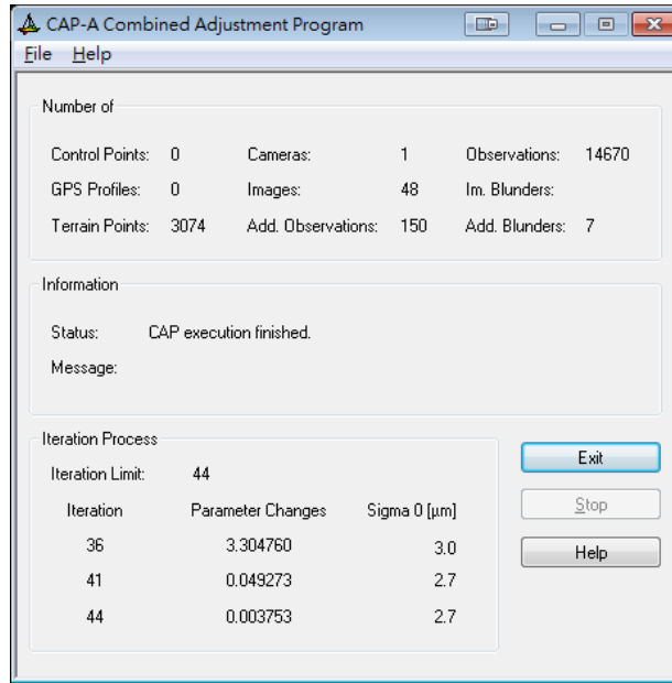
圖 6-53 快速自率光束法空三平差結果
