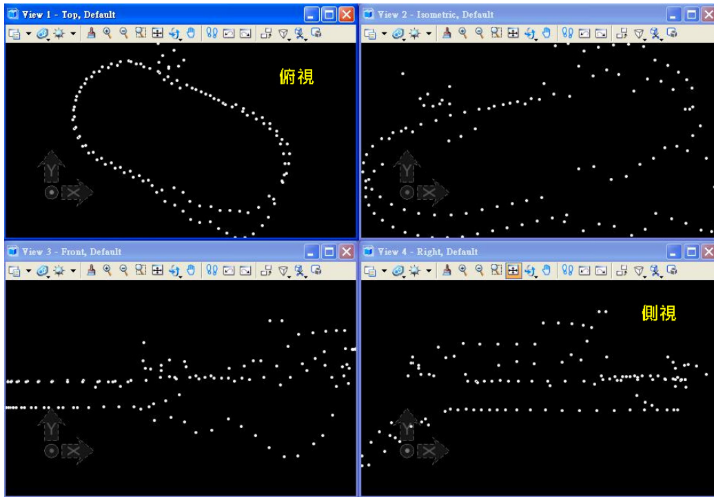
圖 6-74 第二次試驗坐標解算成果圖
