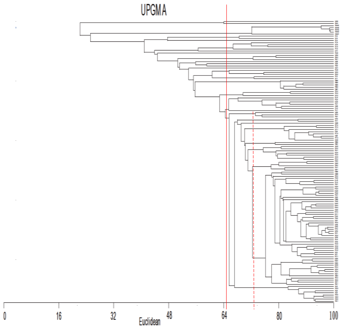
圖 3-1 金門地區 1x50 m 2 帶狀樣區海岸植群樹狀圖(資料來源本研究)
