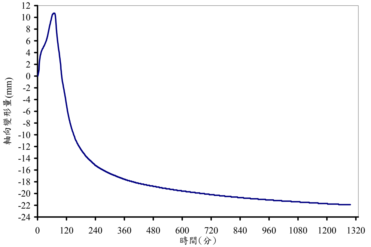
圖 10 軸向變形量歷時曲線圖
