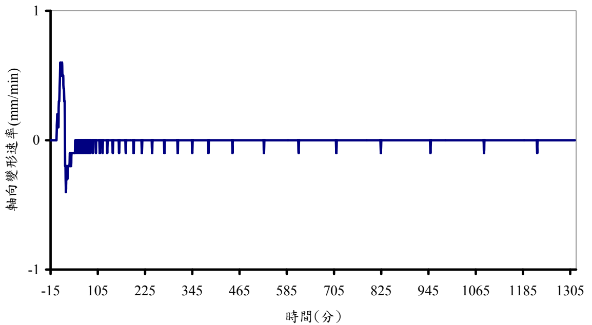
圖 11 軸向變形速率歷時曲線圖
