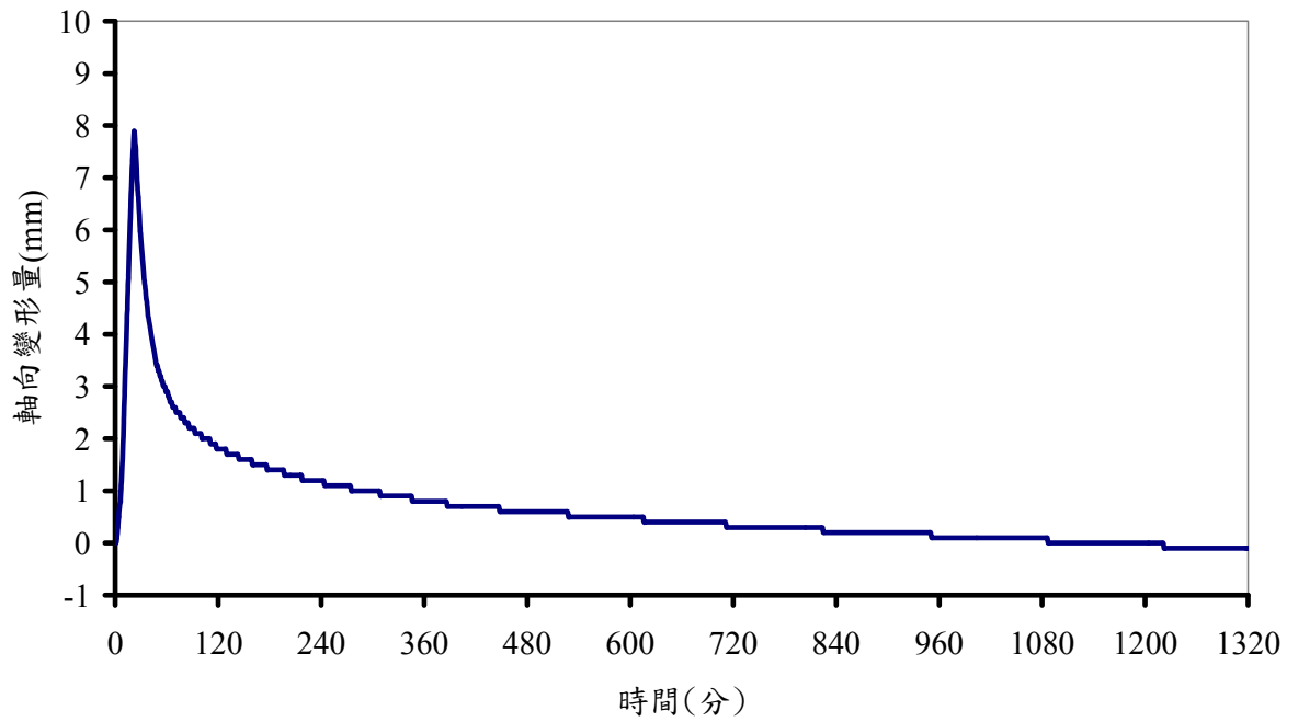
圖 10 軸向變形量歷時曲線圖
