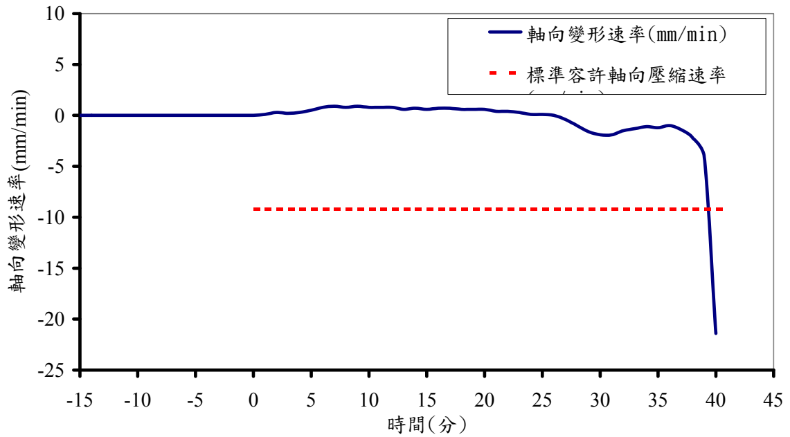
圖 10 軸向變形速率歷時曲線圖
