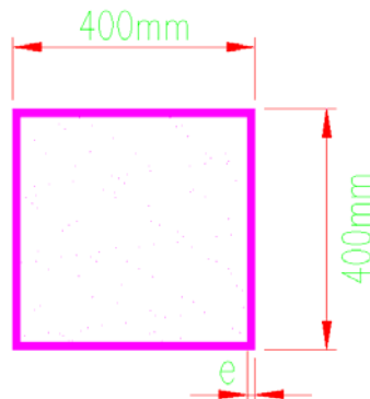
圖1 試體斷面
