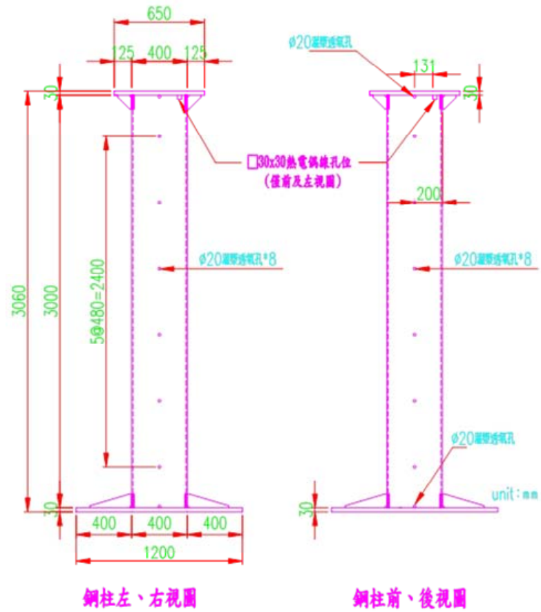
圖 4 試體立面圖
