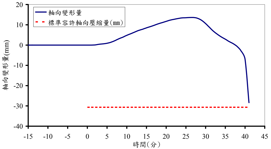
圖 9 軸向變形量歷時曲線圖
