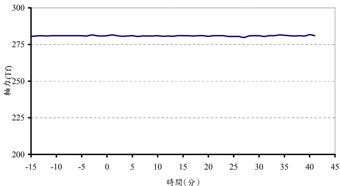
圖 7 加載歷時曲線圖
