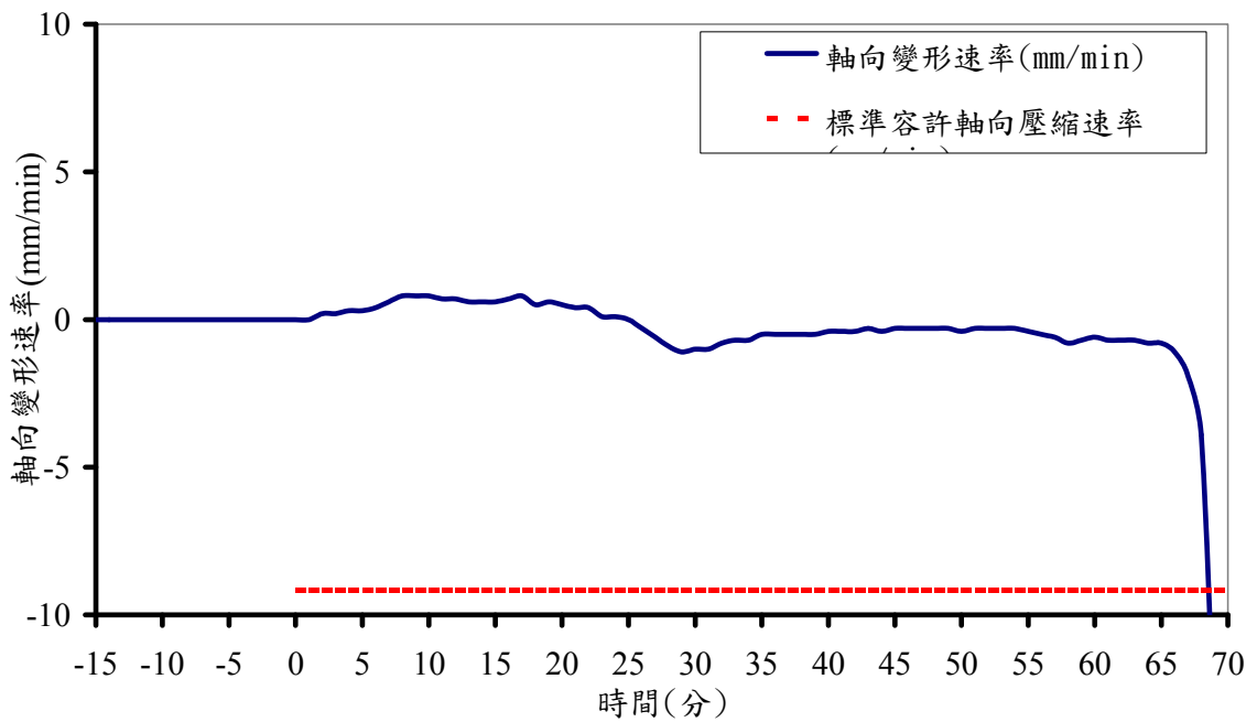
圖 10 軸向變形速率歷時曲線圖
