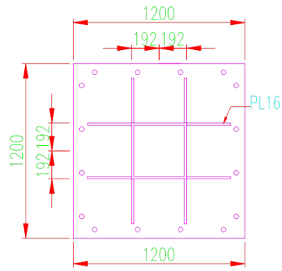
(c) 試體下部加勁板
