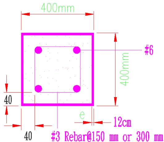
圖1 試體斷面
