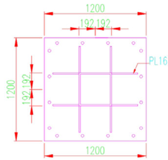
(c) 試體下部加勁板
