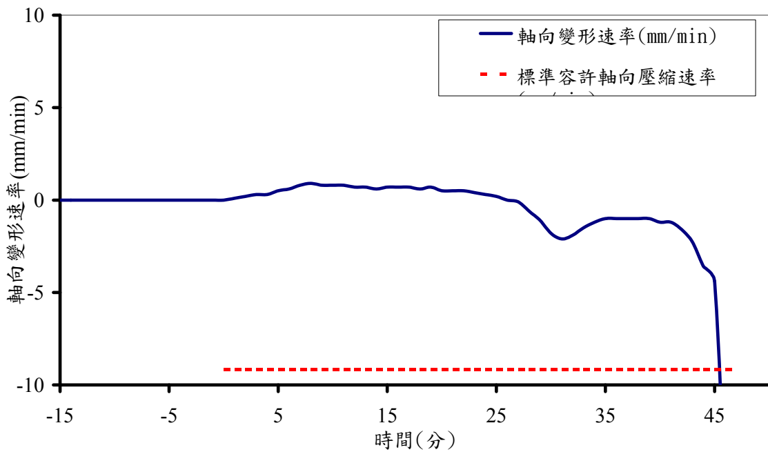
圖 10 軸向變形速率歷時曲線圖
