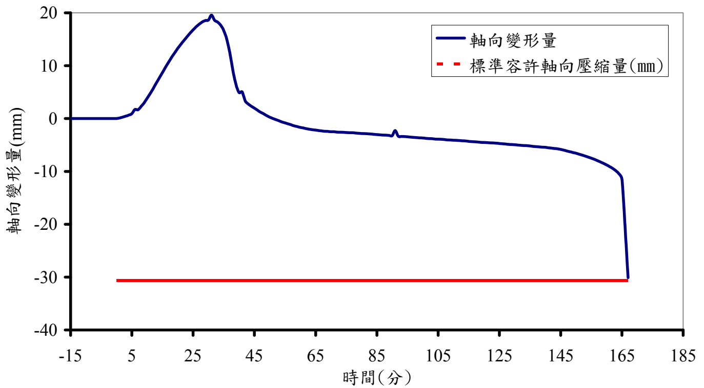
圖7 軸向變形量歷時曲線圖
