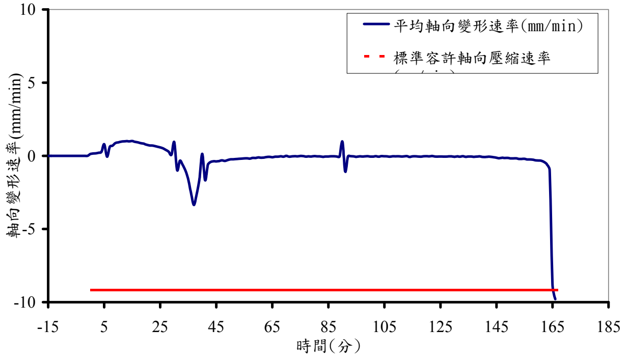
圖 8 軸向變形速率歷時曲線圖
