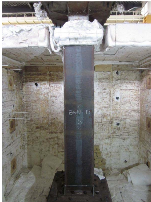
照片2：加載及加熱試驗前試體安裝
