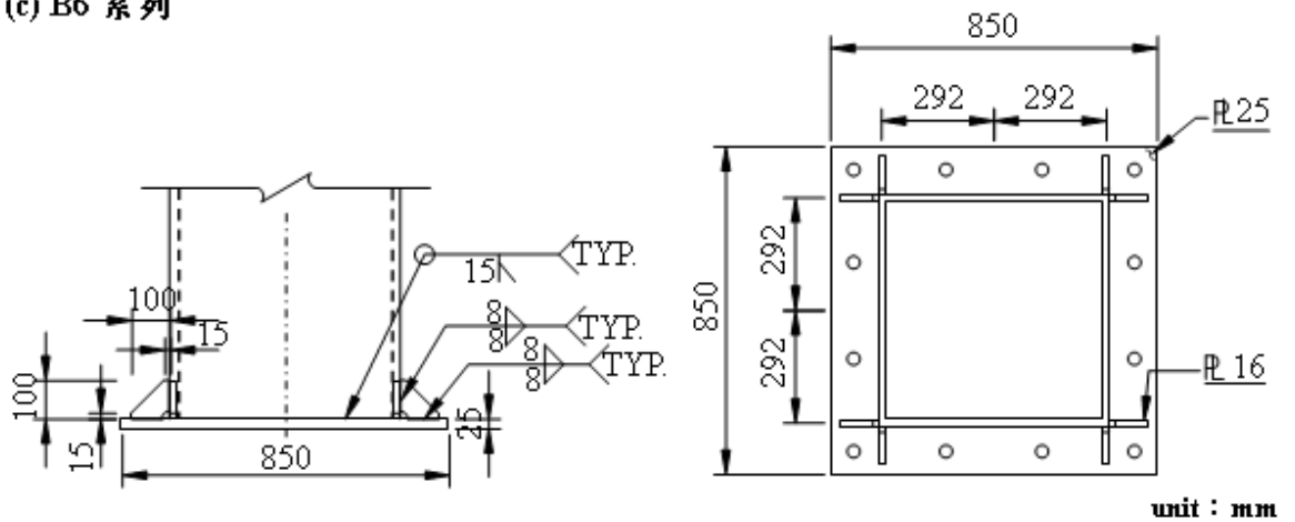
圖2 柱底端板
