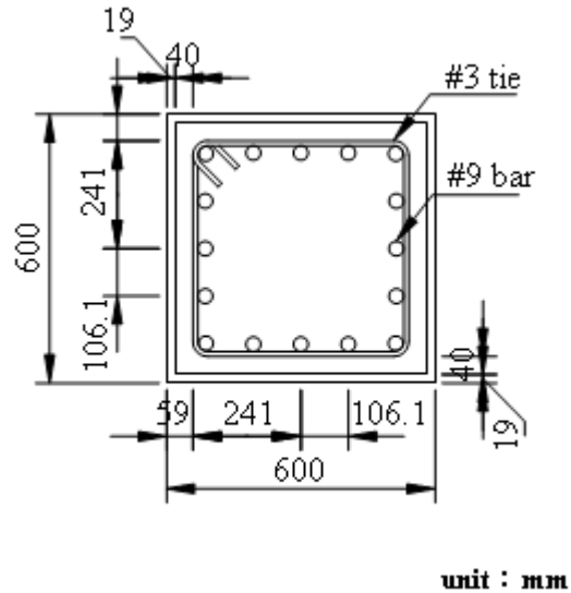
圖1 試體斷面
