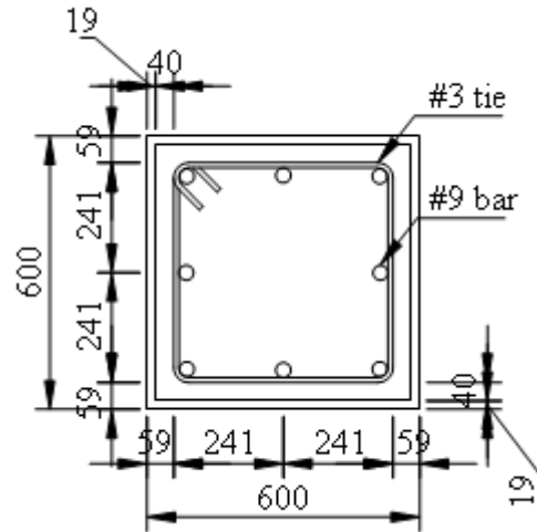
圖1 試體斷面
