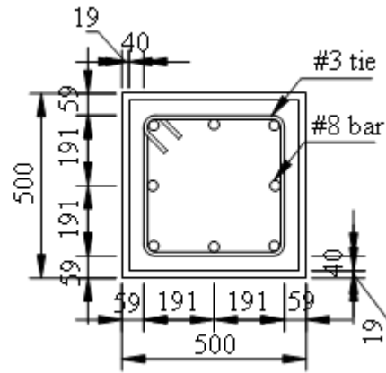
圖1 試體斷面
