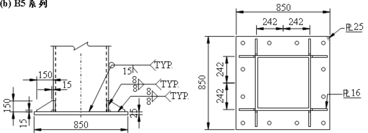
圖2 柱底端板
