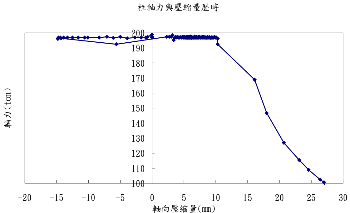
圖 11 軸力與軸向壓縮量歷時曲線圖
