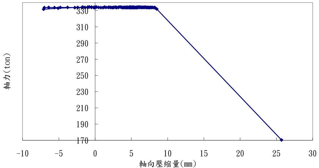
圖 11 軸力與軸向壓縮量歷時曲線圖
