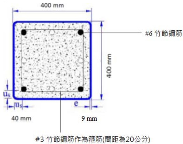
圖1 試體斷面
