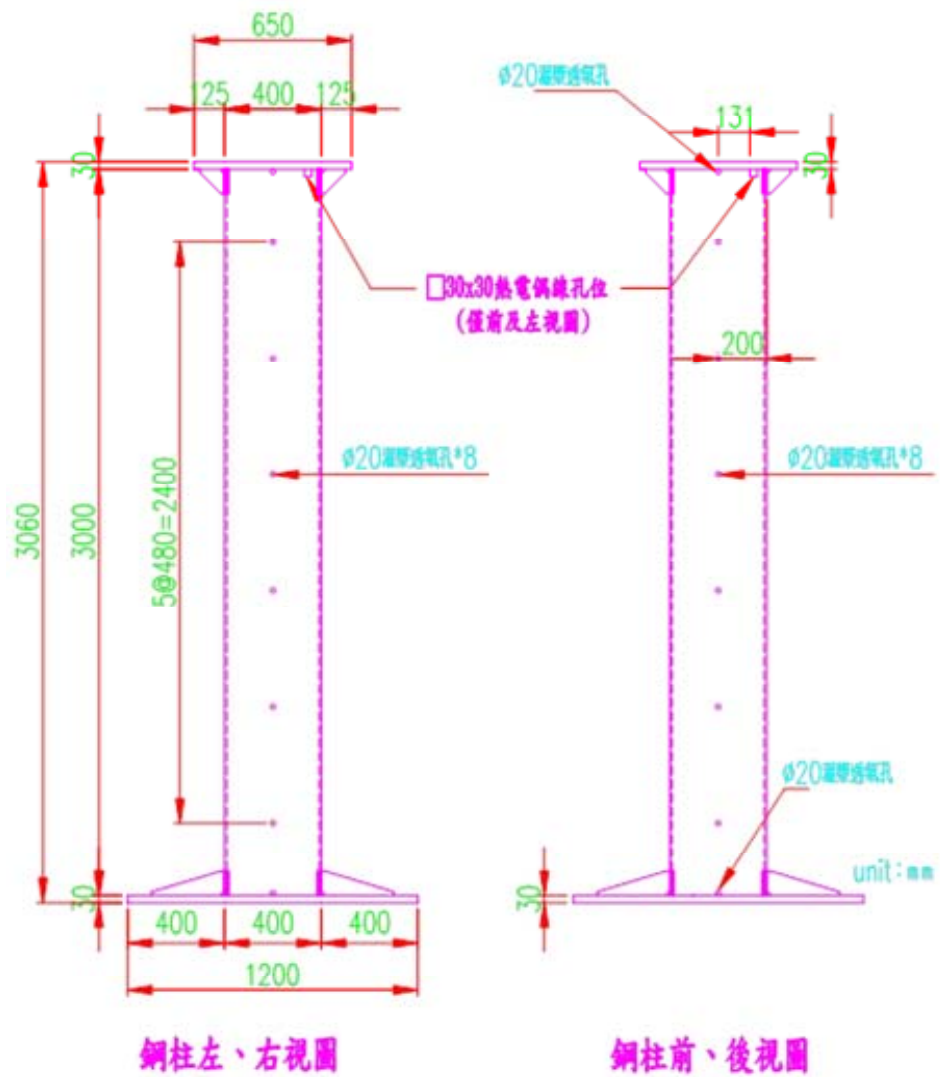
圖 4 試體立面圖
