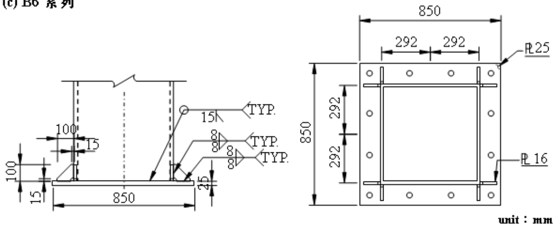
圖2 柱底端板
