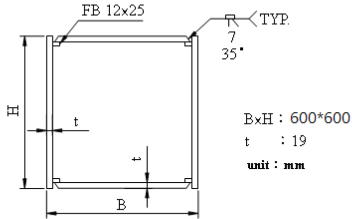
圖1 試體斷面
