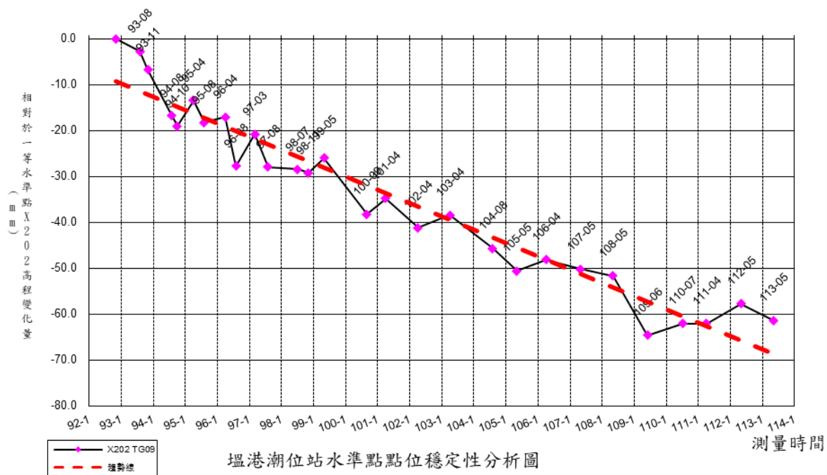
圖 5-6 塭港潮位站水準點 TG09 相對一等水準點 X202 之高程差變化圖
