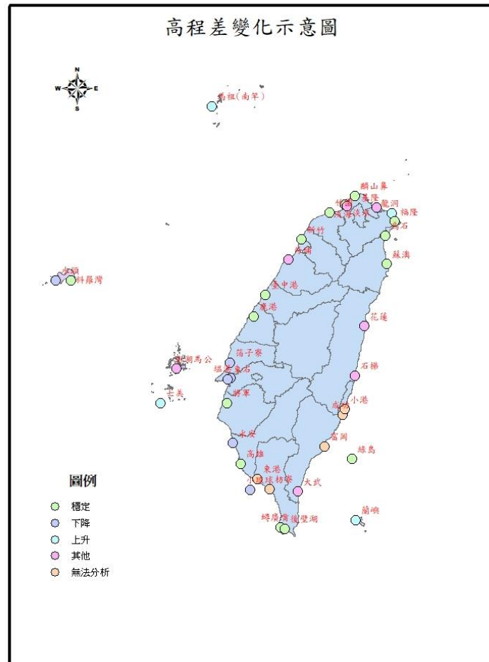
圖 5-4 各潮位站水準點相對於一等水準點高程差變化示意圖
