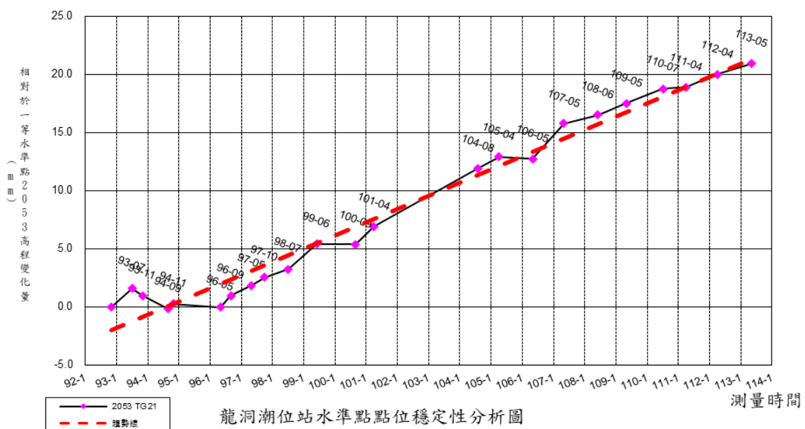
圖 5-12 洞潮位站水準點 TG21 相對一等水準點 2053 之高程差變化圖
