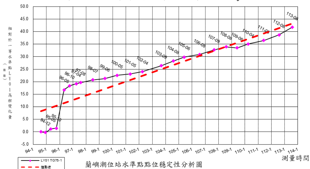
圖 5-14 蘭嶼潮位站水準點 TG75-1 相對一等水準點 LY01 之高程差變化圖
