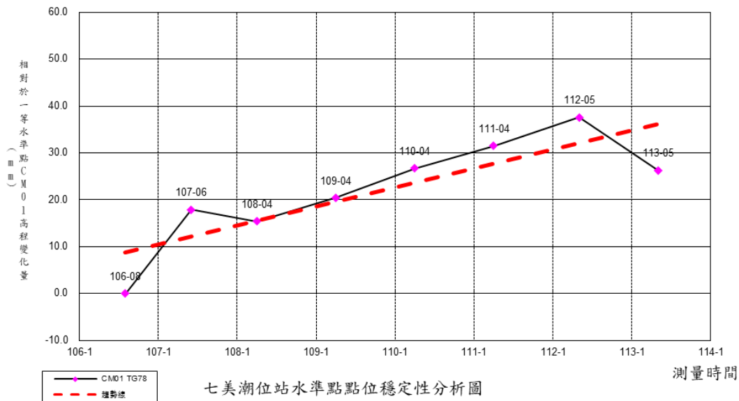
圖 5-15 七美潮位站水準點 TG78 相對水準點 CM01 之高程差變化圖
