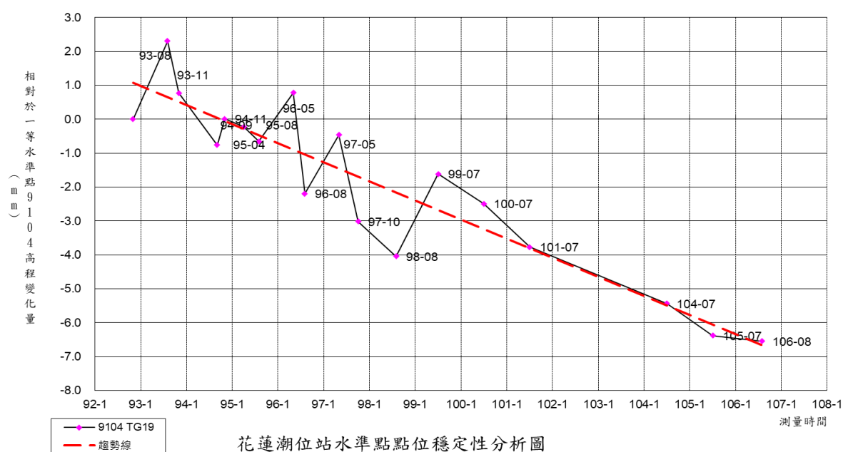
圖 5-17A 花蓮潮位站水準點 TG19 相對一等水準點 9104 之高程差變化圖
