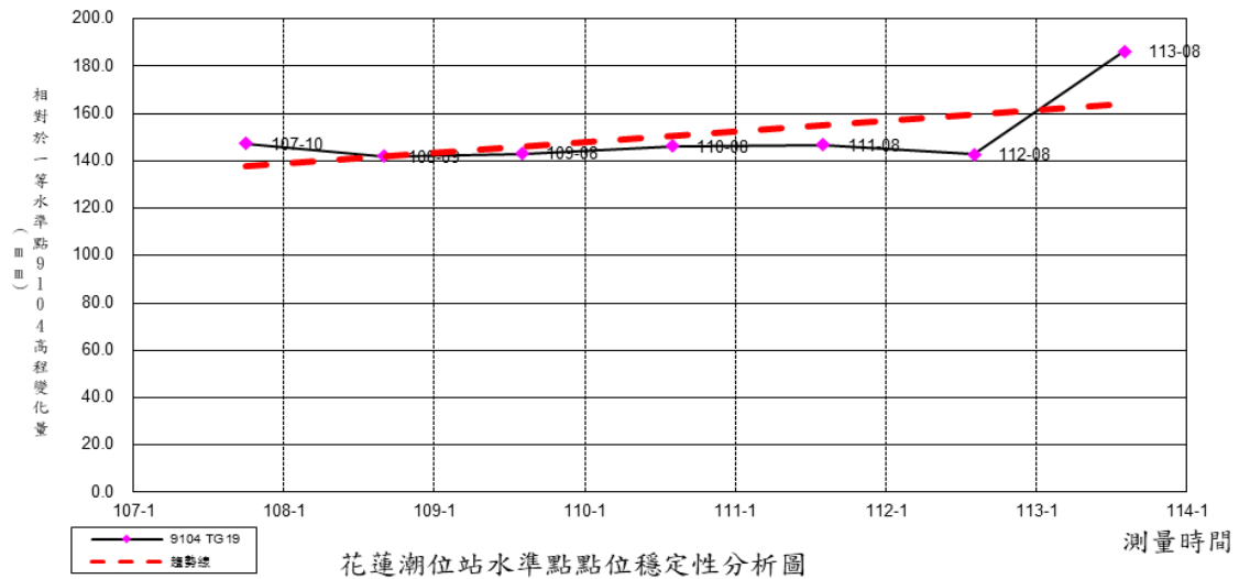
圖 5-17B 花蓮潮位站水準點 TG19 相對一等水準點 9104 之高程差變化圖
