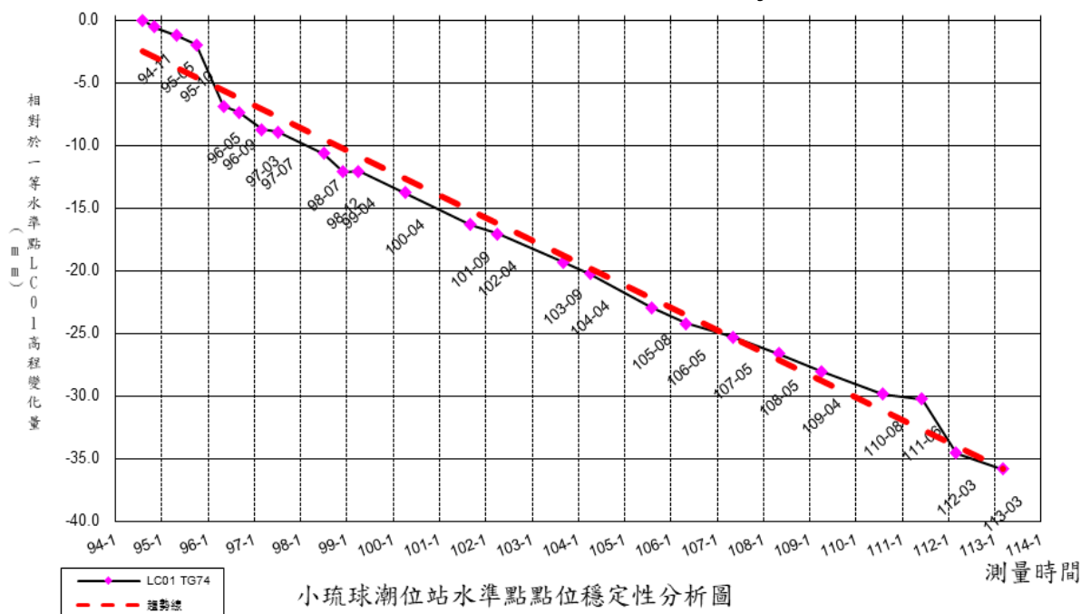
圖 5-10 小琉球潮位站水準點 TG74 相對一等水準點 LC01 之高程差變化圖
