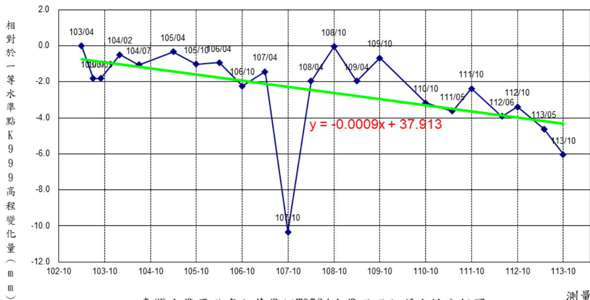
臺灣水準原點高程基準網T0524水準點點位穩定性分析圖
