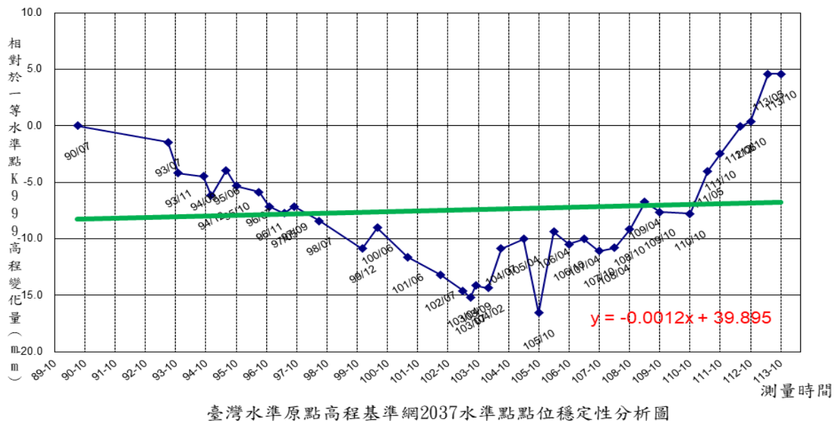
圖 5-3 2037 水準點相對於水準原點 K999 之高程差變化圖
