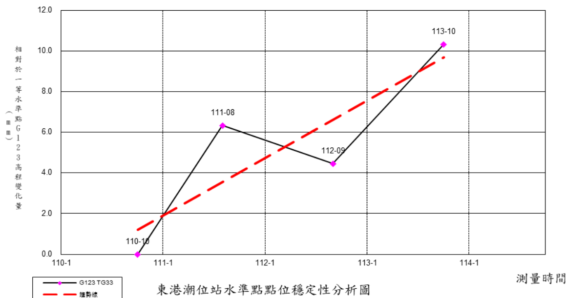
圖 5-22 東港潮位站水準點 TG33 相對水準點 G123 之高程差變化圖
