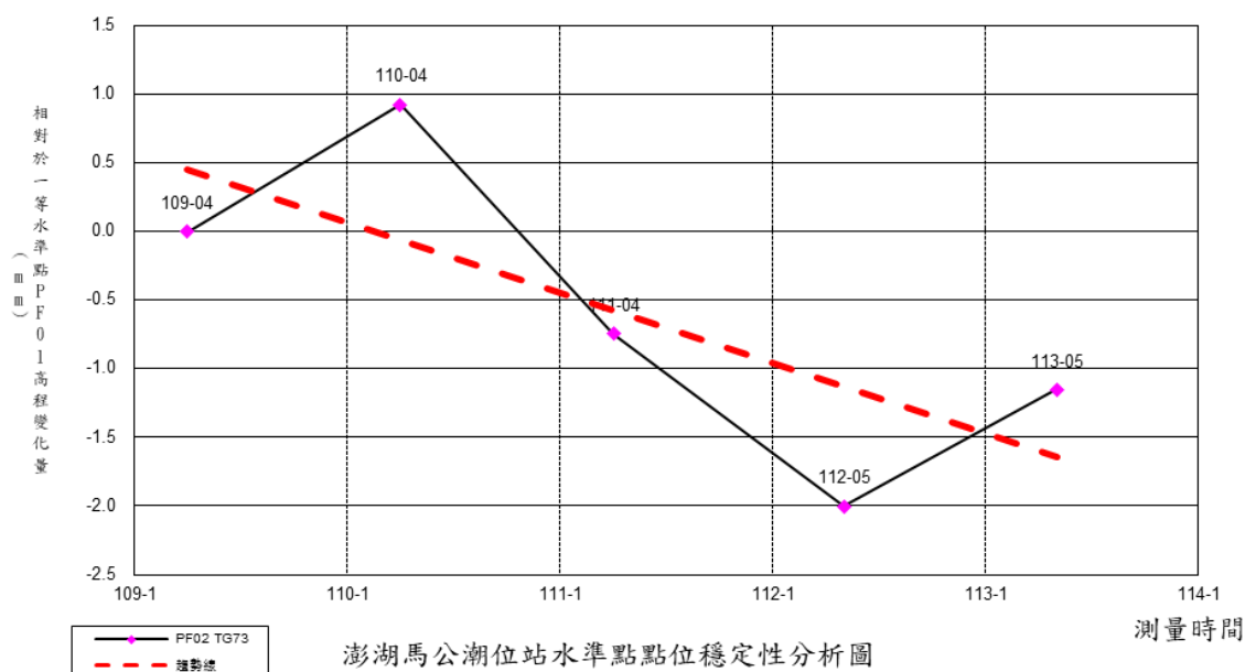
圖 5-23 澎湖馬公潮位站水準點 TG73 相對一等水準點 PF02 之高程差變化圖
