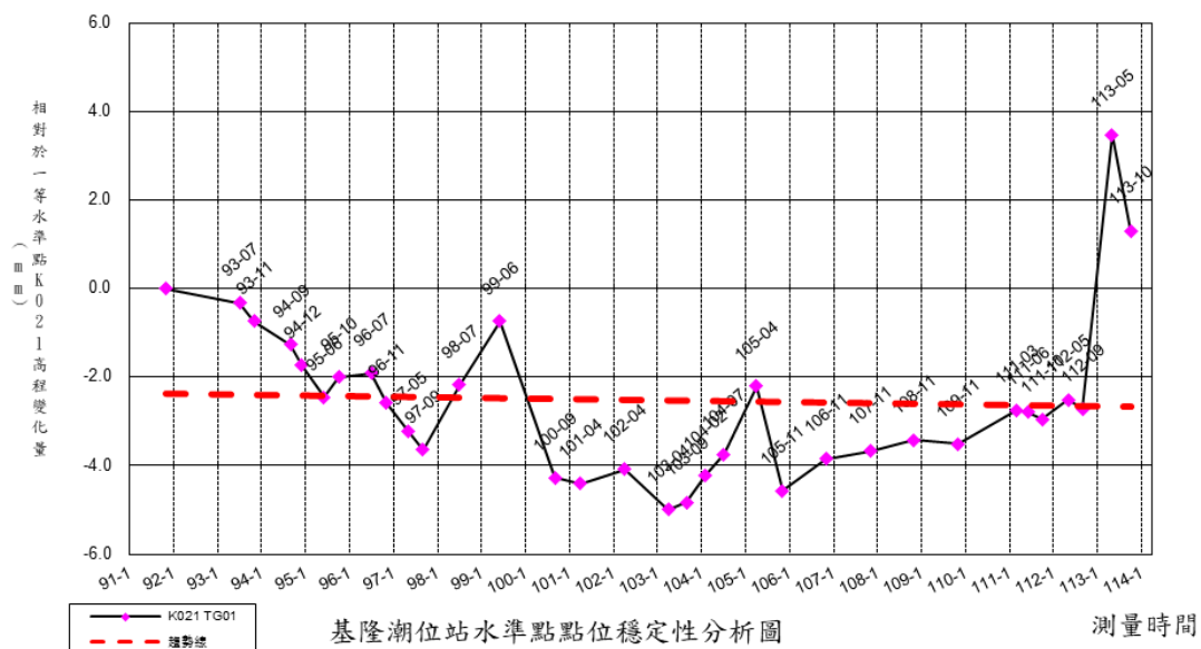
圖 5-16 基隆潮位站水準點 TG01 相對水準點 K021 之高程差變化圖
