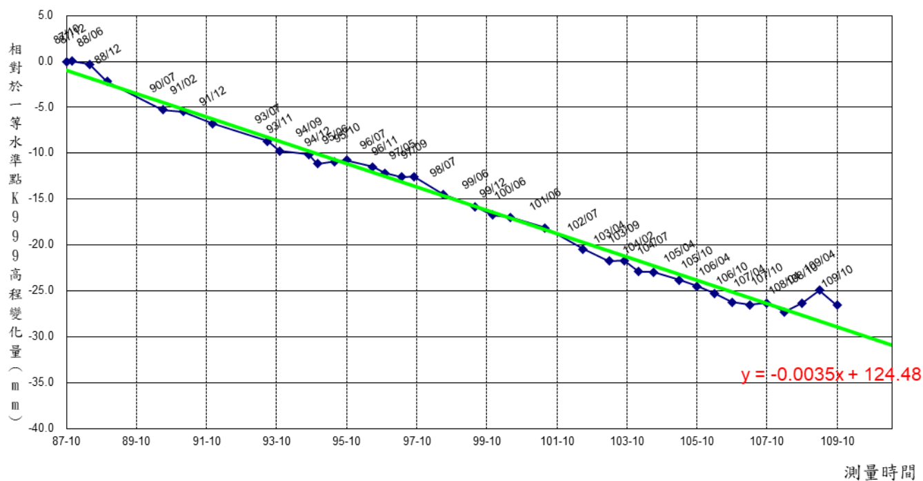
臺灣水準原點高程基準網K001水準點點位穩定性分析圖（毀損前）
