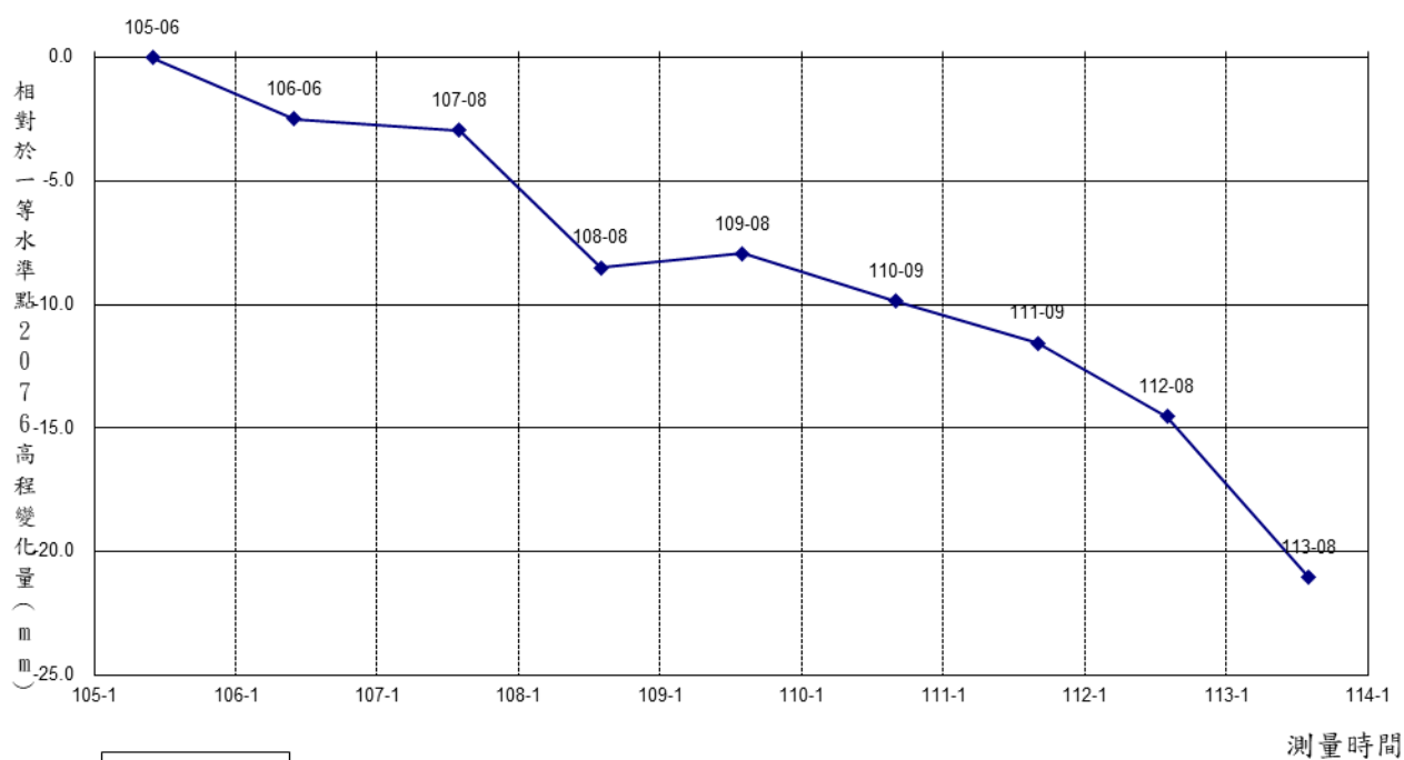
烏石潮位站水準點點位穩定性分析圖
