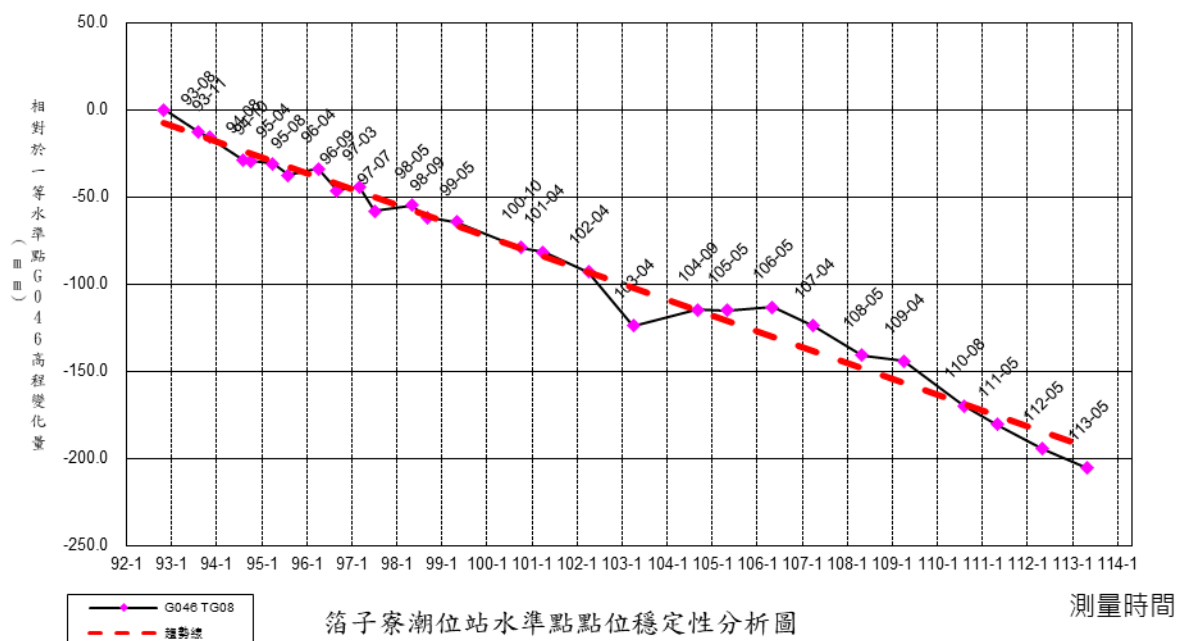
圖 5-5 箔子寮潮位站水準點 TG08 相對一等水準點 G046 之高程差變化圖
