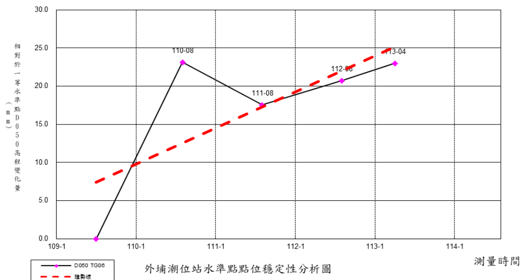
圖 5-18 外埔潮位站水準點 TG06C 相對一等水準點 D050 之高程差變化圖
