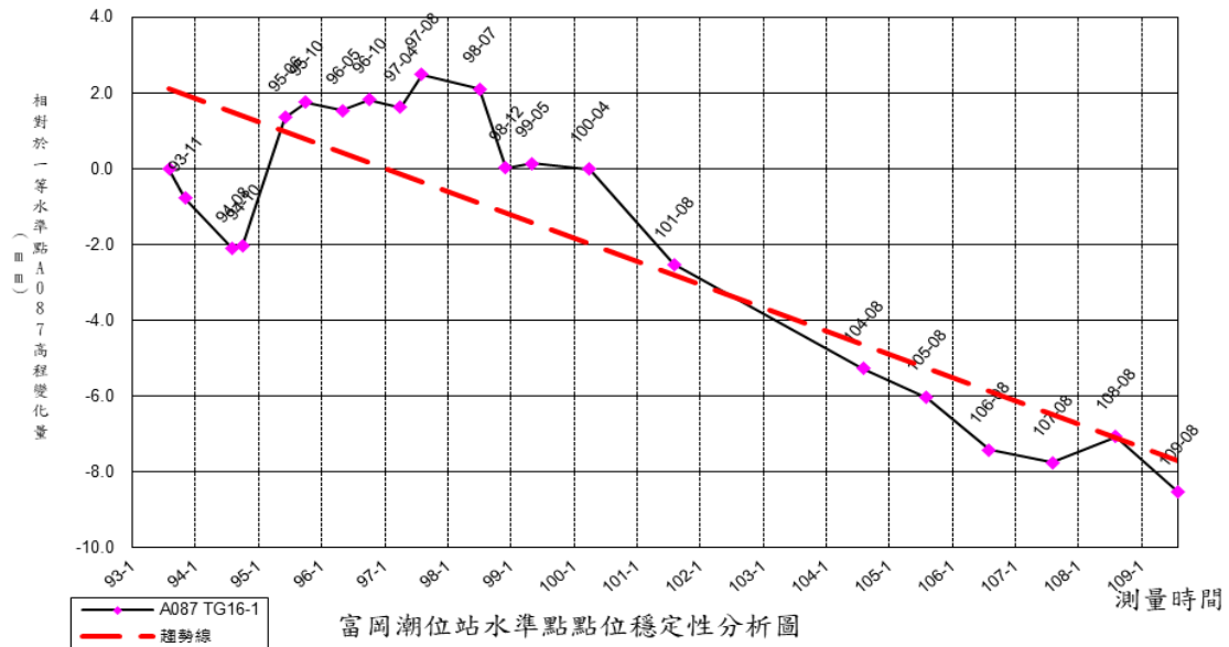
圖 5-19A 富岡潮位站水準點 TG16-1 相對一等水準點 A087 之高程差變化圖
