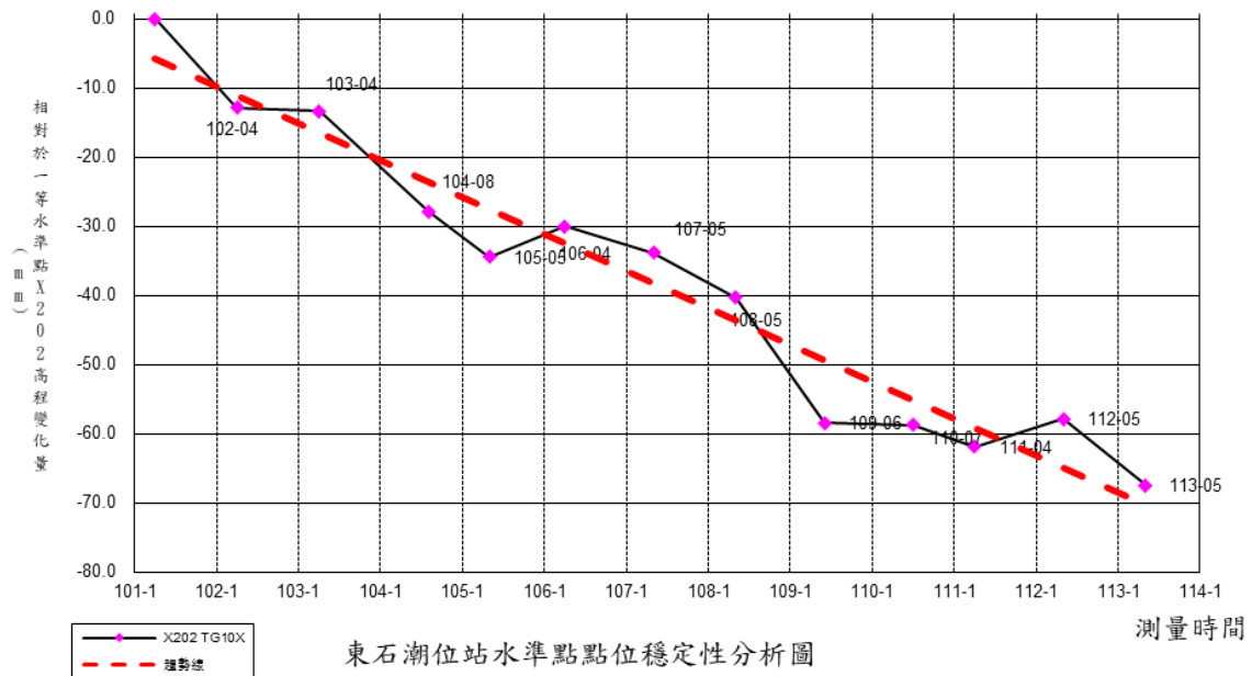
圖 5-7 東石潮位站水準點 TG10X 相對一等水準點 X202 之高程差變化圖
