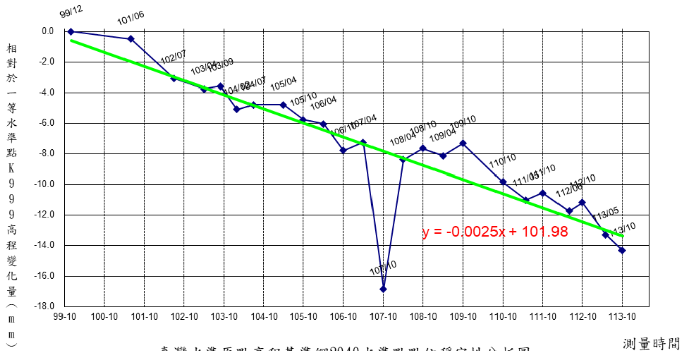
臺灣水準原點高程基準網2040水準點點位穩定性分析圖
