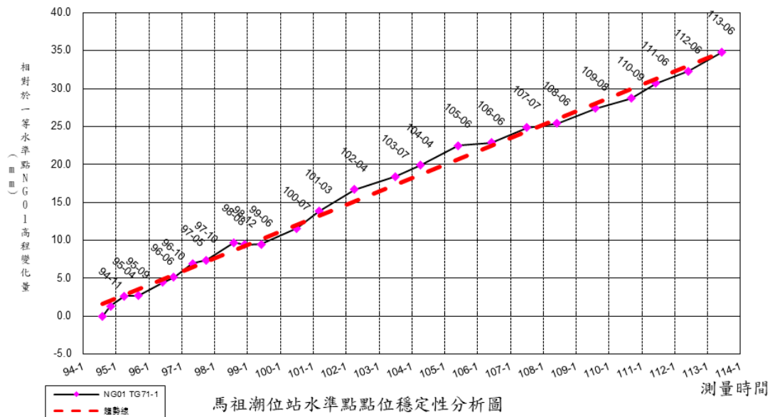
圖 5-13 馬祖潮位站水準點 TG71-1 相對一等水準點 NG01 之高程差變化圖
