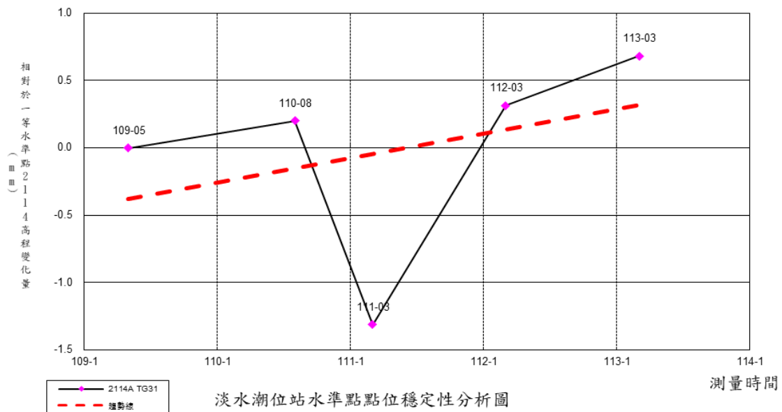
圖 5-21 淡水潮位站水準點 TG31 相對一等水準點 2114A 之高程差變化圖
