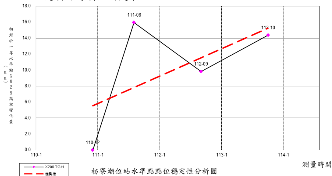
圖 5-24 枋寮潮位站水準點 TG41 相對水準點 X029 之高程差變化圖
