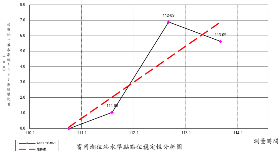
圖 5-19B 富岡潮位站水準點 TG16-1 相對一等水準點 A087 之高程差變化圖
