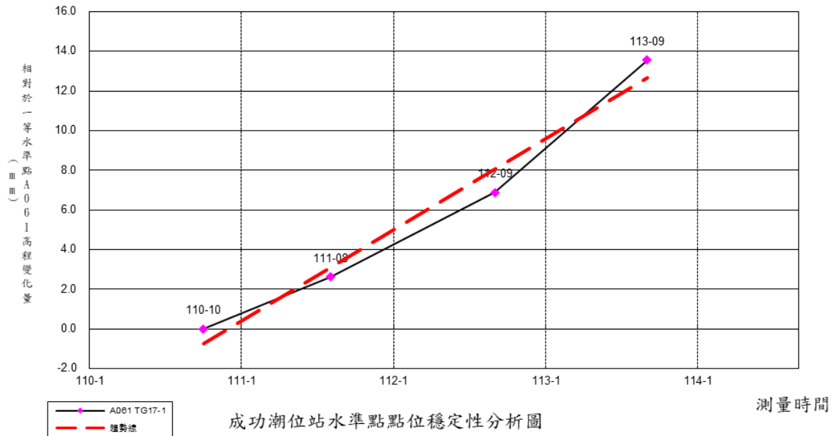
圖 5-20 成功潮位站水準點 TG78-1 相對水準點 A061 之高程差變化圖
