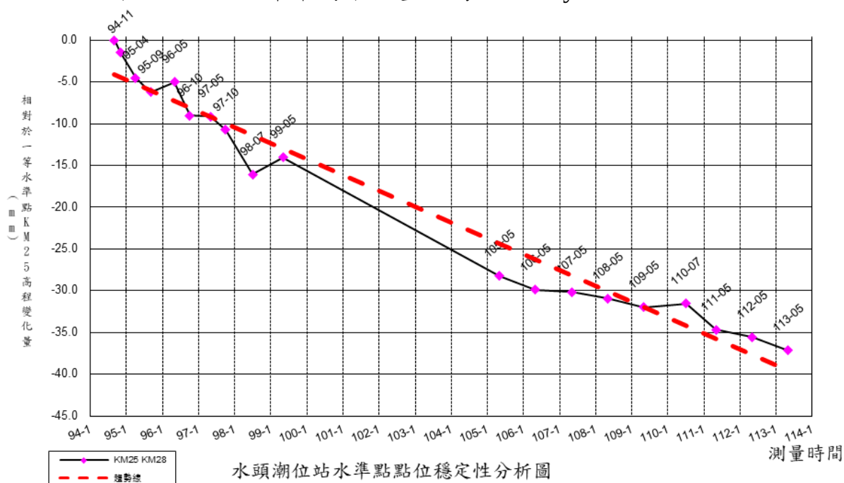
圖 5-9 水頭潮位站水準點 KM28 相對一等水準點 KM25 高程差變化圖
