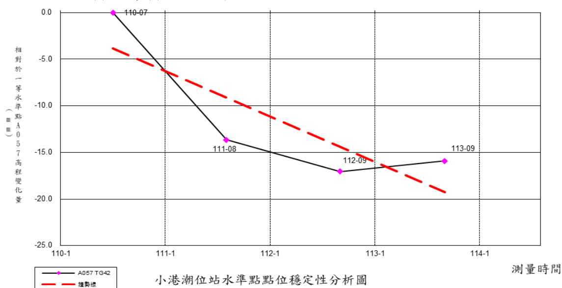
圖 5-25 小港潮位站水準點 TG42 相對水準點 CM01 之高程差變化圖
