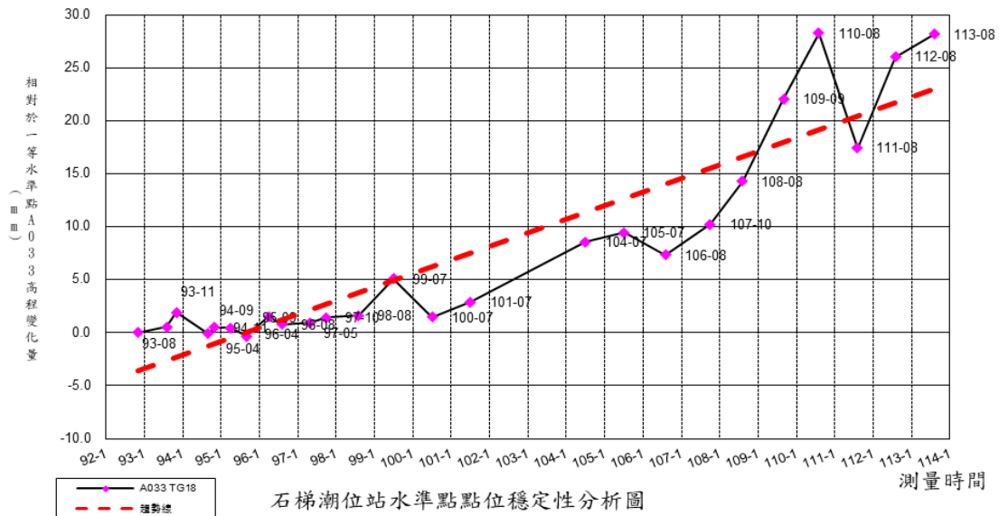
圖 5-11 石梯潮位站水準點 TG18 相對一等水準點 A033 之高程差變化圖
