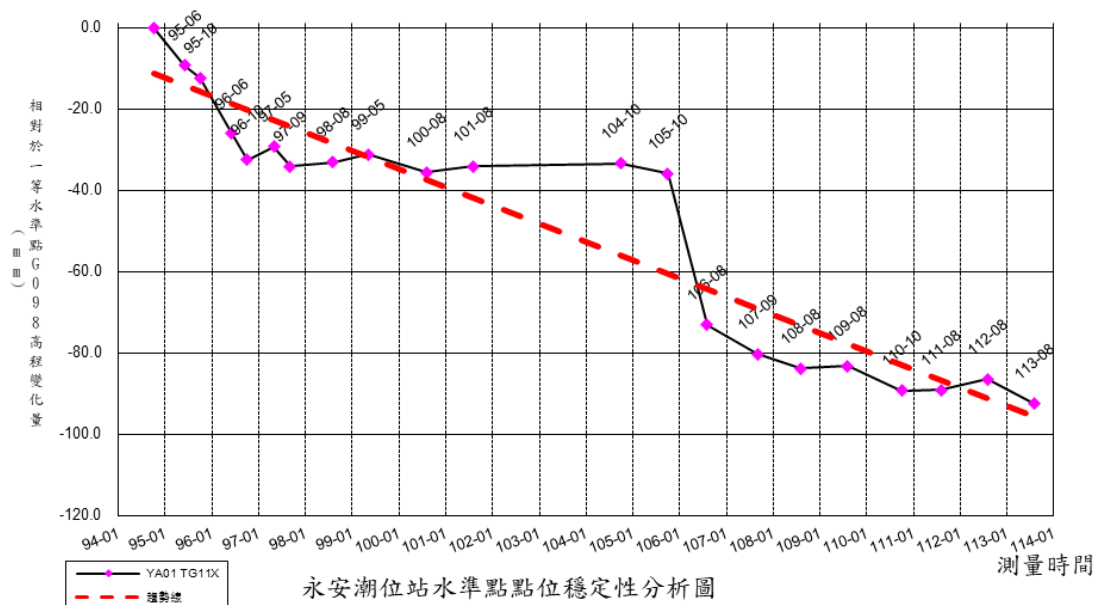
圖 5-8 永安潮位站水準點 TG11X 相對一等水準點 YA01 之高程差變化圖
