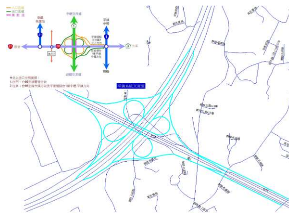
(b) 平鎮系統交流道(國 1-台 66)_不同道路等級，故等級高優先
