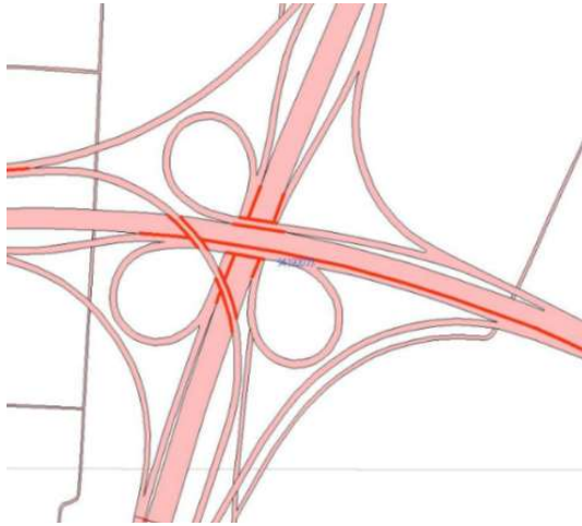
圖 25、多重立體交叉道路示意_使用道路 分隔線區隔
