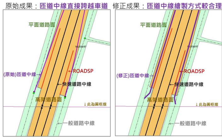
圖 6、匝道路口處之道路中線交會方式繪製範例
