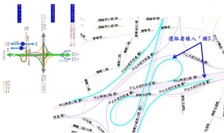
(a) 汐止系統交流道(國 1-國 3)_相同道路等級，按車流起迄方向紀錄編號
