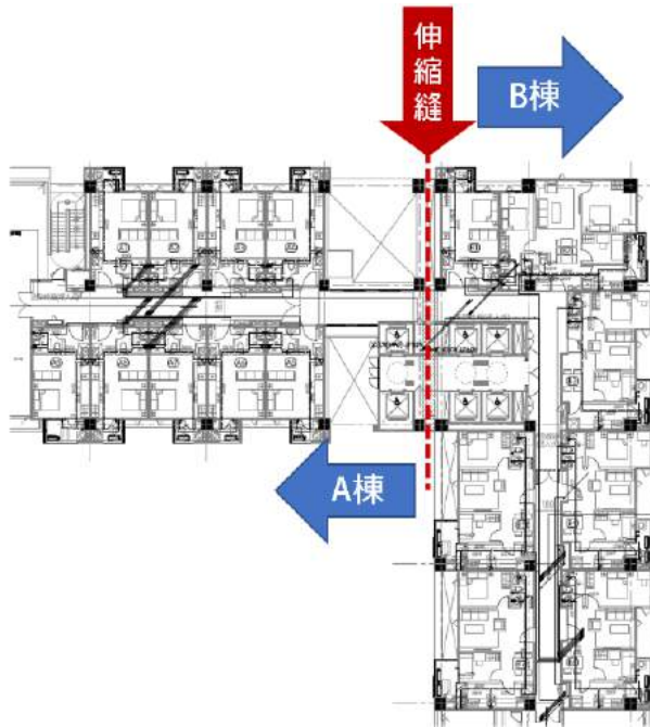
圖 16 有伸縮縫設計之建築物應分兩棟來執行碳排評估
