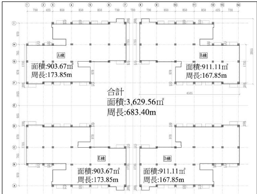
圖 6 平面形狀係數 f_1 參數檢討圖
