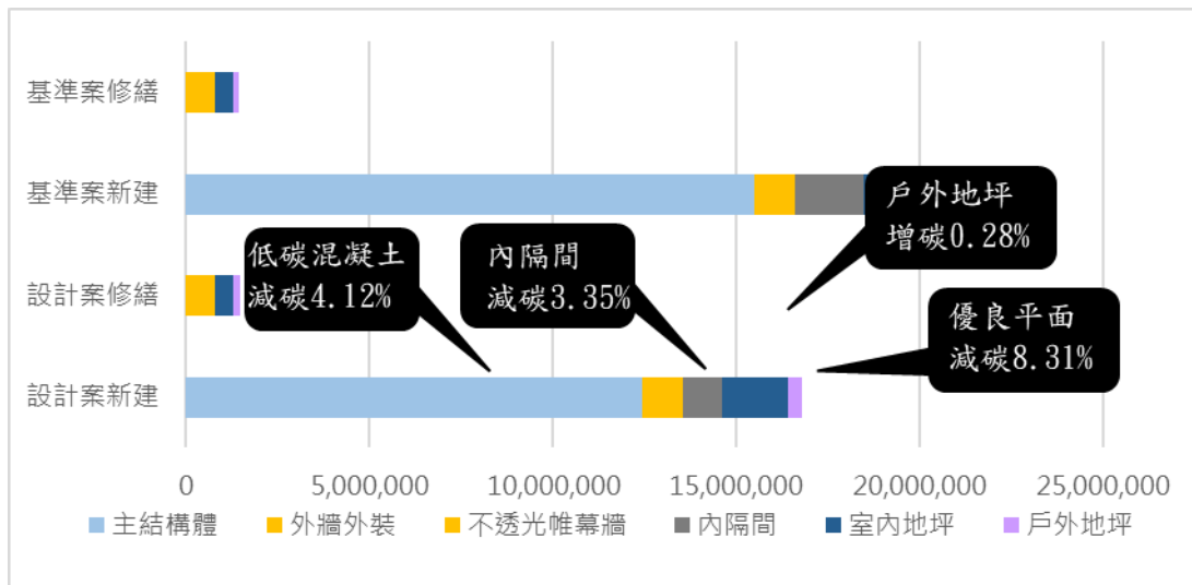
圖 14 資料製造運輸之各項減碳設計 ΔCF 貢獻度分析
