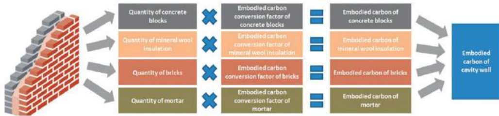
圖 15 RICS 建議以建築設計圖說來計算構件碳排的方法（RICS，2012）
