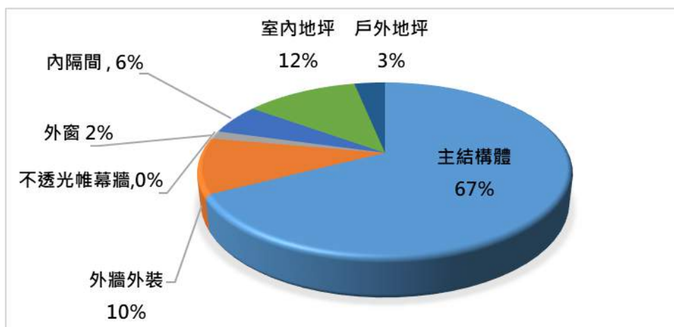
圖 11 設計案資材碳排佔比百分比圖（新建+修繕）
