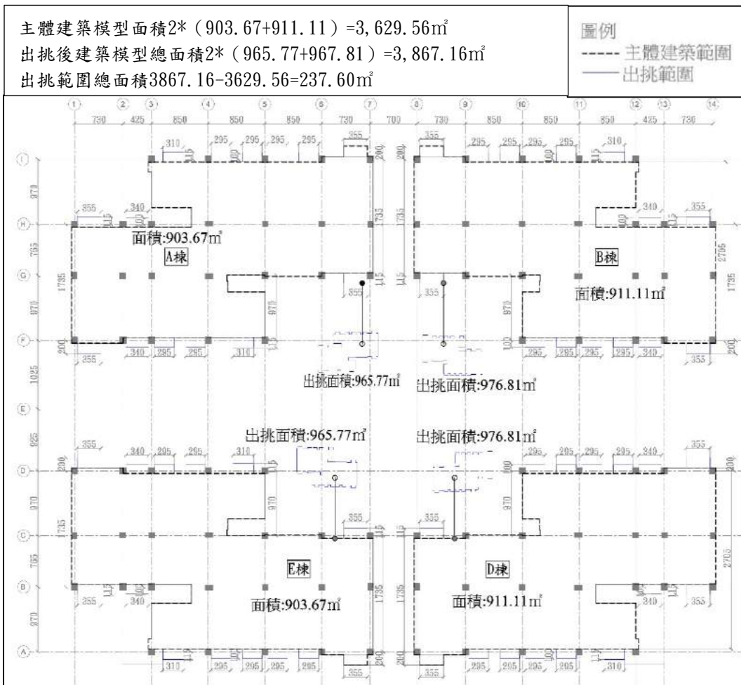
圖 8 平面形狀係數 f_3 參數檢討圖
