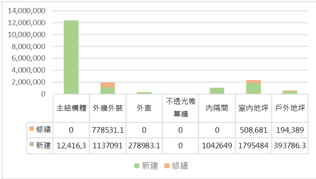
圖 12 分項工程新建與修繕碳排量比較圖
