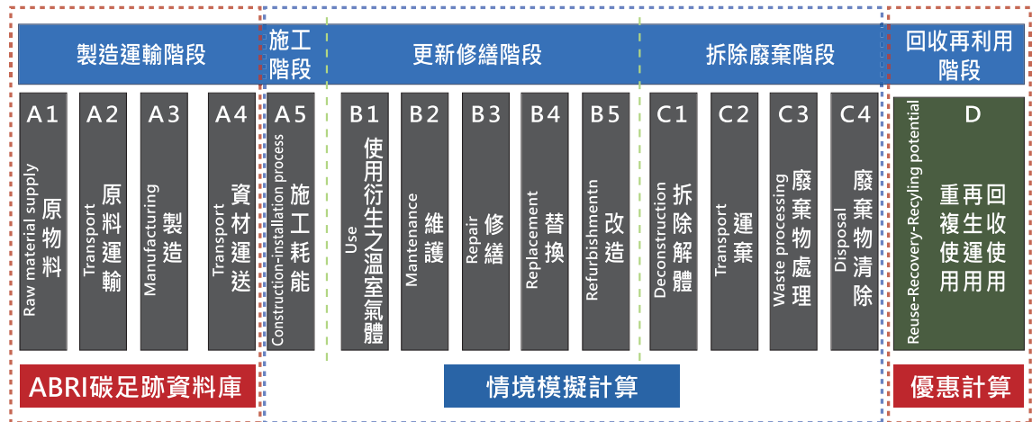
圖 13 低碳建築評估系統 LEBCR 方法論概要 (改繪自 EN15978 (2011))
