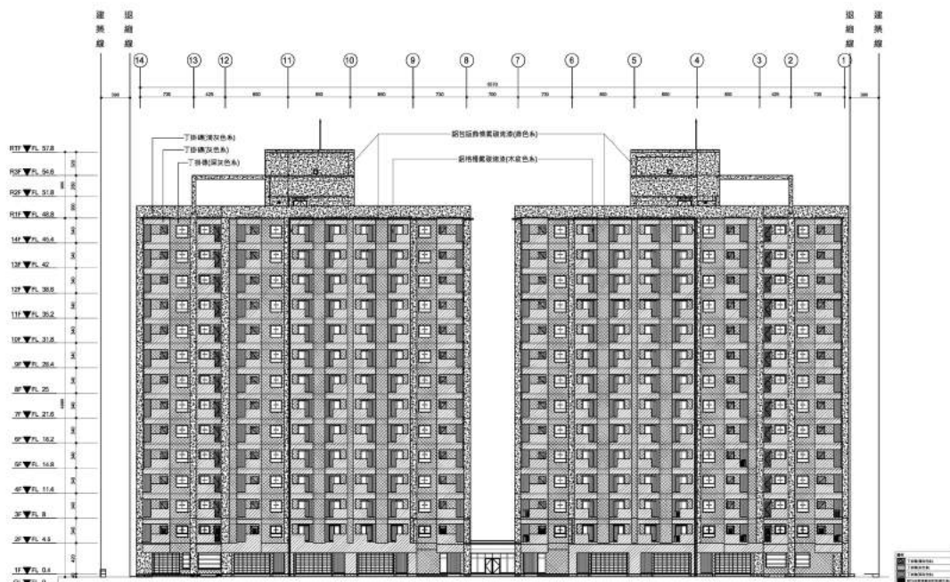
圖 2 北向立面圖
