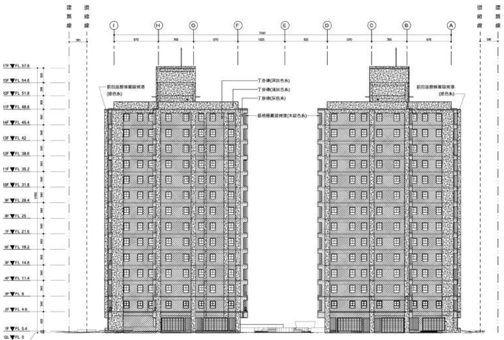
圖 3 東向立面圖
