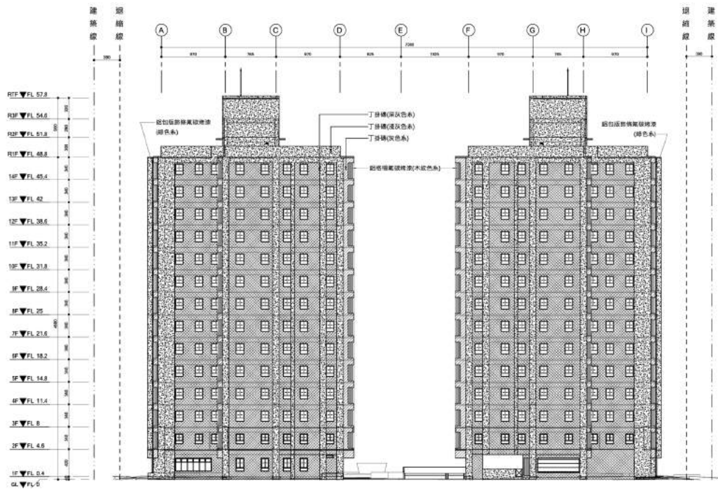
圖 4 西向立面圖
