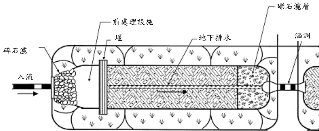
(a) 俯視圖
