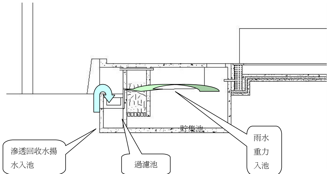
圖 2-14 設置滲透管溝將透水鋪面下的水回收
