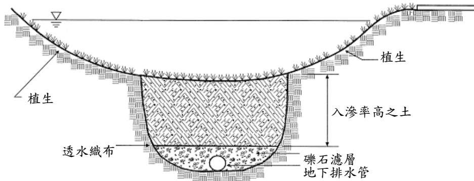
(b) 剖面圖
