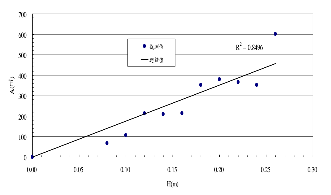
圖 5-28 滲透陰井（直徑 50 cm、開孔率 0.708%） A_{us} 與 H 關係圖
