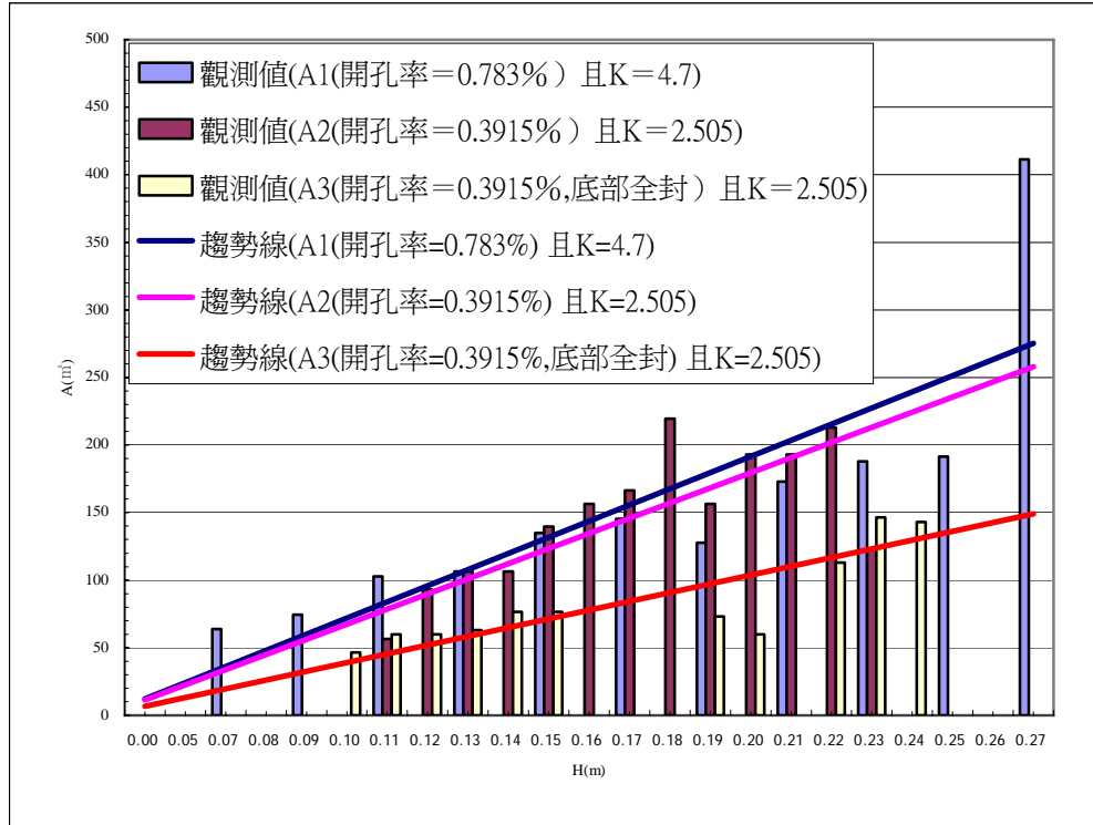
圖 5-33 滲透陰井(直徑 40 cm)觀測值與推估值 A_{us} 與 H 關係圖
