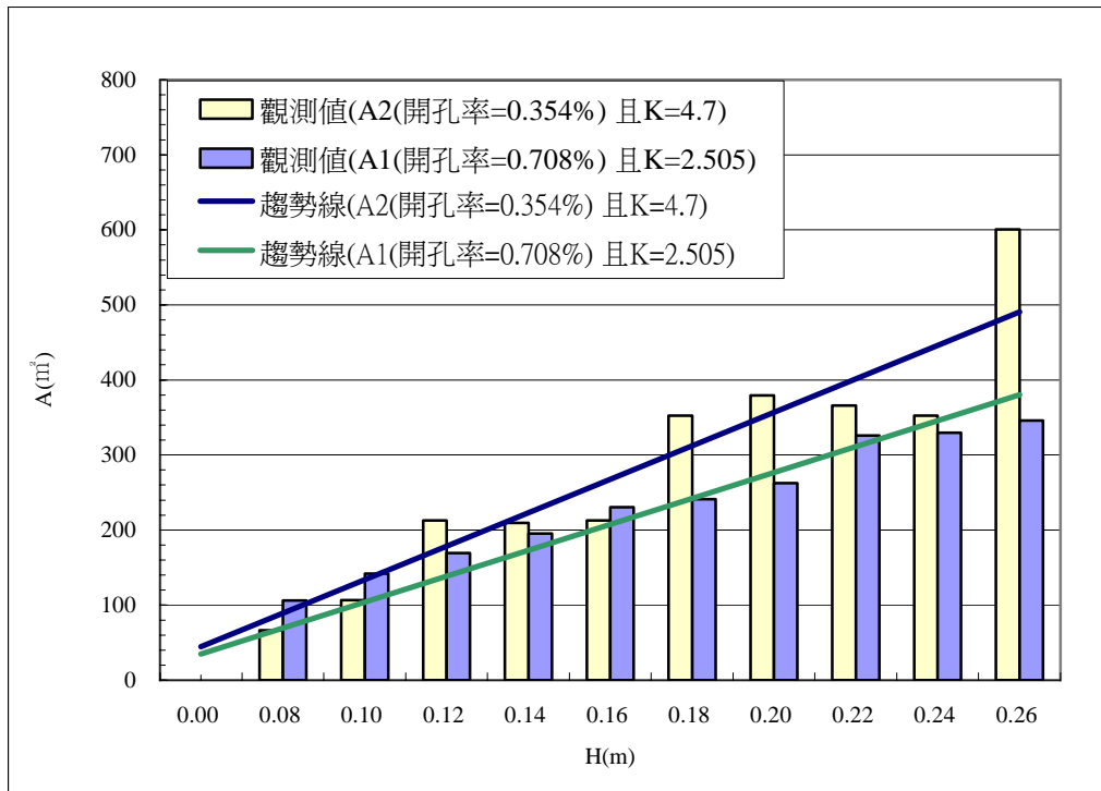
圖 5-32 滲透陰井(直徑 50 cm)觀測值與推估值 A_{us} 與 H 關係圖
