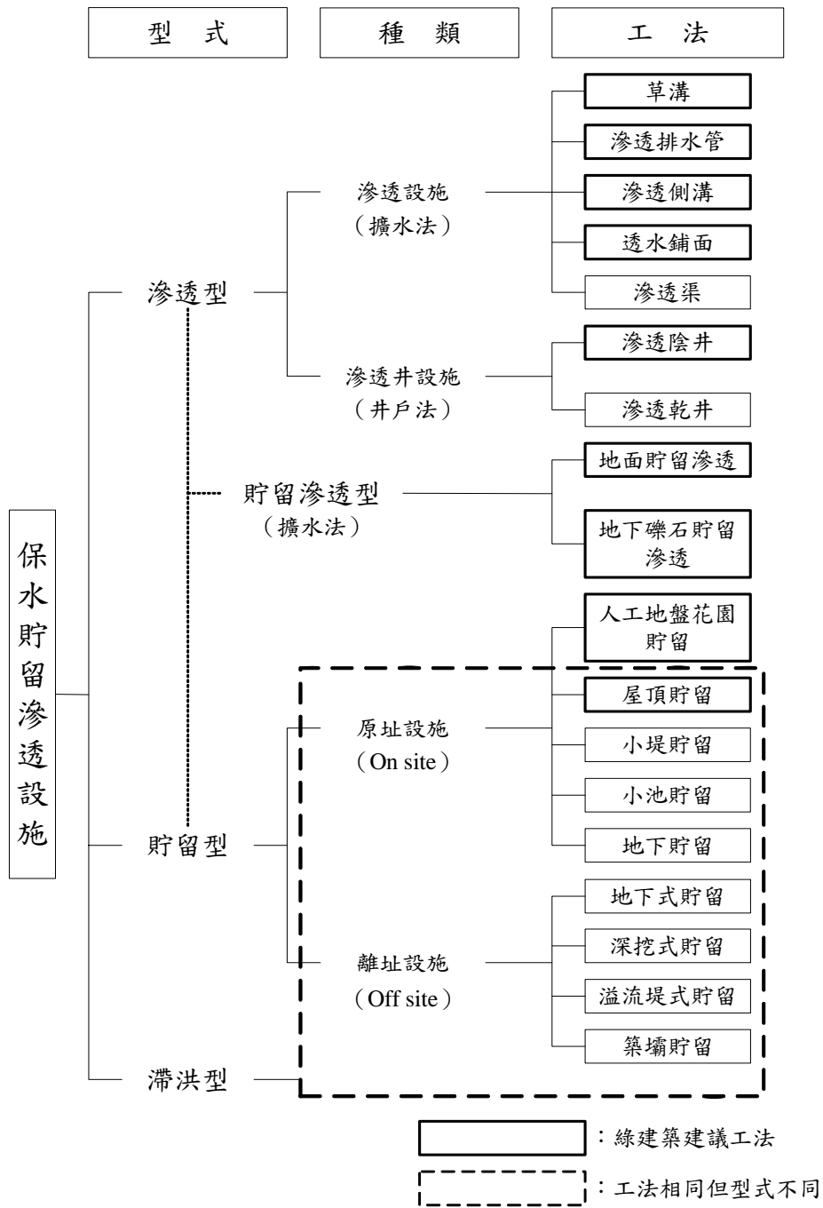
圖 2-9 水貯留及滲透設施分類示意圖
