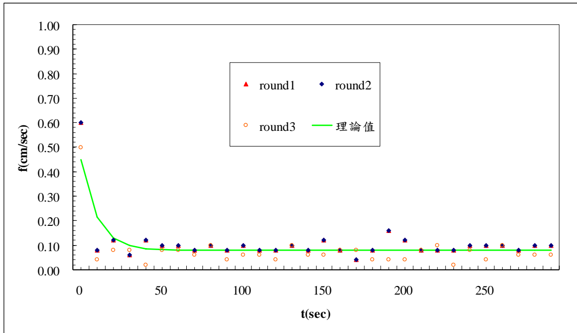
圖 5-13 試驗孔葛洛夫滲透儀觀測入滲曲線
