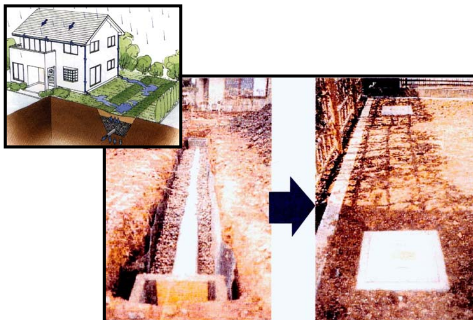
圖 2-11 日本滲透側溝設置實例
