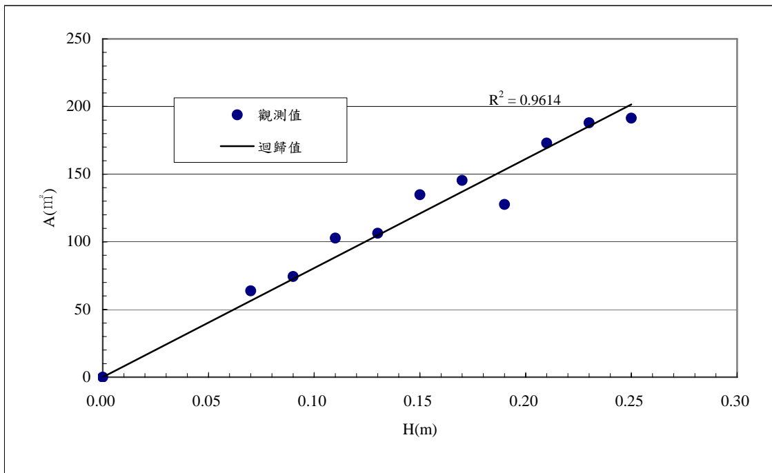
圖 5-25 滲透陰井（直徑 40 cm、開孔率 0.783%） A_{us} 與 H 關係圖
