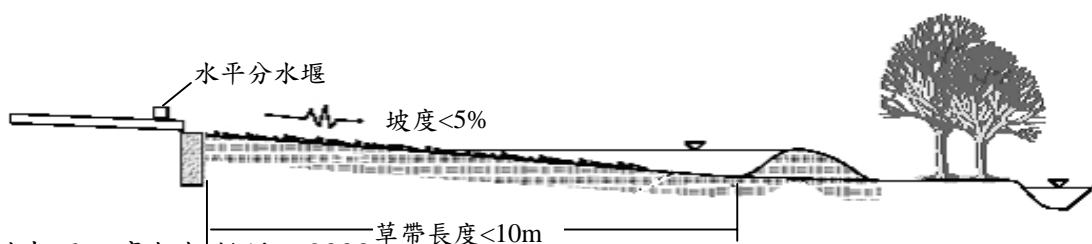
圖 3-4 草帶構造示意圖
