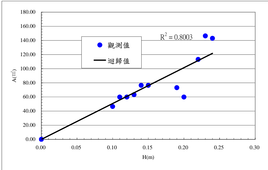
圖 5-27 滲透陰井 (直徑 40 cm、開孔率 0.39125%，底部全封) A_{us} 與 H 關係圖
