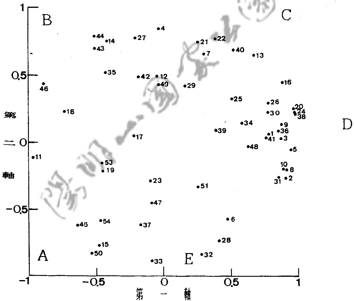
圖九、下層各型植物社會與覆被植物在PCA前二軸所成平面之分布圖
