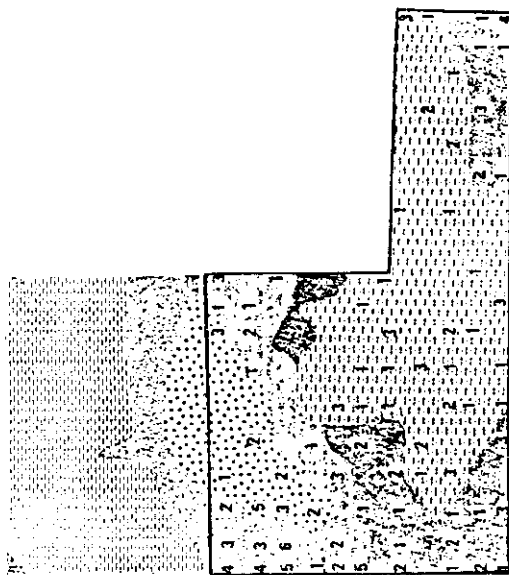
圖二十、樹林中捕獲赤腹松鼠之位置與多次示意圖 (自1989年1月至12月)
