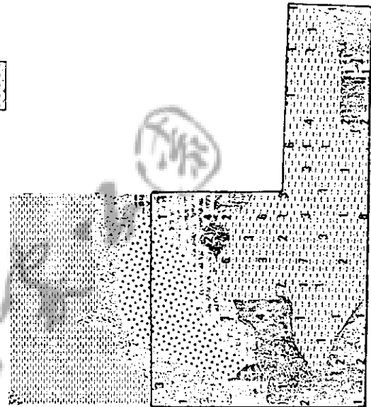
圖二十一、樹林中捕獲刺鼠之位置與多次示意圖 (自1989年1月至12月)
