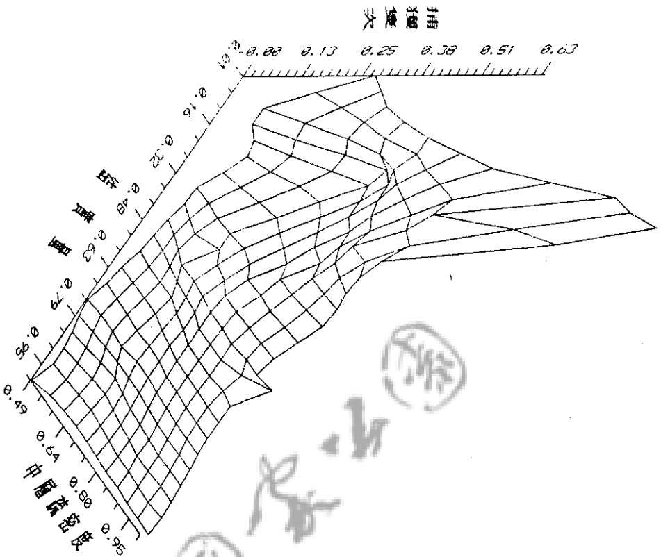
圖二十四、各型植物社會相對結實量、中層植物密度與赤松鼠捕獲隻次之關係 (數據來自西北坡A、B、C、D型, 自1989年1月至12月)
