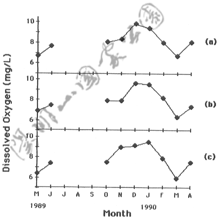
圖 7.1、翠翠谷流水部份水中溶氧量之月變化圖。 (a:上游 b:中游 c:下游)
