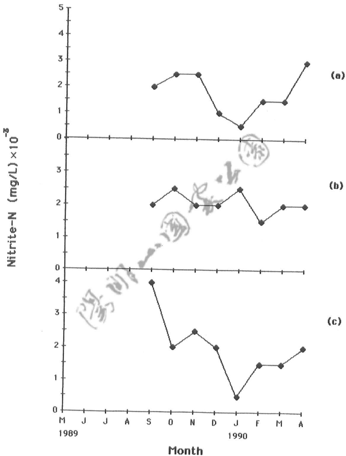
圖10.1、翠翠谷流水部份水中含亞硝酸氮濃度之月變化圖。 (a:上游 b:中游 c:下游)
