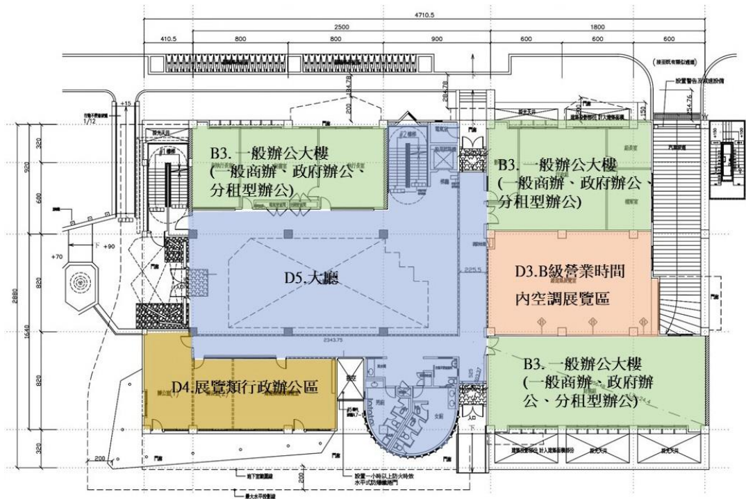
圖 B 一層平面圖
