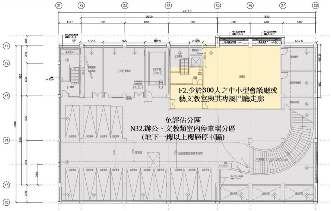
圖 A 地下一層平面圖
