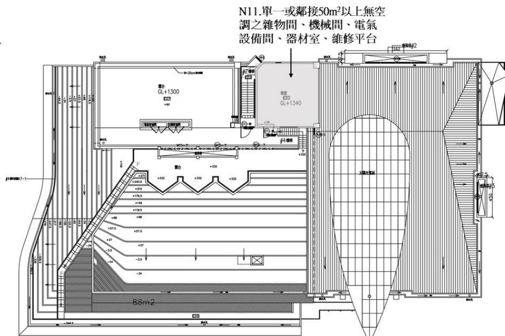
圖 F 屋凸平面圖
