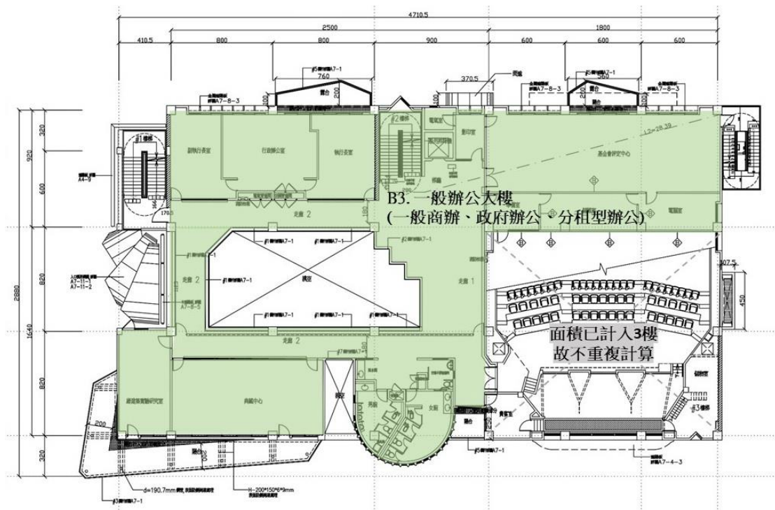
圖 D 三層平面圖
