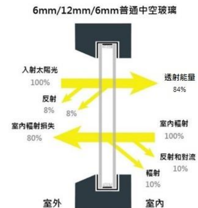
圖 7-26 複層玻璃之玻璃參數示意圖
