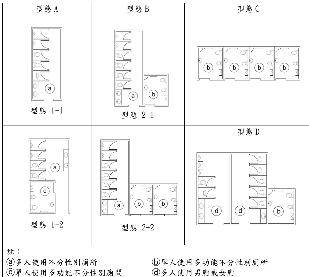
圖 2-7 不分性別廁所建議型態(資料來源：性別友善廁所設計手冊之研究，2016)
