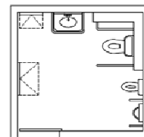
平面圖 B (有設小便器)
