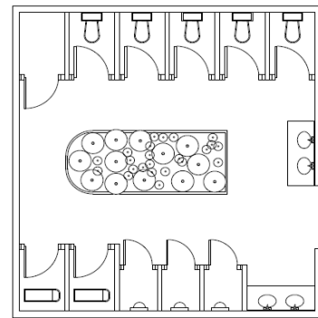
平面圖 3 (小便器隔間式+景觀花台)
