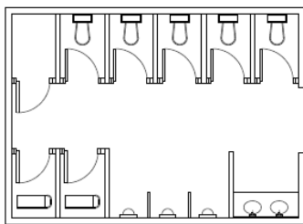
平面圖 1 (小便器開放式)
