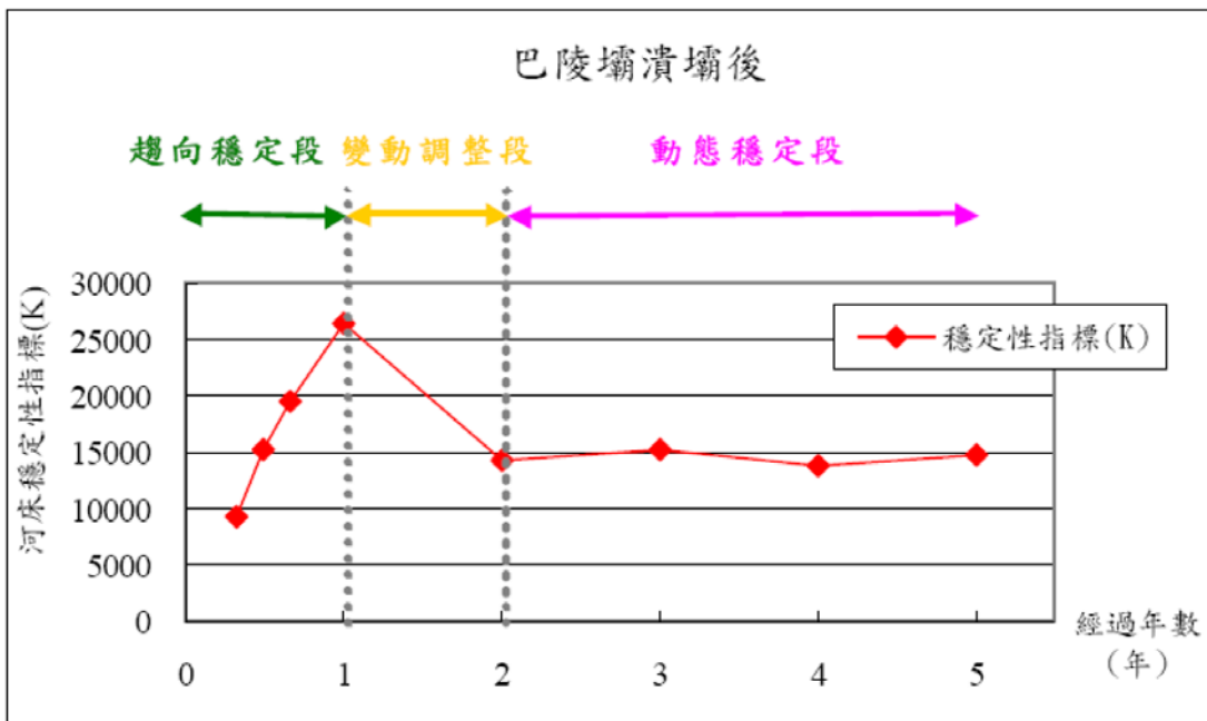
圖 3-12 巴陵壩潰壩後-穩定性指標(K)與經過年數之關係圖
