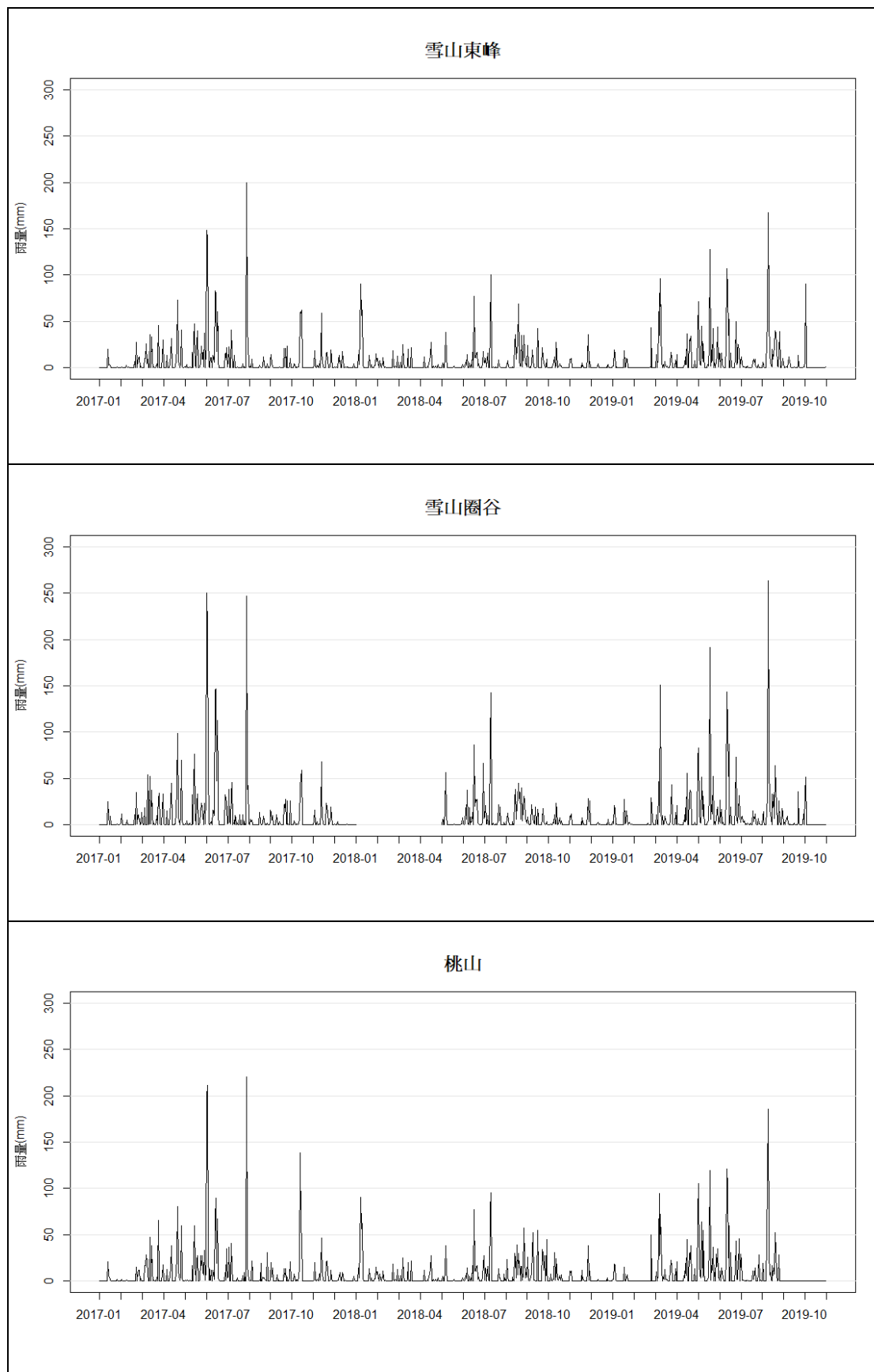
圖 4-5 七家灣溪集水區中央氣象局氣象站日雨量(2017 年至 2019 年)
