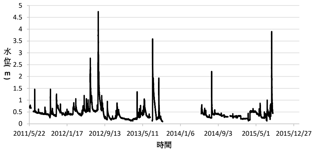
圖 4-10 萬壽橋水位測站之時水位資料
