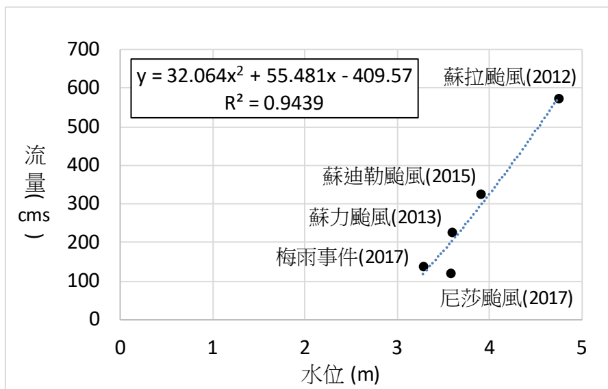
圖 5-20 2011-2019 年各事件尖峰流量-水位率定曲線圖
