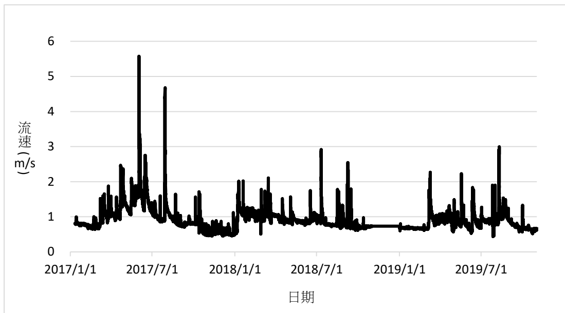
圖 5-7 萬壽橋水文測站-流速
