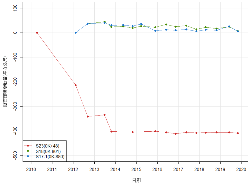
圖 5-15 斷面面積變動量 (縱軸正向代表淤積；負向代表冲刷)
