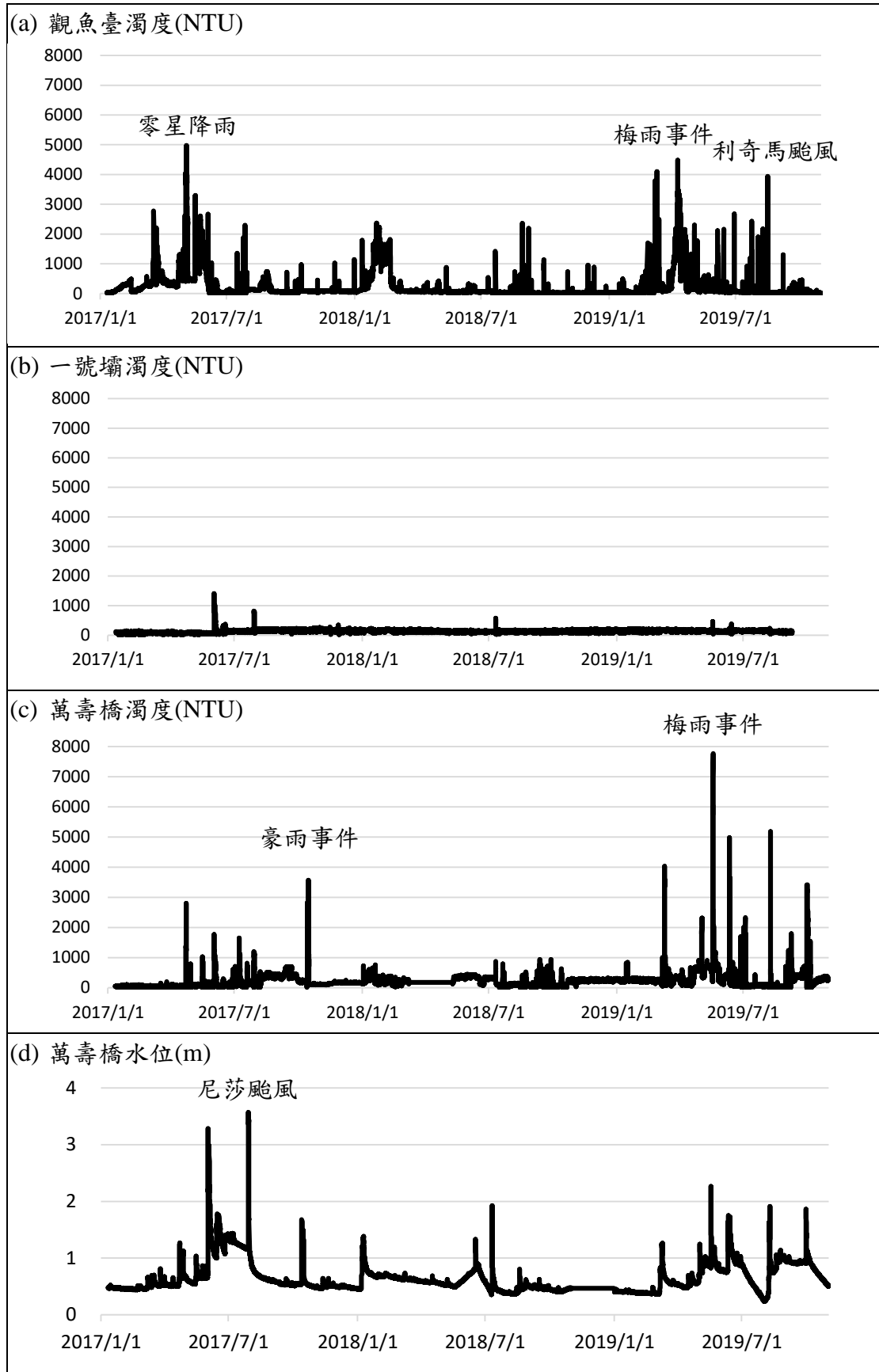
圖 5-8 水文測站濁度(a)觀魚臺、(b)一號壩、(c)萬壽橋與(d)萬壽橋水位
