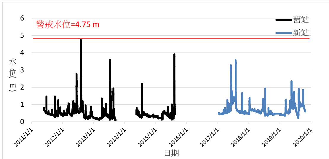
圖 5-5 萬壽橋水文測站-水位
