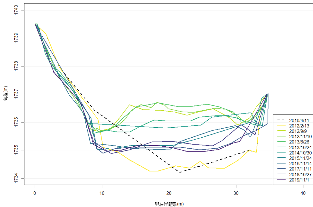
圖 5-13 S18 斷面(OK-801)
