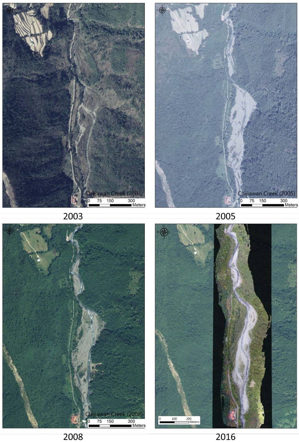
圖 4-12 七家灣溪歷年航照圖(2/3)
