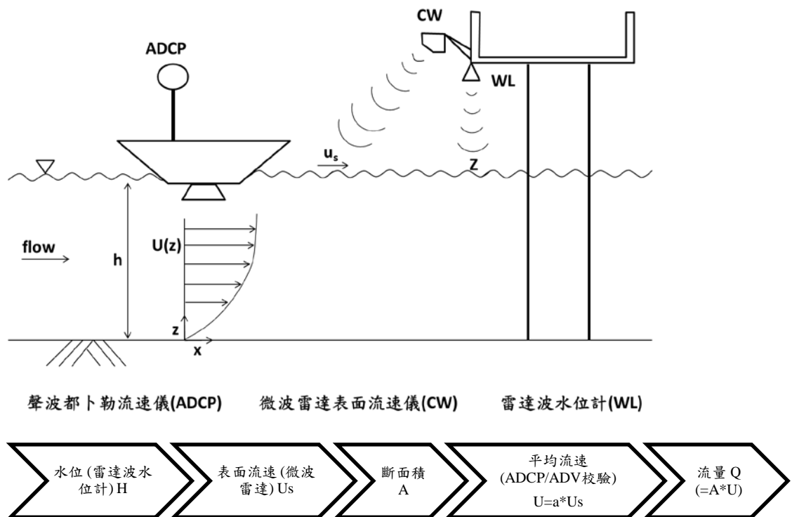
圖 5-18 流量推估流程
