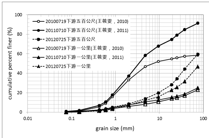
圖 4-18 七家灣溪一號壩明坑挖掘下游各區粒徑級配比較圖
