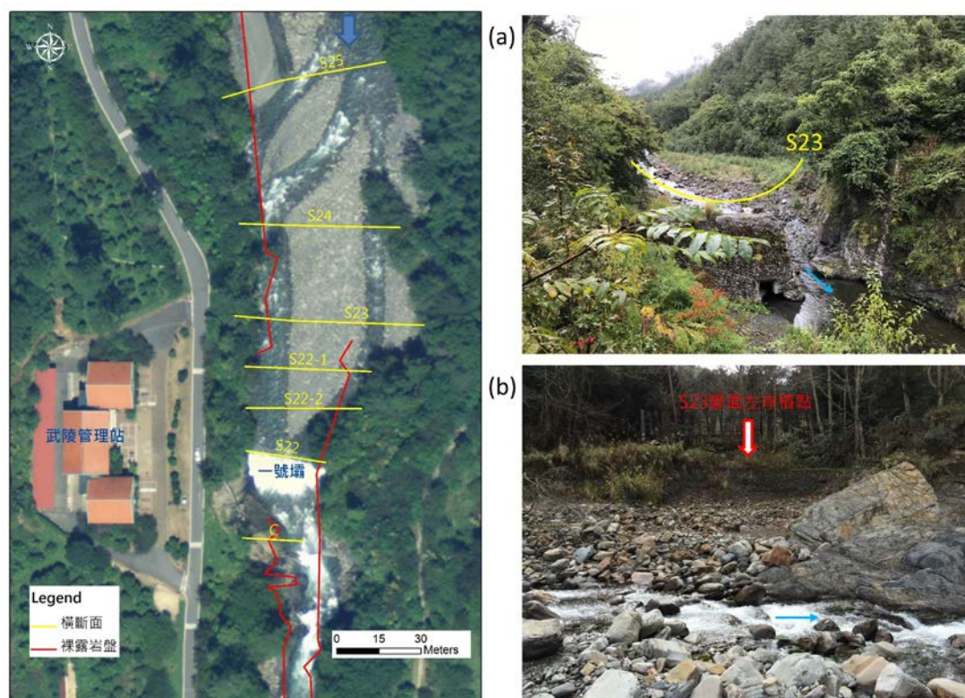
圖 5-9 一號壩河道環境 (航照底圖為農林航空測量所於 2008 年 9 月 21 日拍攝；現場照片為本研究於 2018 年 10 月 18 日(a)及 2015 年 1 月 28 日(b)拍攝)
