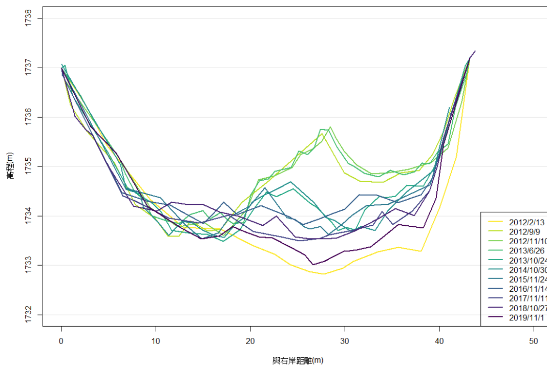
圖 5-14 S17-1 斷面(OK-880)
