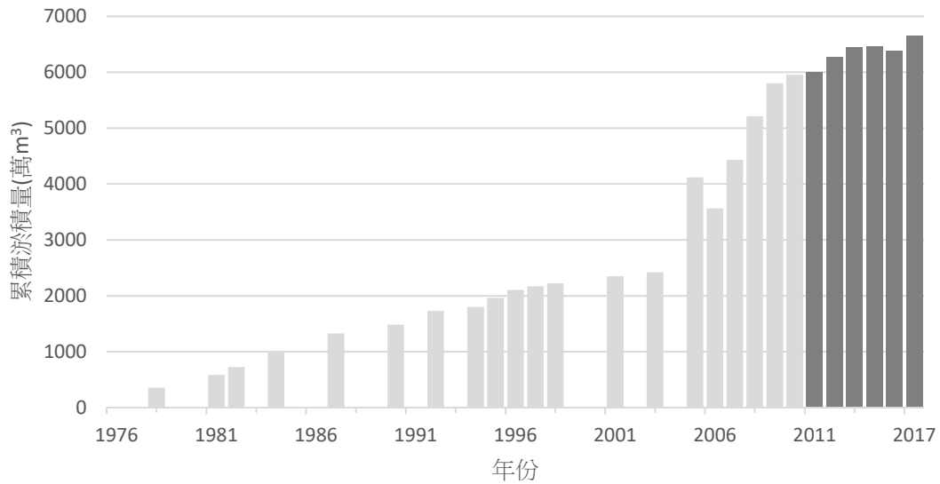
圖 6-3 德基水庫歷年累積淤積量
