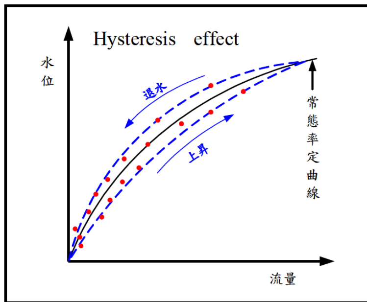
圖 5-17 洪水期間水位-流量之遲滯現象示意圖
