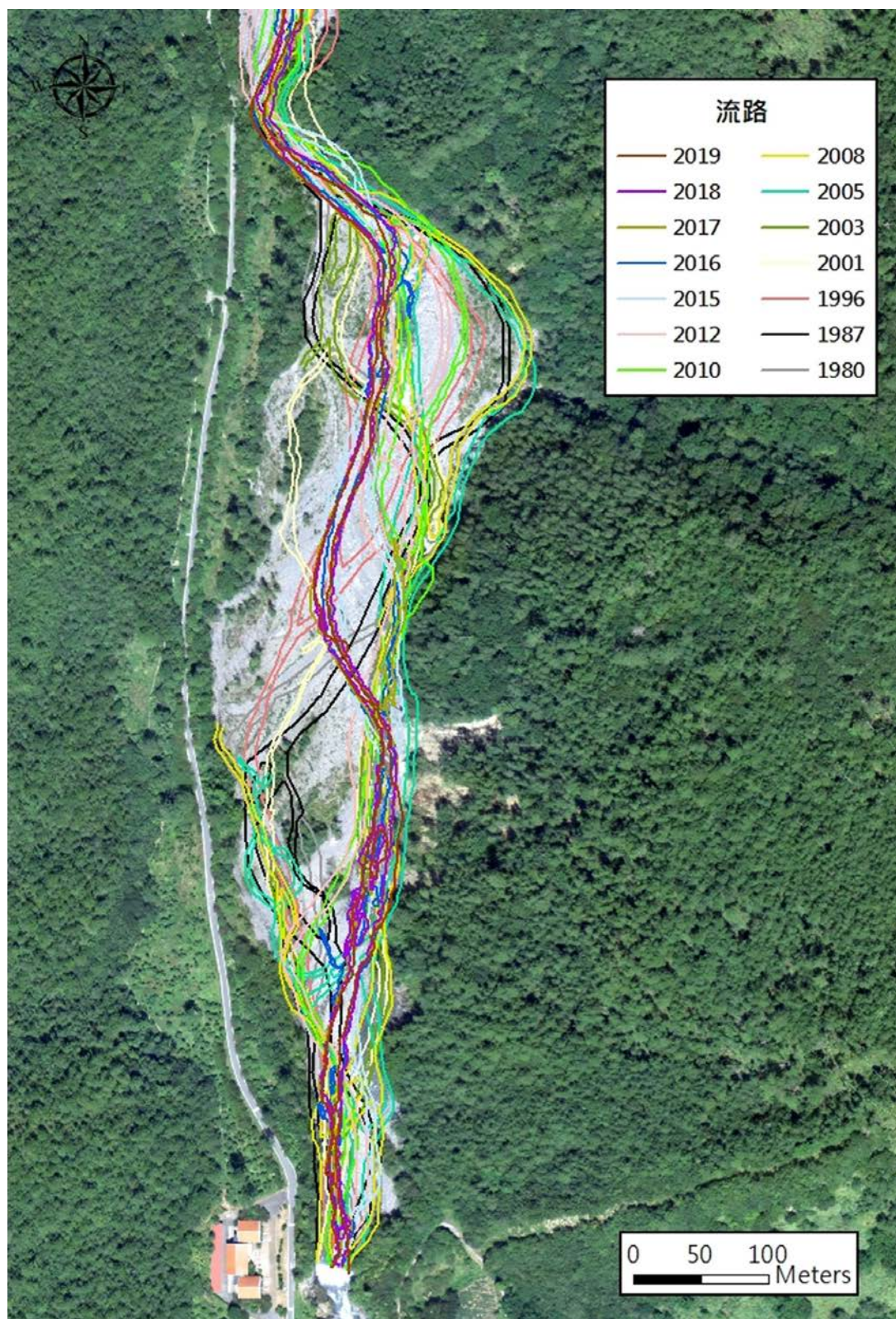
圖 5-21 一號壩上游河道歷年比較
