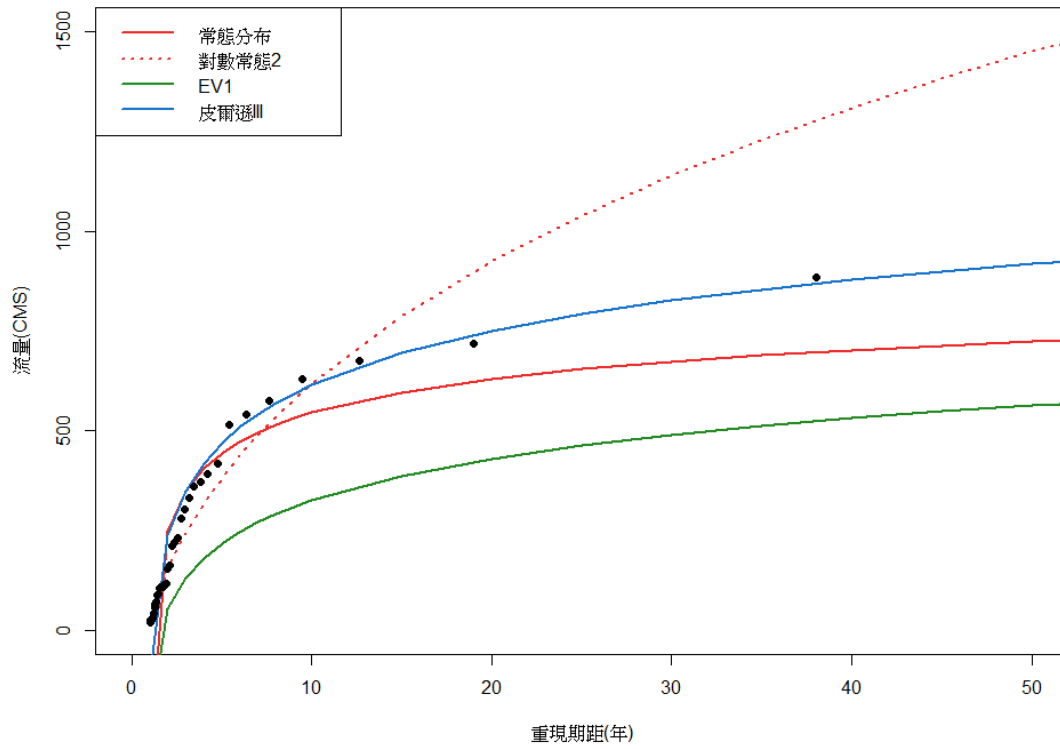
圖 4-7 七家灣測站流量頻率分析結果
