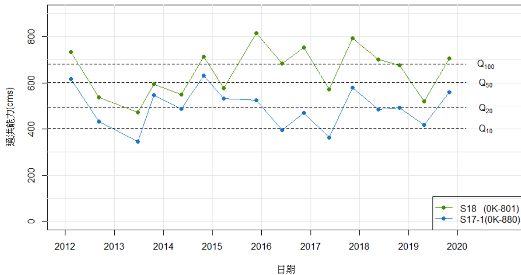
圖 5-16 斷面基本通洪能力
