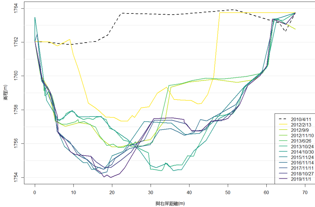
圖 5-12 S23 斷面(OK+48)
