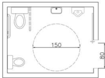
獨立式多功能廁所空間尺寸
