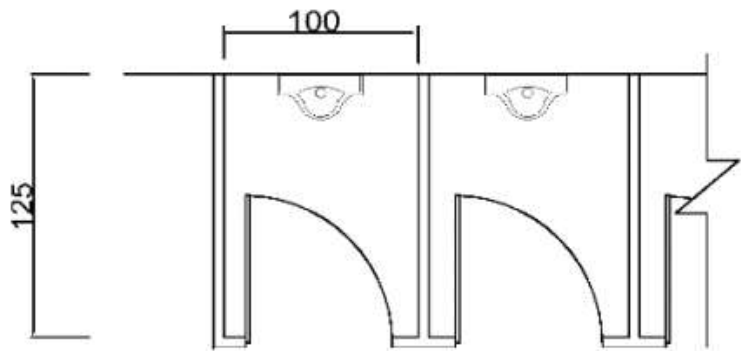
小便器廁間空間尺寸
