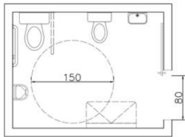
小便器廁間空間尺寸
