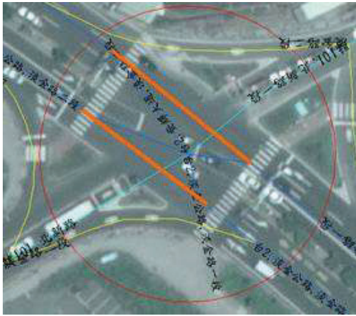
圖 14、交叉路口前後之道路中線數量對等_井字接法 圖 15、交叉路口前後之道路中線數量不對等_米字接法
