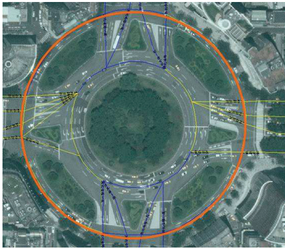
圖 17、圓環數化原則與標註方式
