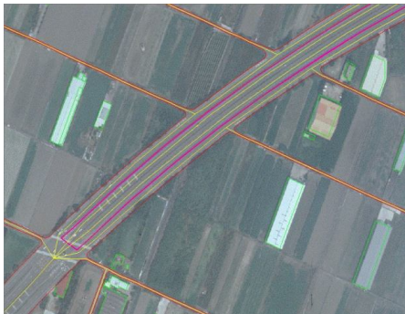
圖 7、高速公路中線繪製圖
