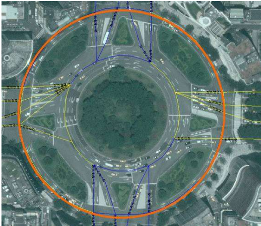
圖 16、圓環數化原則與標註方式
