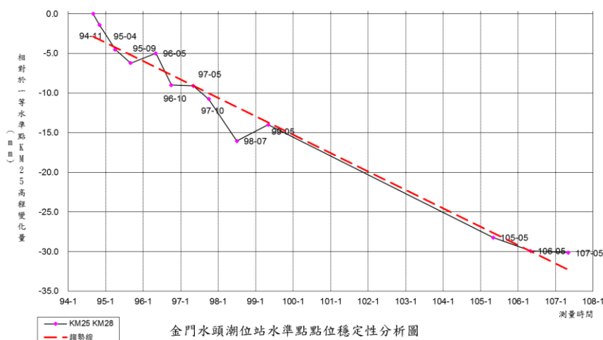
圖 5-8 金門水頭潮位站水準點 KM28 相對一等水準點 KM25 高程差變化圖
