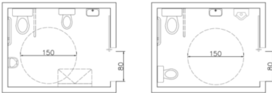
獨立式多功能廁所空間尺寸
