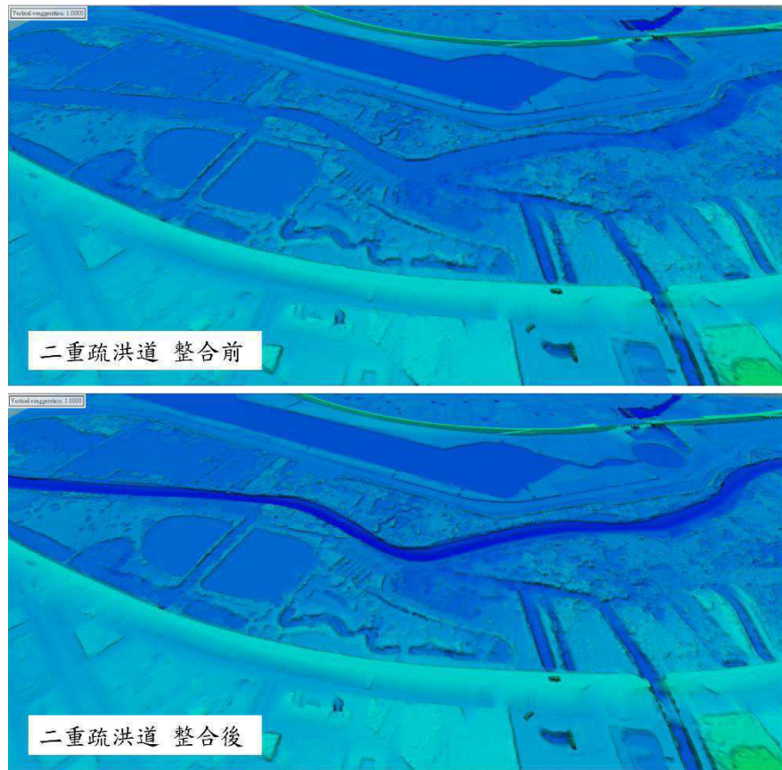
圖 2-63 二重疏洪道断面與 HyDEM 網格整合前後比較示意圖
