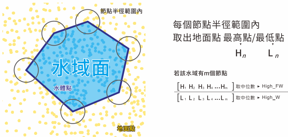
圖 2-31 指引規定之水域高程賦予方法
