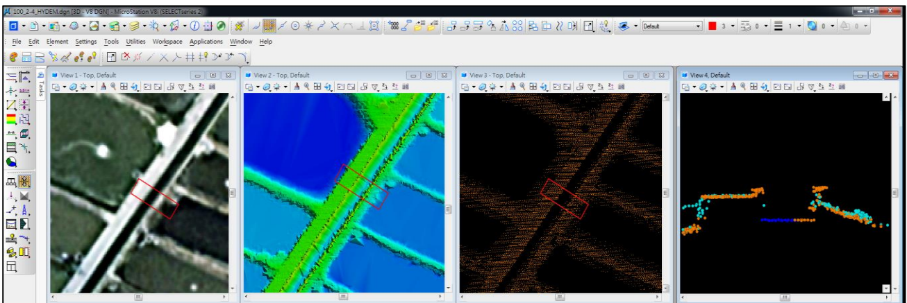
圖 2-8 水利數值地形模型點雲分類作業畫面
