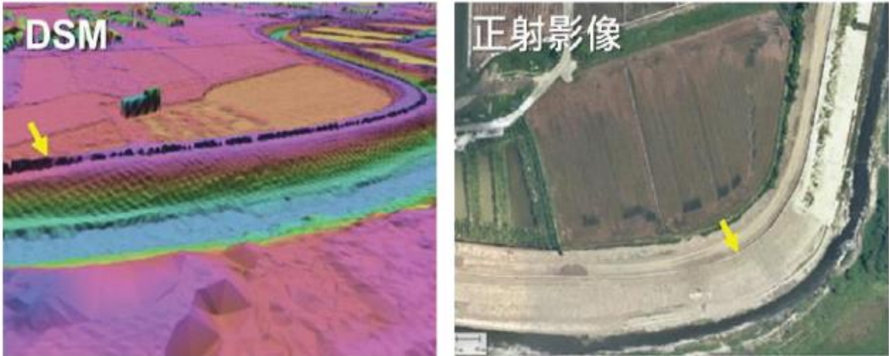
圖 2-10 寬度小於 1 公尺之人工組水構造物於 DSM 與正射影像上表示
