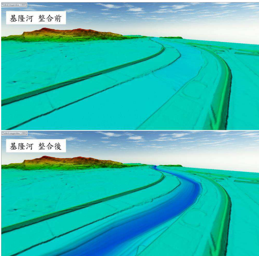
圖 2-59 基隆河河川斷面與 HyDEM 網格整合前後比較示意圖
