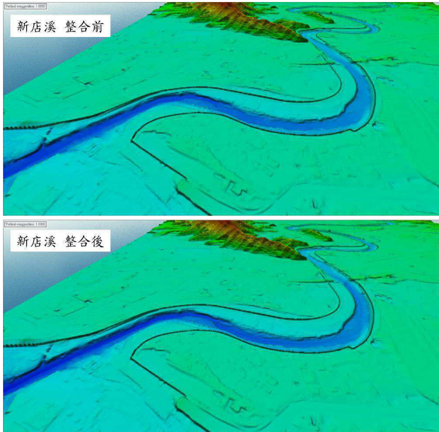
圖 2-62 景美溪河川断面與 HyDEM 網格整合前後比較示意圖
