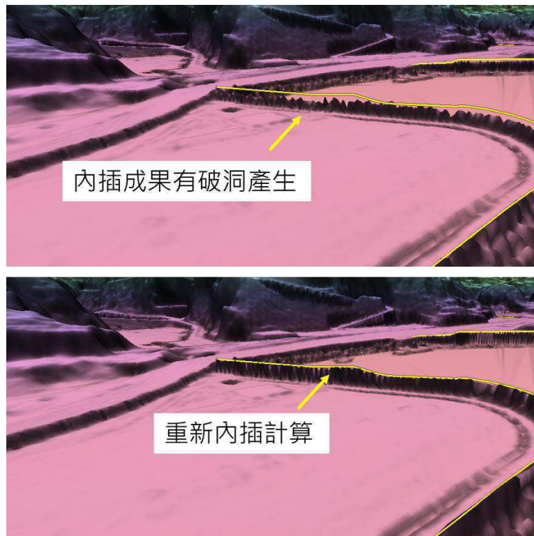
圖 2-45 重新內插計算小於 1 公尺寬度之阻水人工構造物
