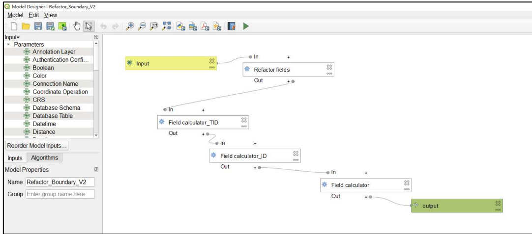
圖 3-9 三維水利圖徵屬性表檢查
