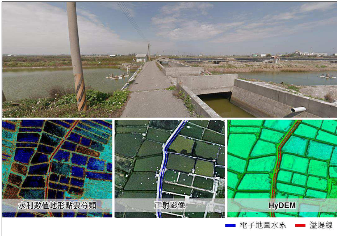
圖 2-19 溢堤線繪製原則：可以判斷渠道流通性
