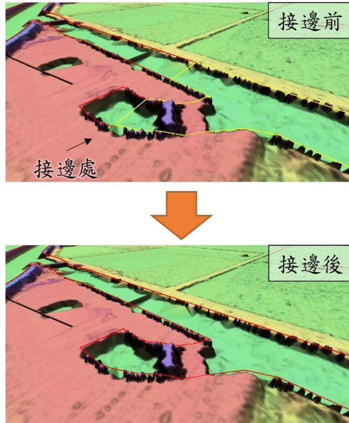
圖 2-43 圖徵接邊處理示意圖 (紅黃線為不同圖幅)
