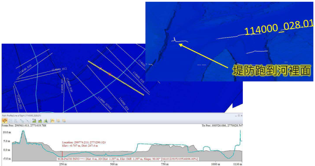
圖 2-54 淡水河断面編號 114000_028.01 無法與光達資料做整合
