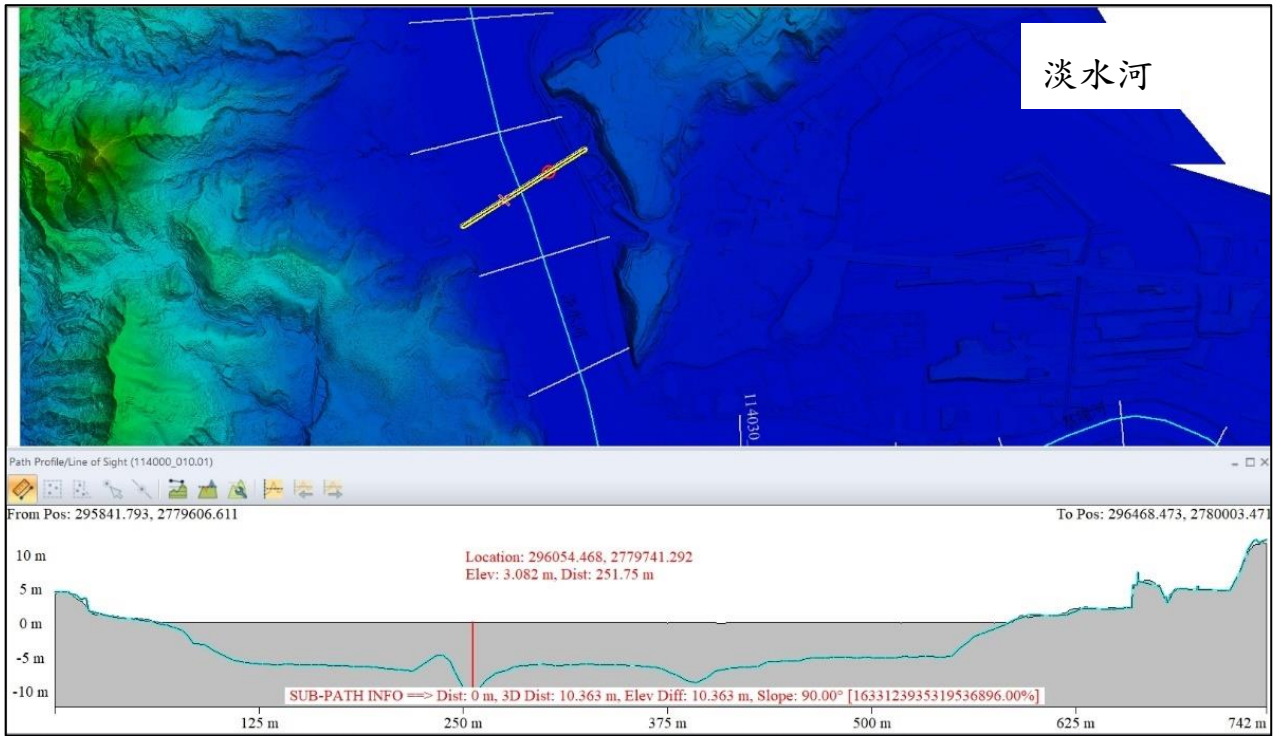
圖 2-53 淡水河断面測量成果與空載光達地形整合比對範例
