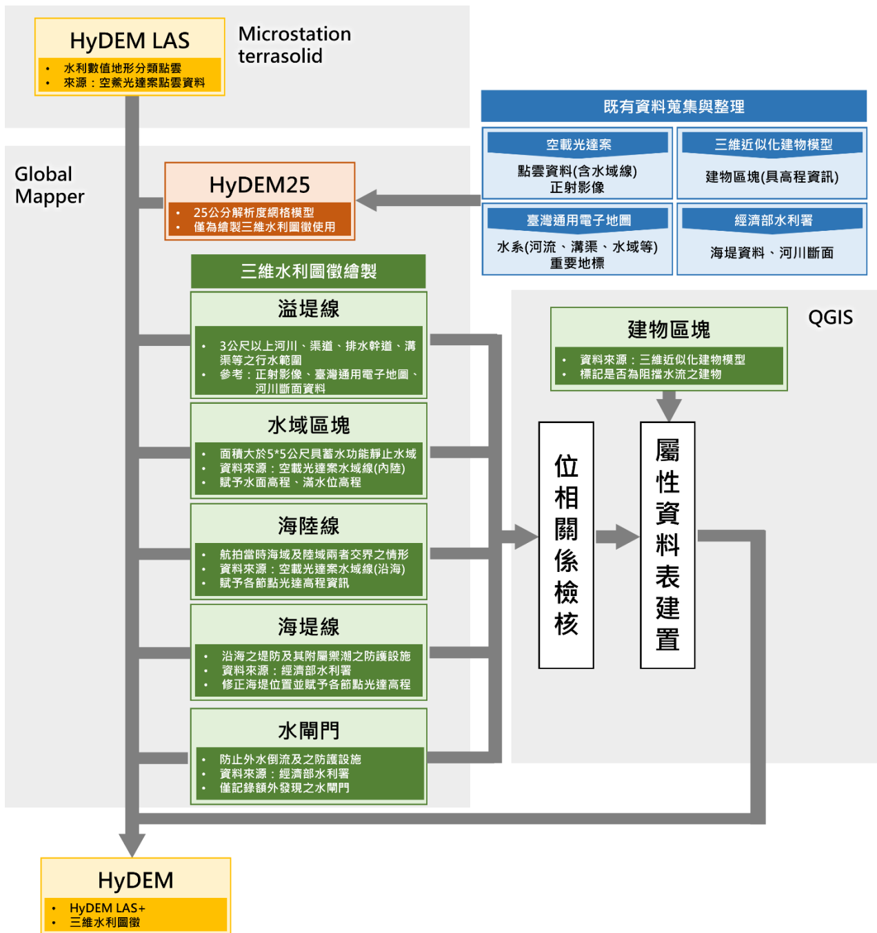
圖 2-15 三維水利圖徵建置作業流程
