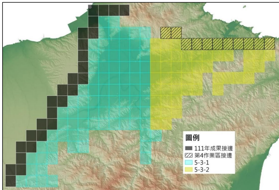
圖 1-1 112 年第 3 業區辦理測製範圍
