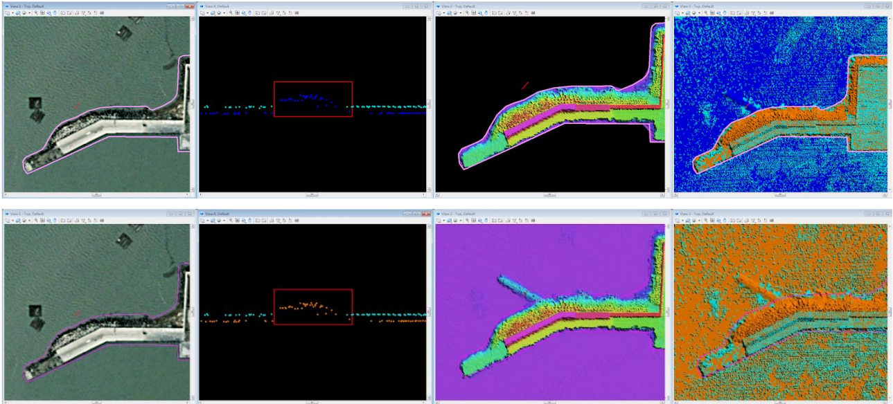
圖 2-14 水線錯誤導致水點分類錯誤(上)與修正點雲分類後成果(下)
