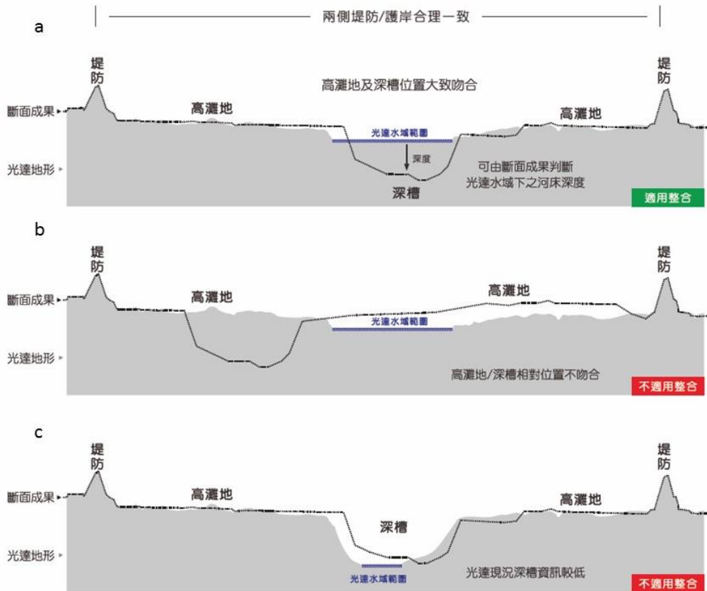
圖 2-50 河川斷面測量成果與空載光達地形比對示意圖
