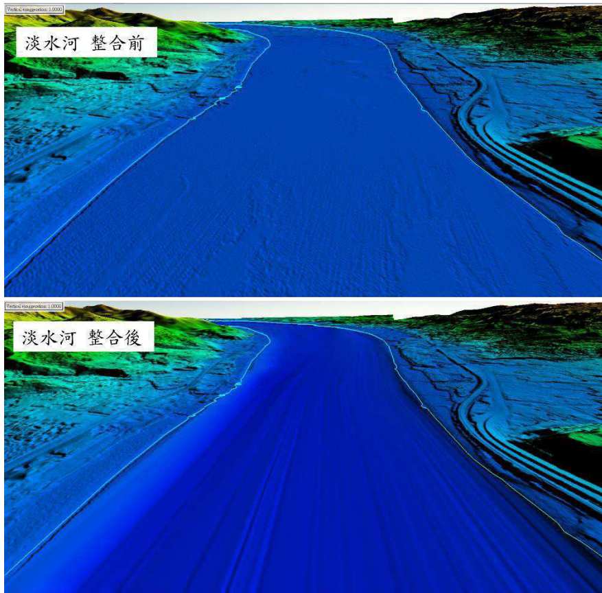
圖 2-58 淡水河河川斷面與 HyDEM 網格整合前後比較示意圖
