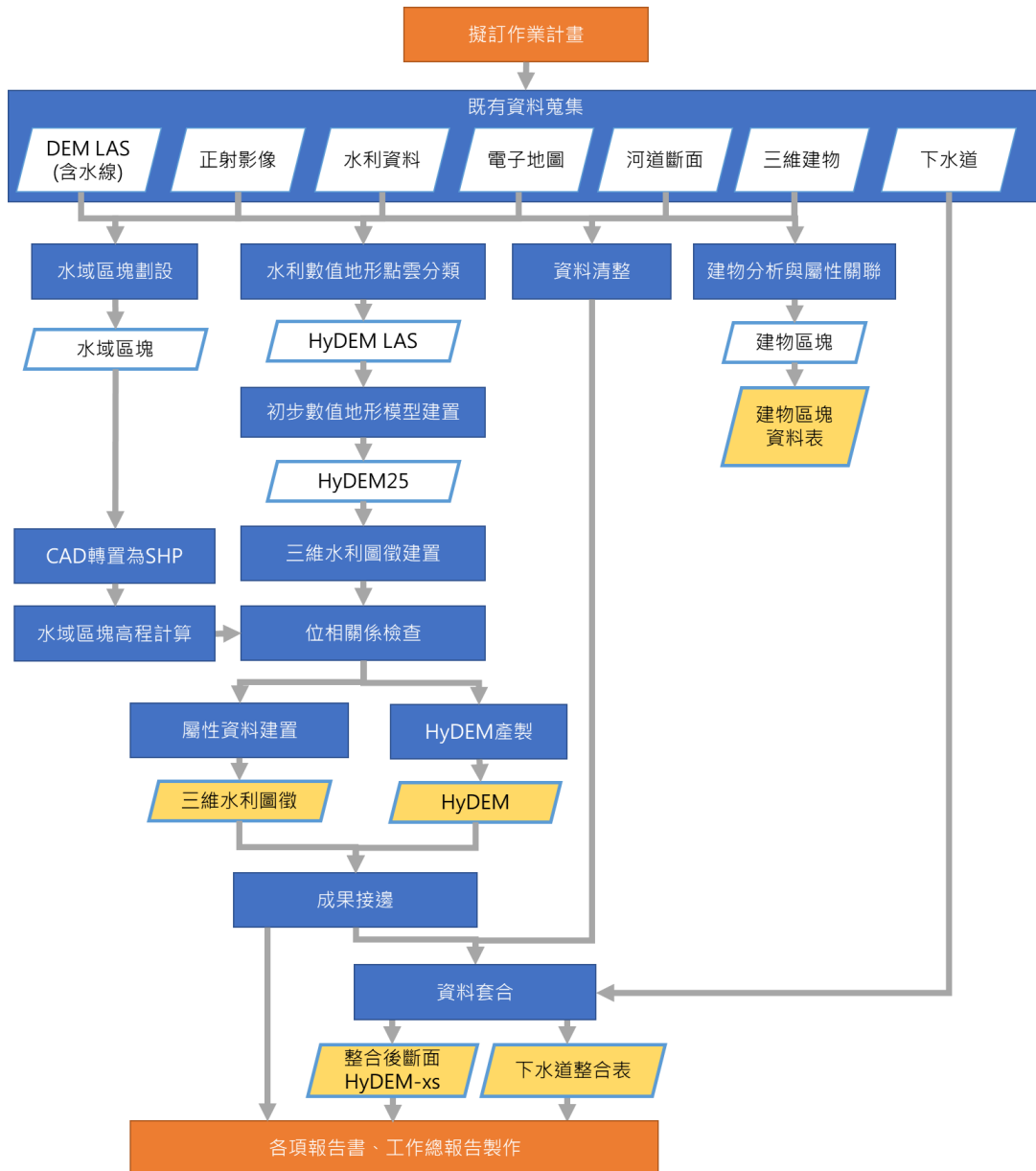
圖 2-1 水利數值地形測製工作流程圖
