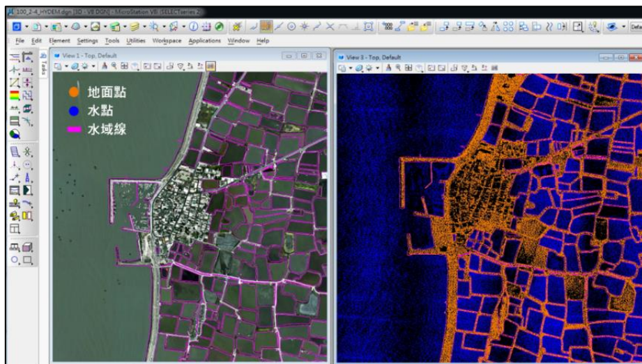
圖 2-3 水域線套疊正射影像與點雲資料
