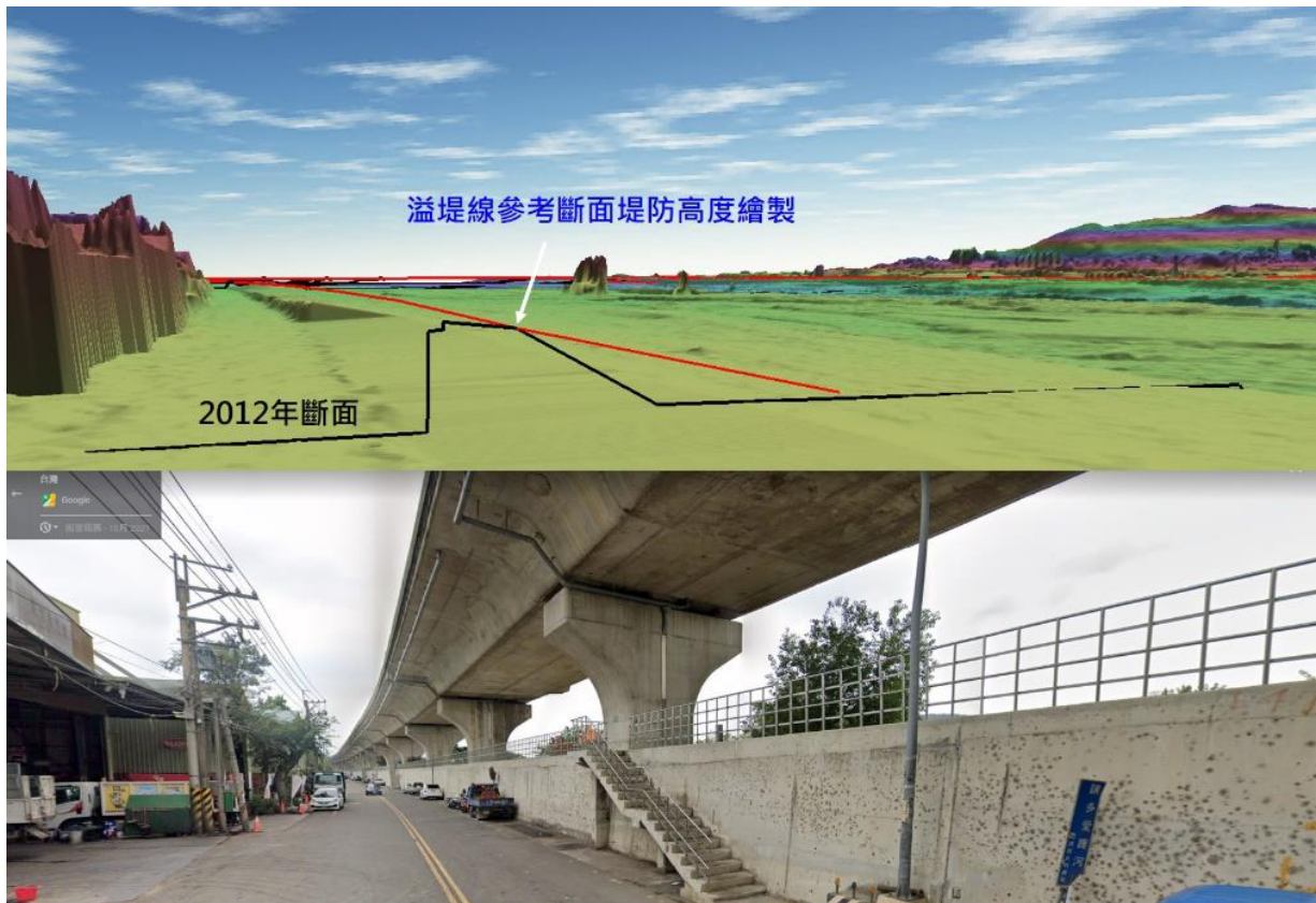
圖 2-24 參照断面資料繪製防洪構造物
