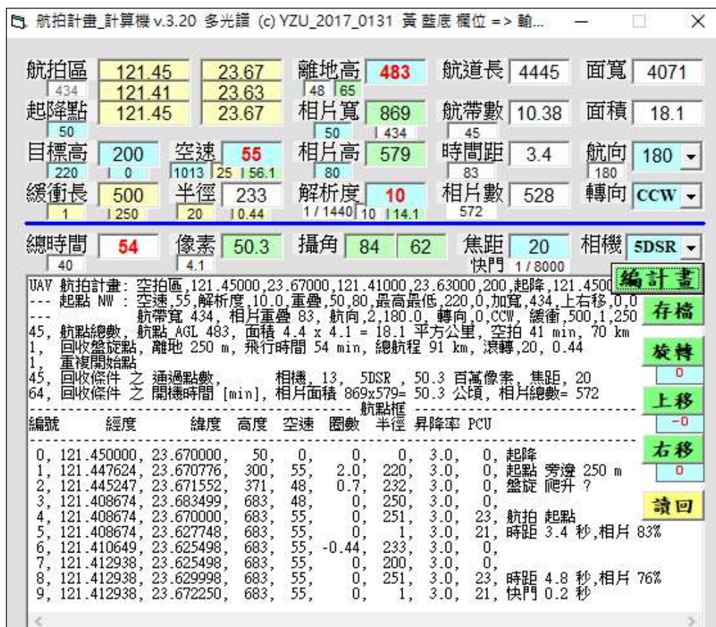
圖 2-7 航拍計算機工具示意圖
