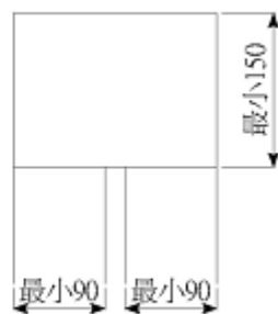
圖 206.3.3.2 坡道迴轉
