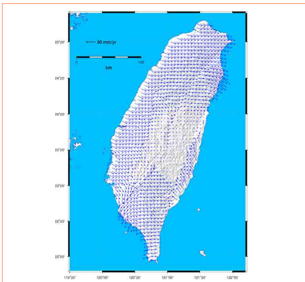
◀ 臺灣地區 TWD97 國家坐標系統變位模式 National coordinate system displacement model under TWD97 for Taiwan
