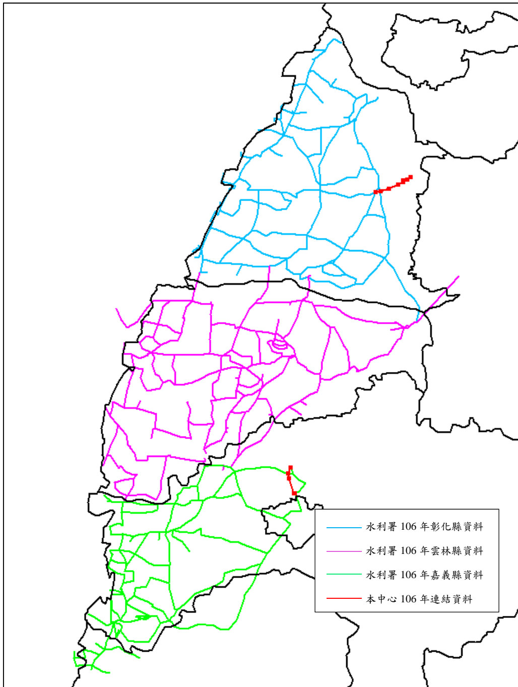
圖 2 106 年度地層下陷區水準網路線圖
