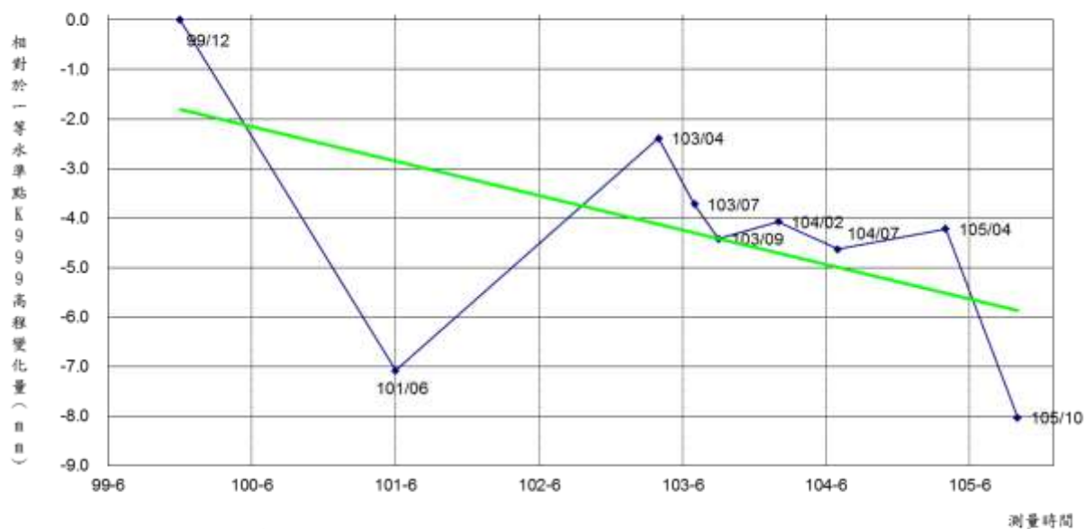
臺灣水準原點高程基準網2041水準點點位穩定性分析圖
