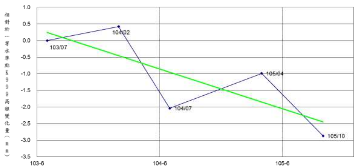
臺灣水準原點高程基準網TG01水準點點位穩定性分析圖
