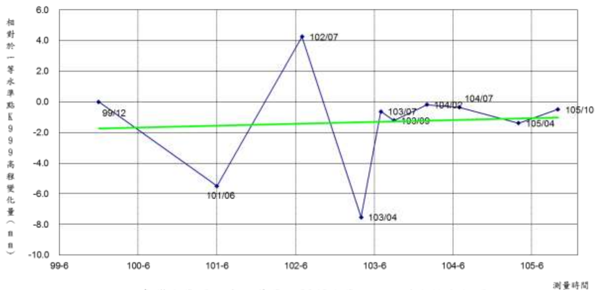
臺灣水準原點高程基準網2043水準點點位穩定性分析圖
