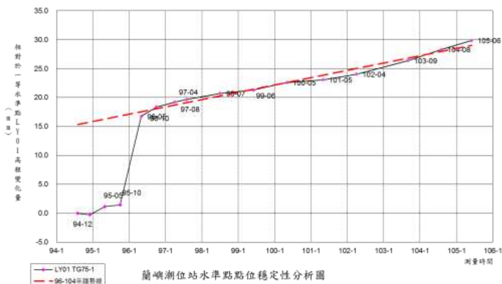
圖 5-13 蘭嶼潮位站水準點 TG75-1 相對一等水準點 LY01 之高程差變化圖
