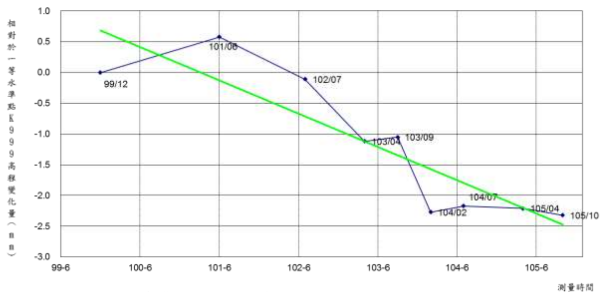
臺灣水準原點高程基準網K011水準點點位穩定性分析圖
