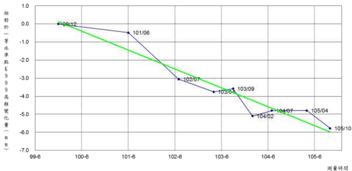
臺灣水準原點高程基準網2040水準點點位穩定性分析圖
