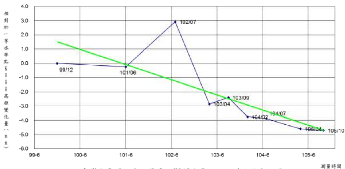
臺灣水準原點高程基準網K013水準點點位穩定性分析圖
