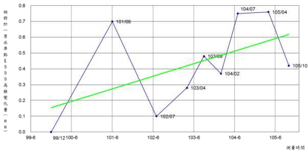
臺灣水準原點高程基準網2039水準點點位穩定性分析圖
