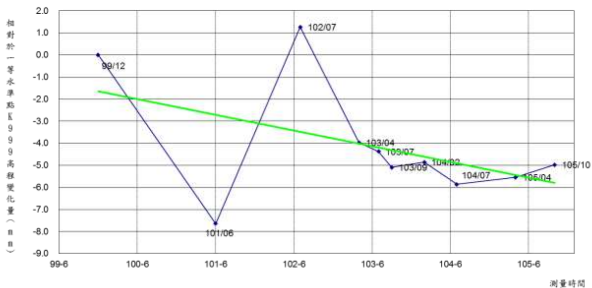
臺灣水準原點高程基準網2042水準點點位穩定性分析圖
