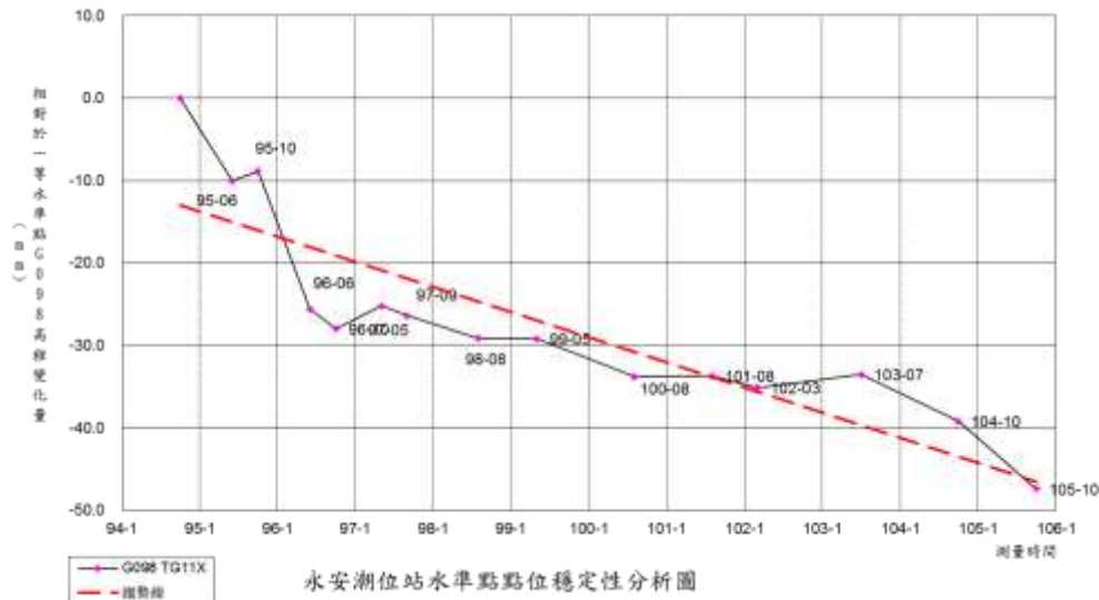
圖 5-7 永安潮位站水準點 TG11X 相對一等水準點 G098 之高程差變化圖
