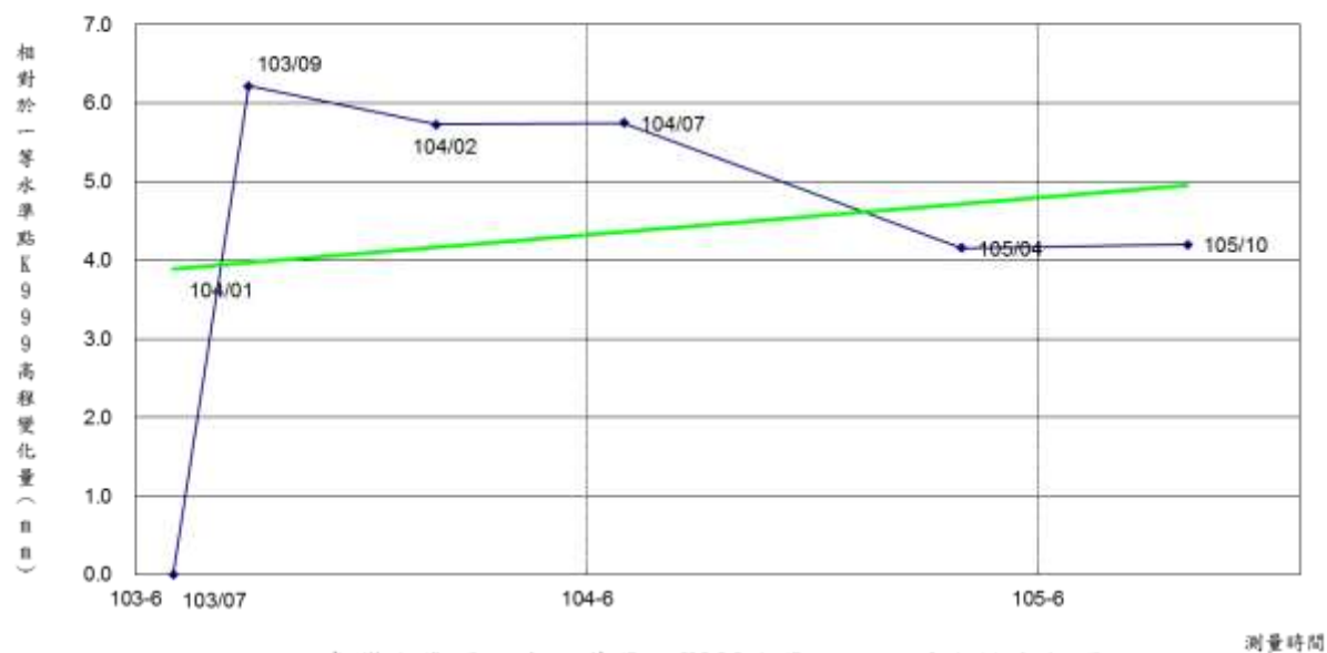
臺灣水準原點高程基準網K996水準點點位穩定性分析圖
