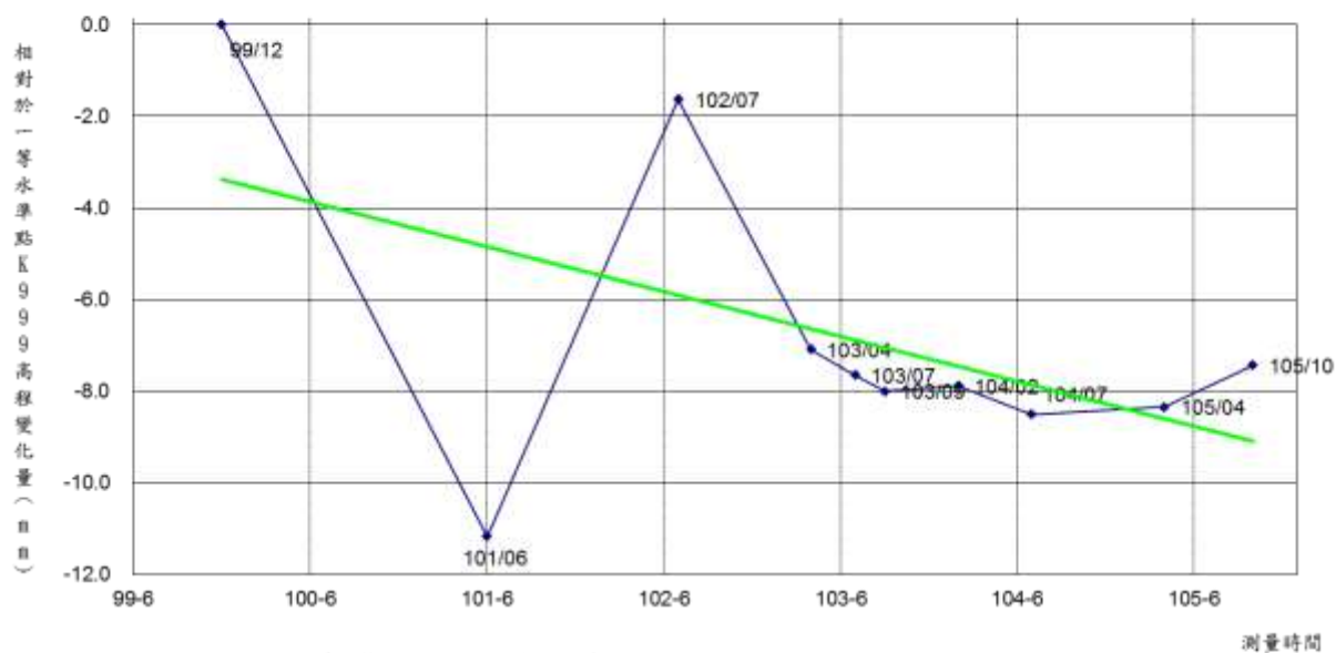
臺灣水準原點高程基準網K014水準點點位穩定性分析圖
