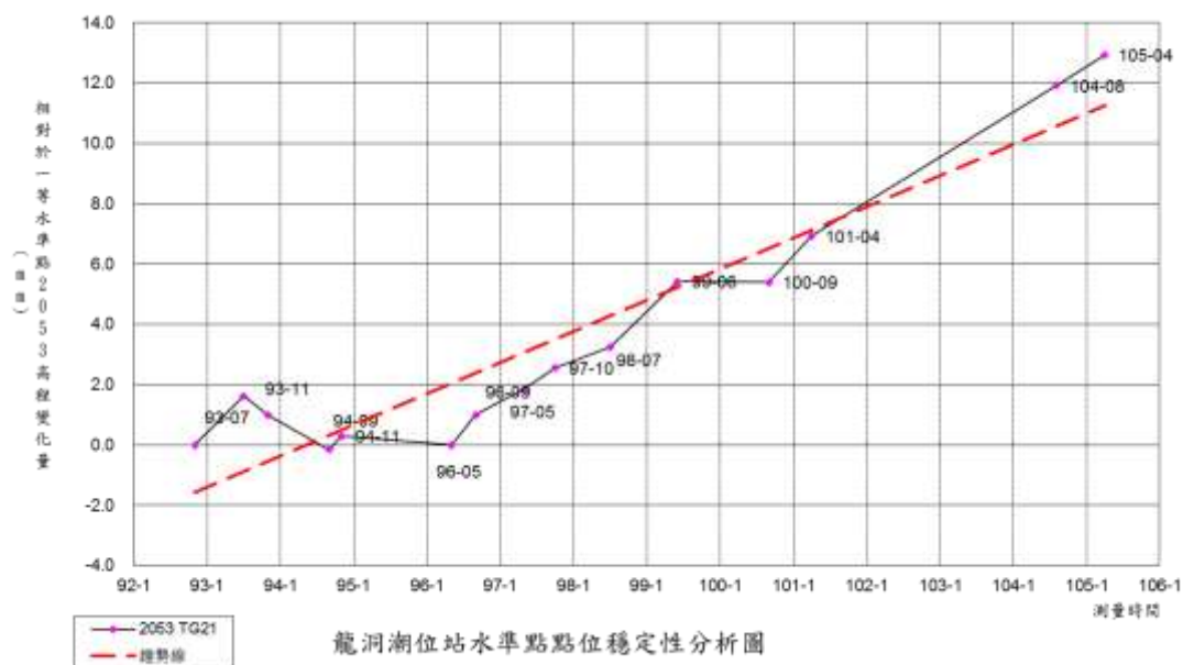
圖 5-10 龍洞潮位站水準點 TG21 相對一等水準點 2053 之高程差變化圖
