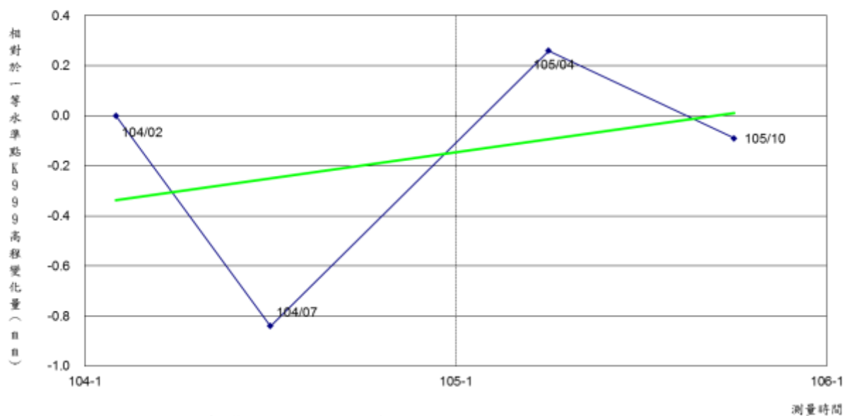
臺灣水準原點高程基準網TG997水準點點位穩定性分析圖
