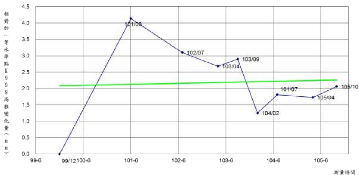
臺灣水準原點高程基準網K012水準點點位穩定性分析圖
