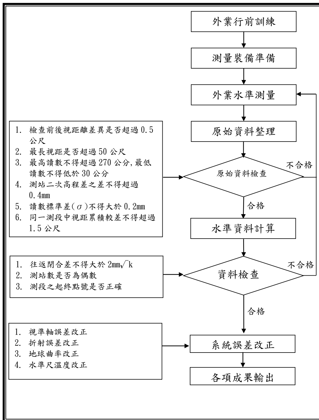
圖 2-2 高程基準檢測作業流程圖
