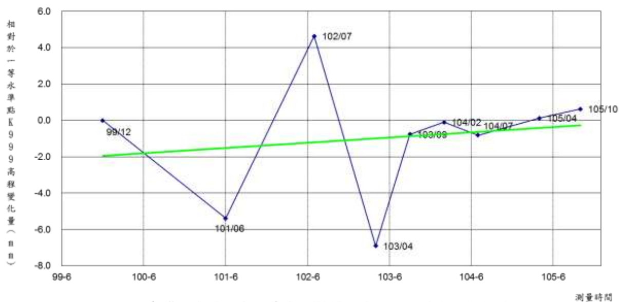
臺灣水準原點高程基準網K015水準點點位穩定性分析圖
