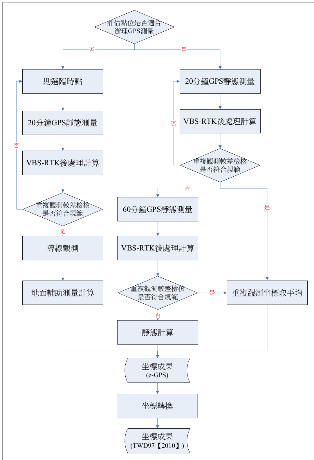
圖 2 點位坐標計算流程圖
