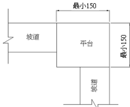
圖 305.3.3.1 坡道 90° 轉彎
