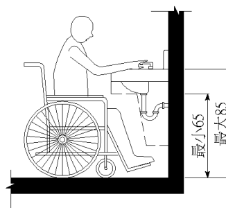
圖 3-1.2 輪椅乘坐者可及範圍
