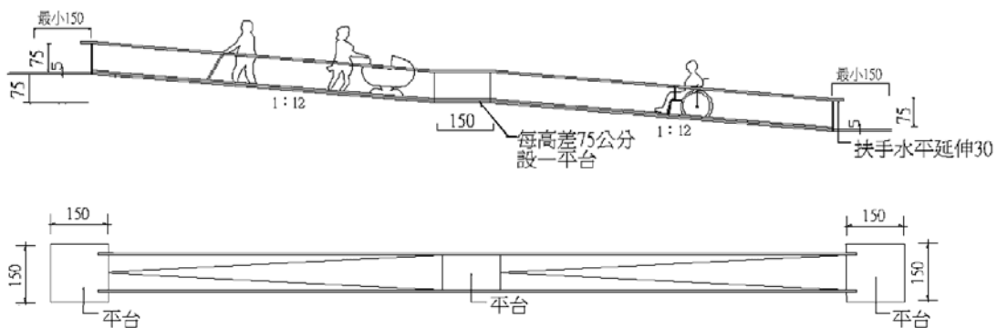
圖 3-1.1 輪椅通行需要之具體尺寸
