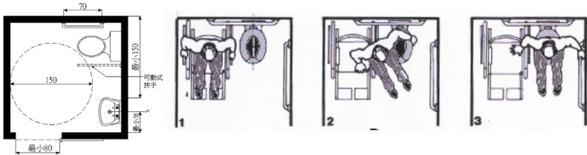
圖 5-2.2 馬桶兩側設扶手之移位方式
