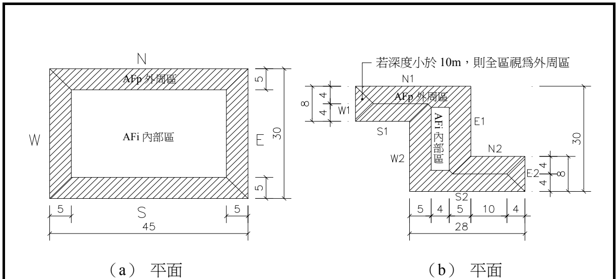
圖 2 建築物外周區範圍（外牆中心線起算深度 5m 內）
