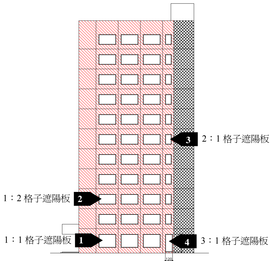
東向立面圖
