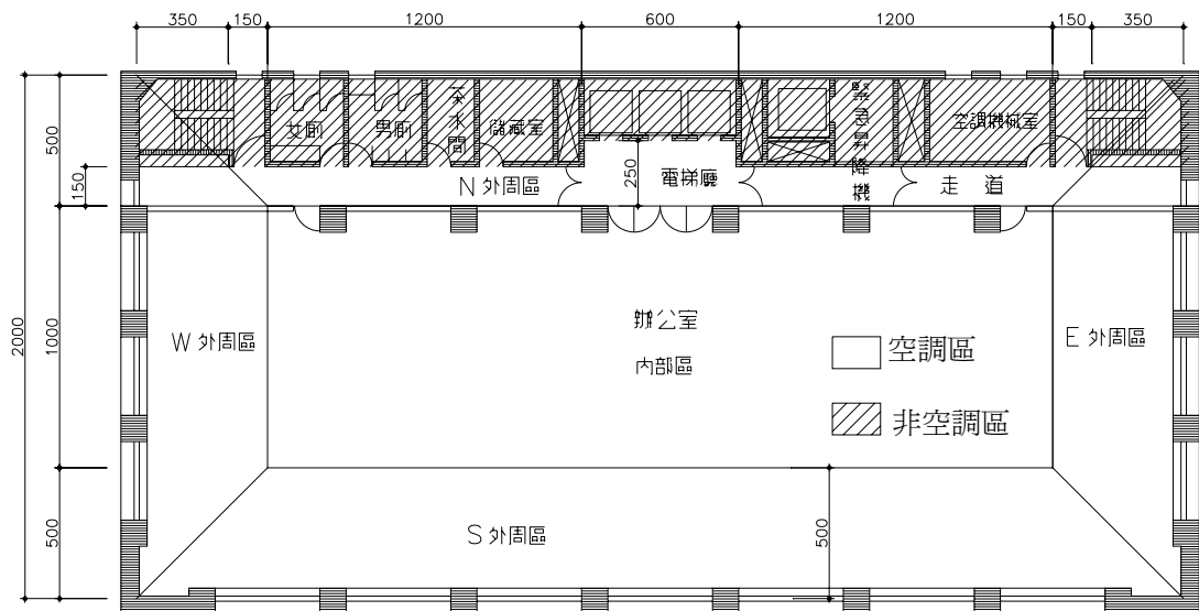
圖 A-3 標準層平面圖
