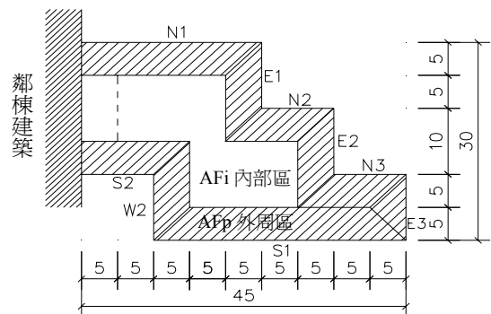
(平面)
