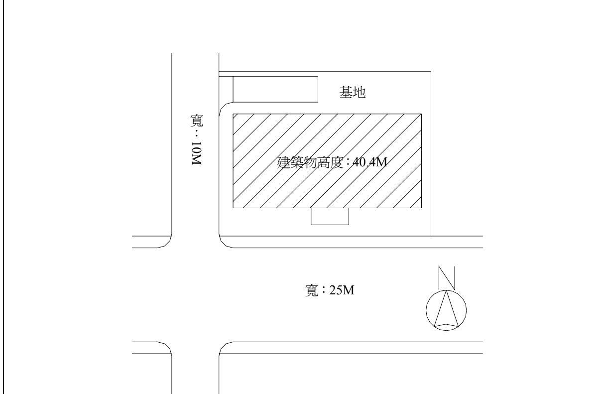
圖 A-1、大樓配置圖
