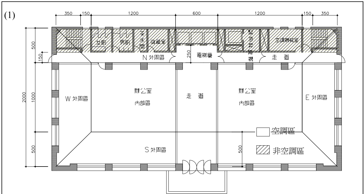
圖 A-2 地面層平面圖
