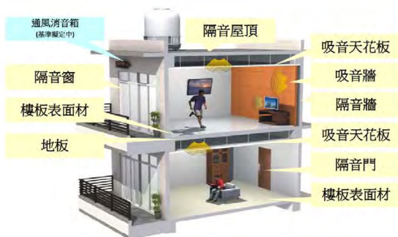
圖 7-14 高性能防音綠建材評定範圍
