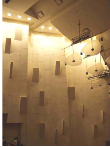
圖 7-4 多樣聲學建材組成之演藝空間
