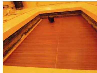
(b) 輕量衝擊源樓板衝擊音測試
