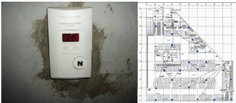
圖2-4.1 一氧化碳偵測器設置實例
