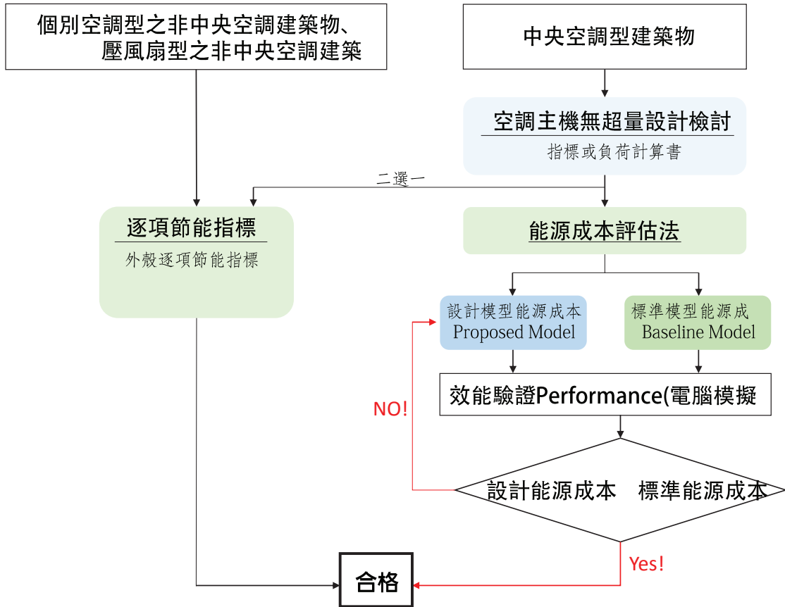
圖2-2.2 EEWH-GF日常節能評估步驟
