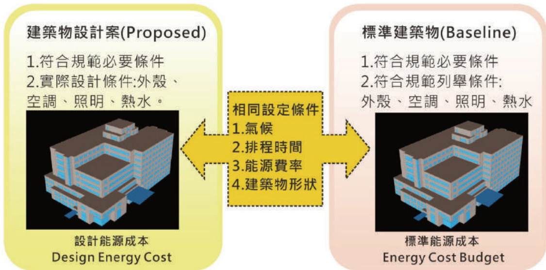
圖2-2.3 EEWH-GF 廠房能源成本分析概念
