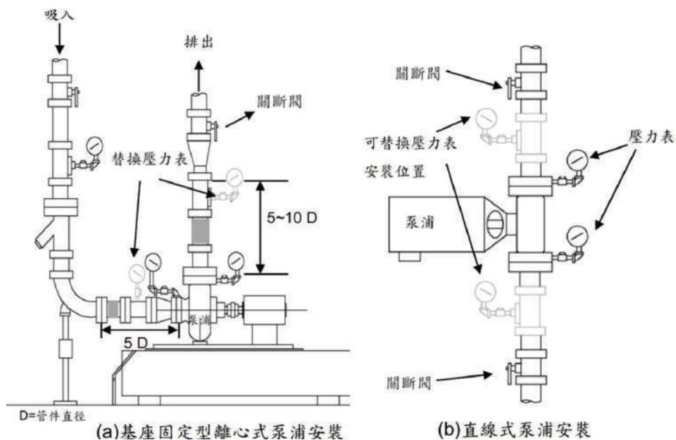
圖2.1 泵的進出口安裝考克壓力表組安裝位置示意圖
