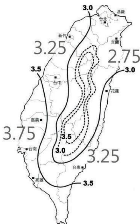
圖2-2.4 太陽光電發電量基準值kWh/(m 2 .day)
