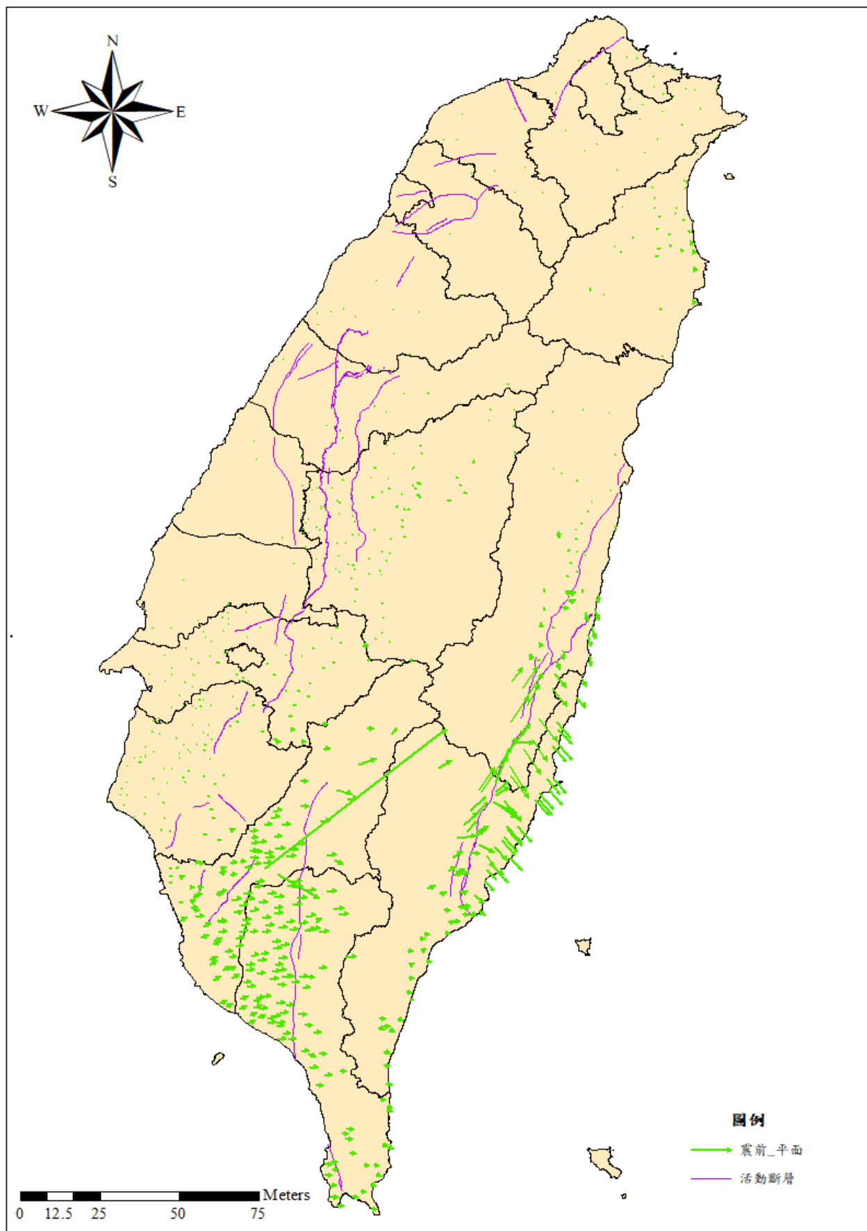
圖 1A 震前平面分量較差向量示意圖
