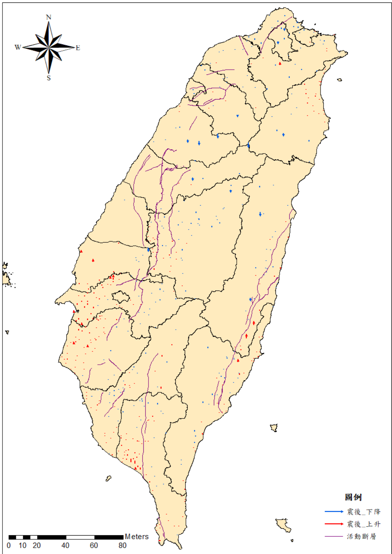
圖 2B 震後高程分量較差向量示意圖
