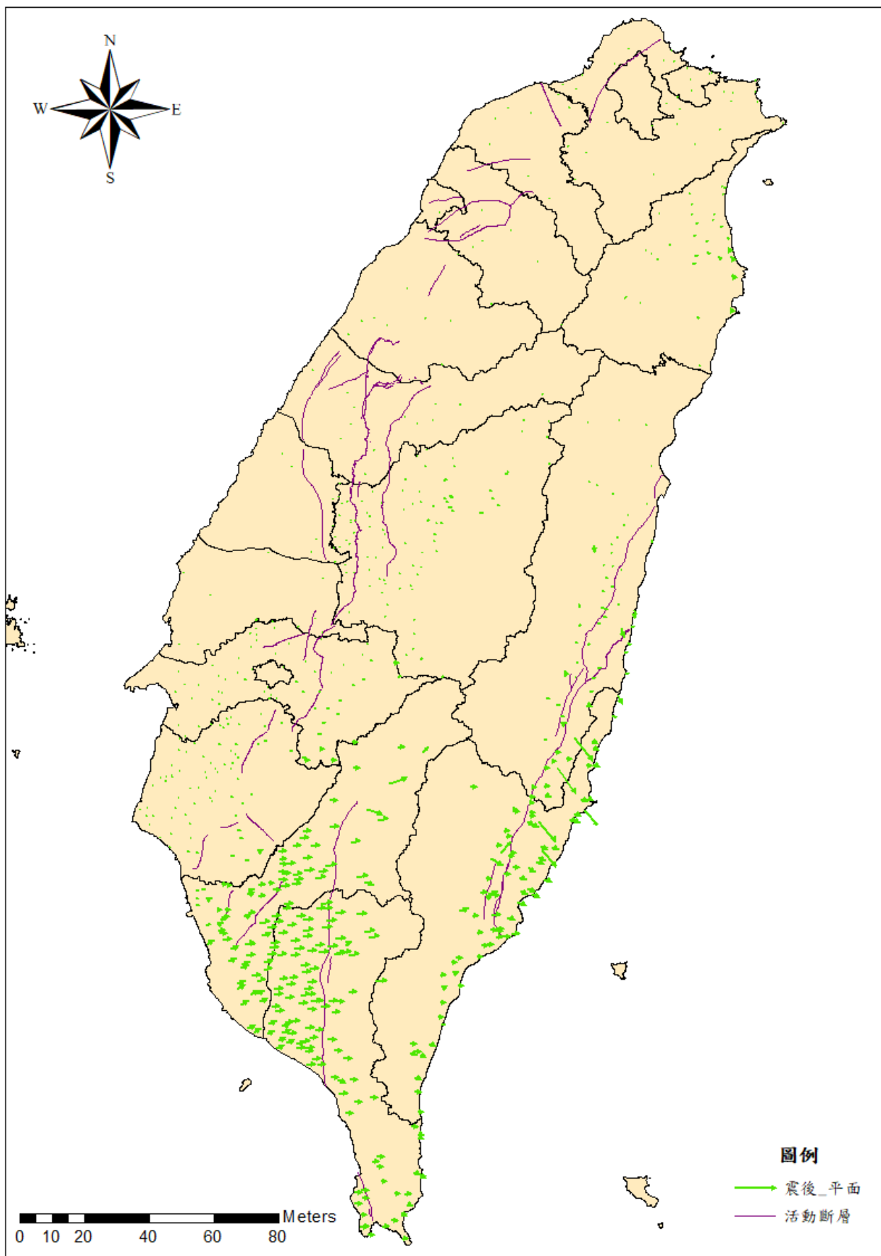
圖 2A 震後平面分量較差向量示意圖
