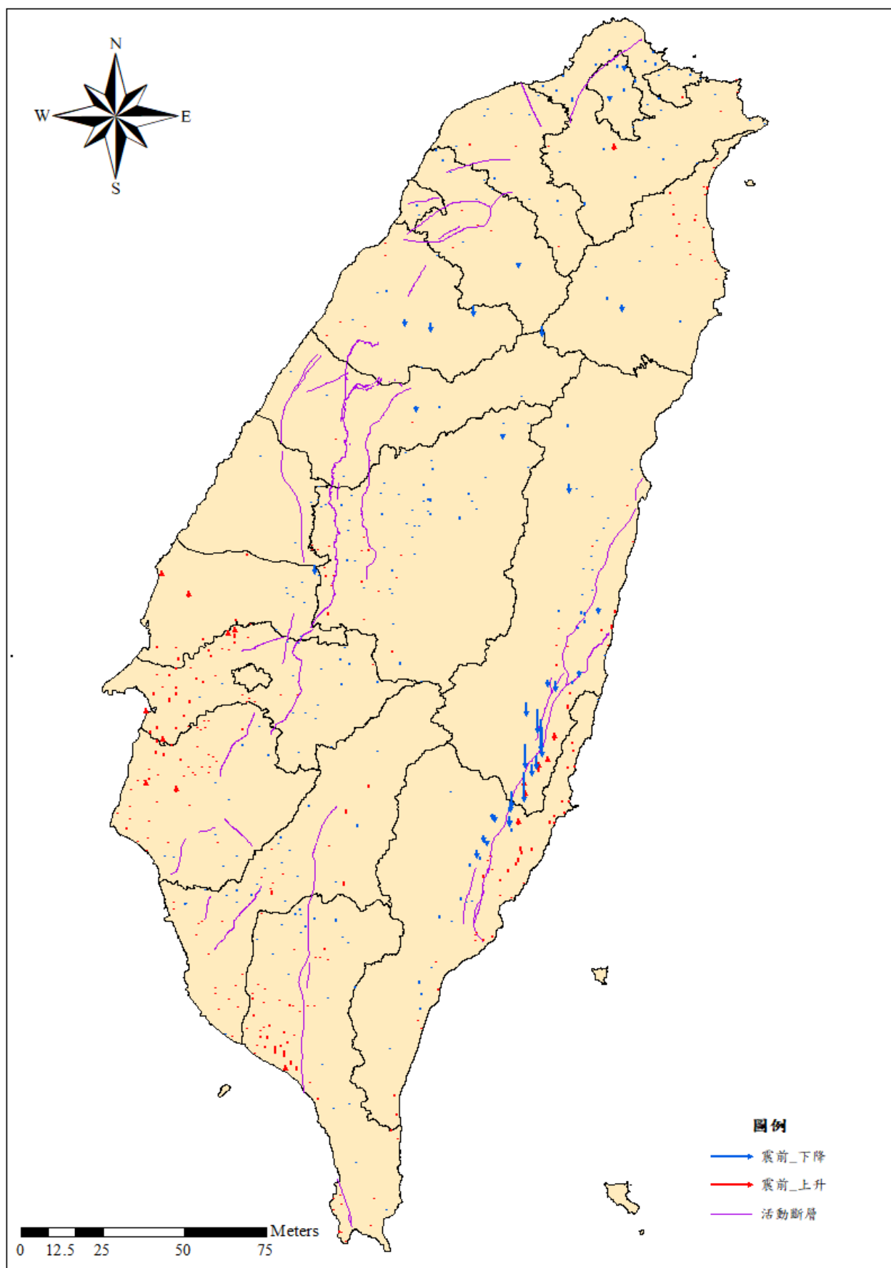
圖 1B 震前高程分量較差向量示意圖
