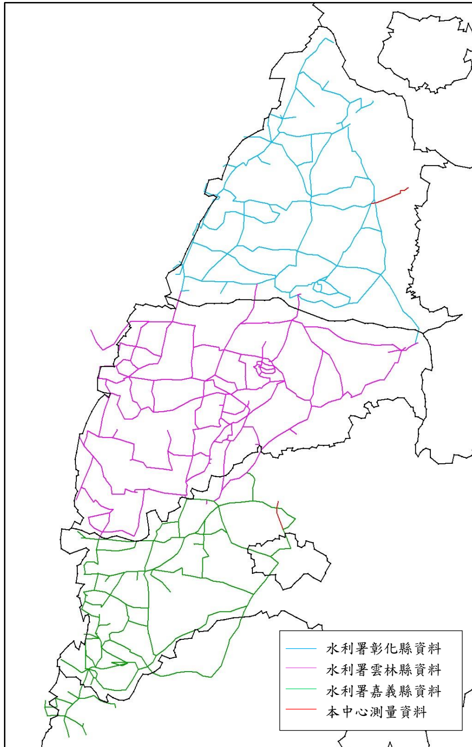
圖 2 109 年度地層下陷區水準網路線圖
