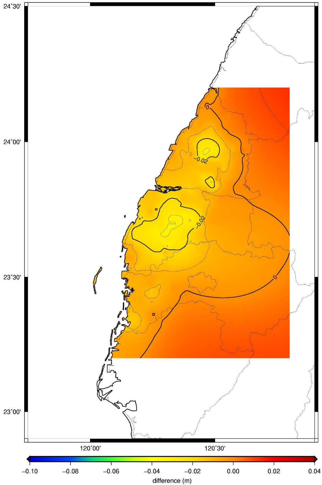
圖 4 108 年至 109 年地層下陷區正高變化情形
