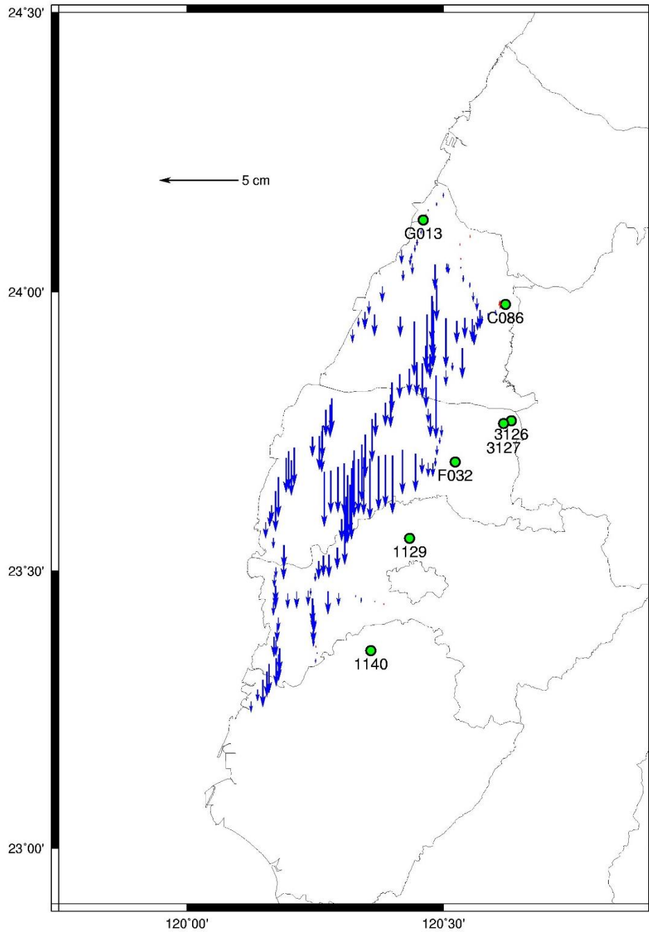
圖 3 109 年與 108 年計算成果較差圖
